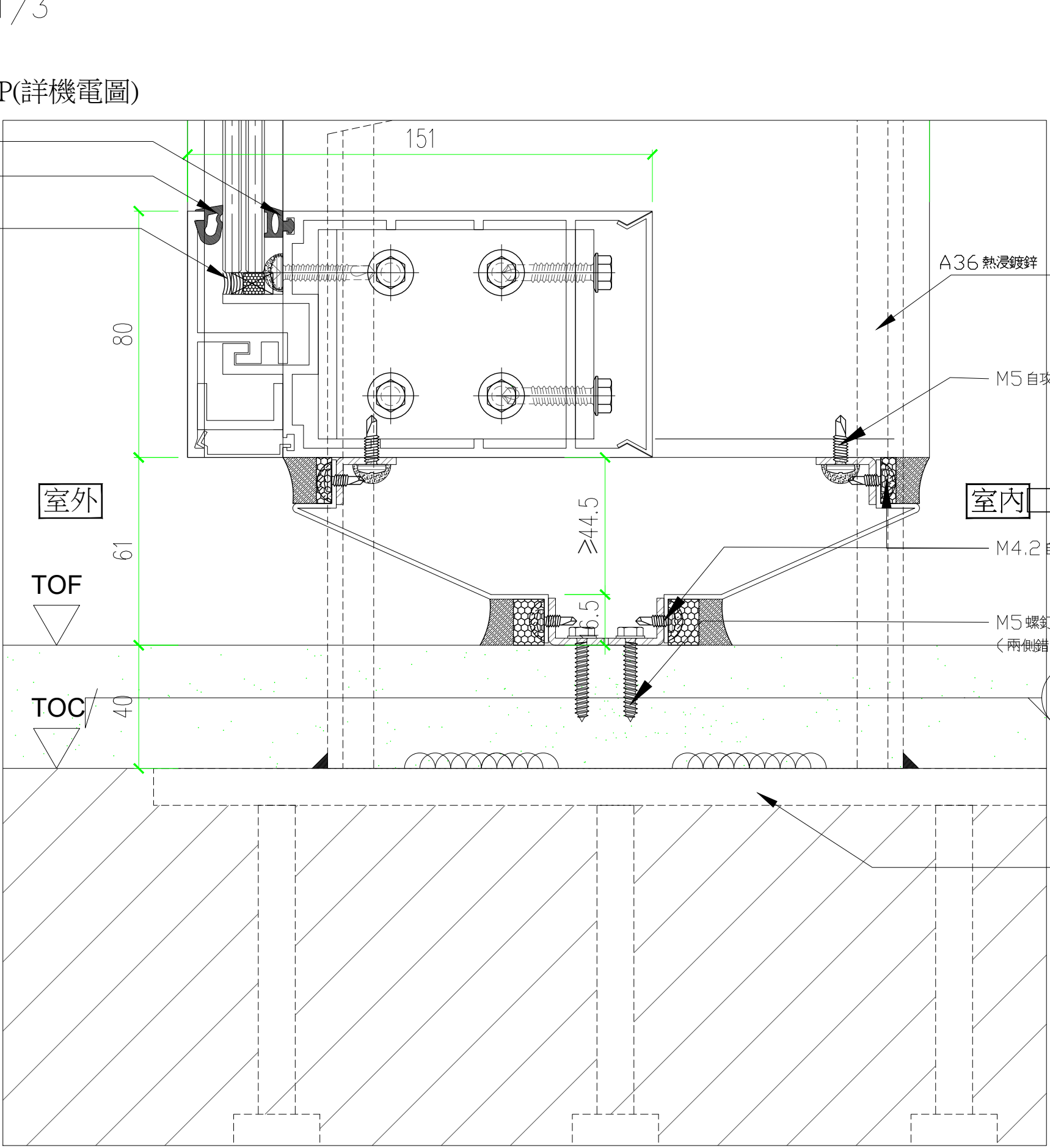
剖面大樣 1/3
