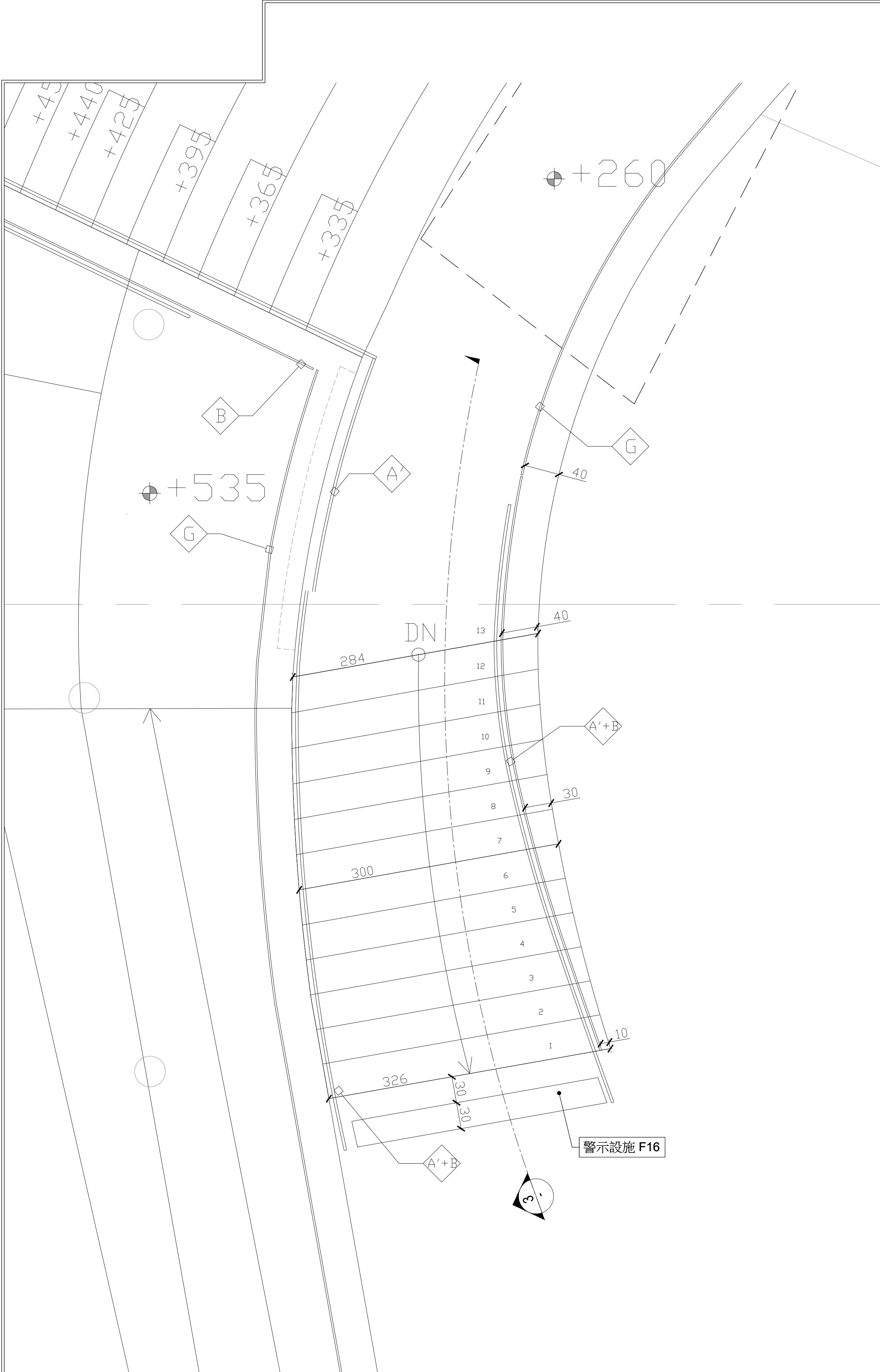
① 樓梯 N 平面圖
