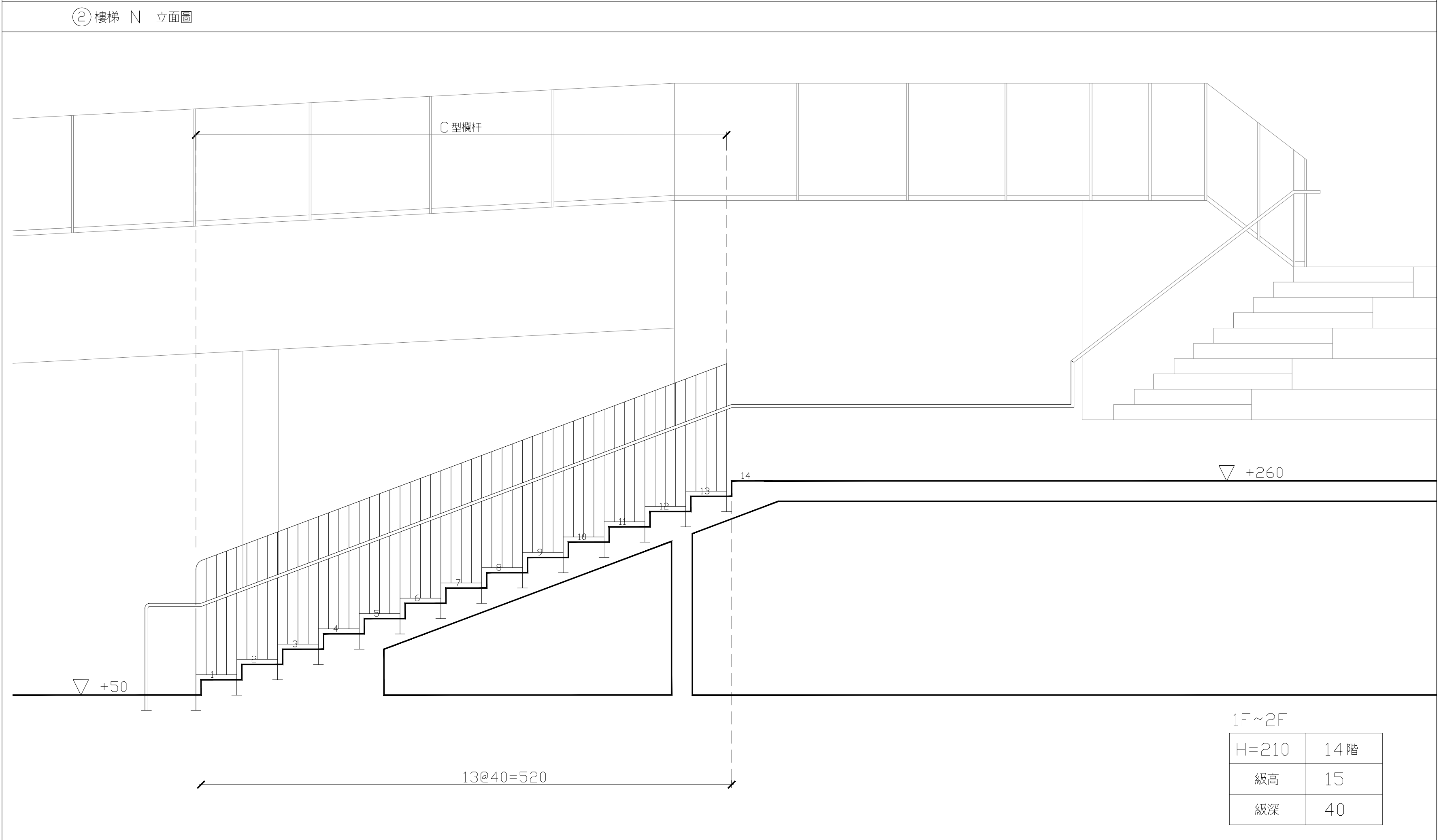
② 樓梯 N 立面圖
