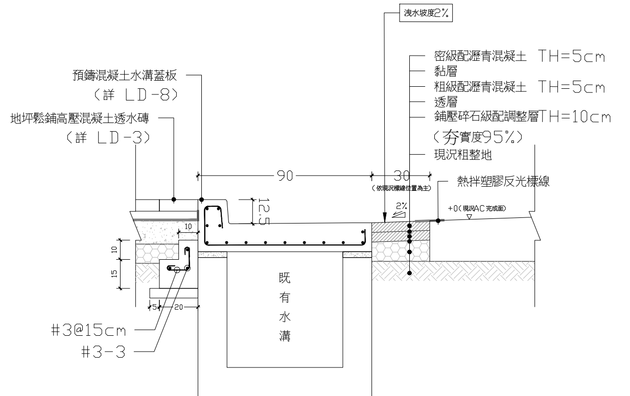
③ 熱拌瀝青混凝土—預鑄混凝土水溝蓋板 連接斷面詳圖
