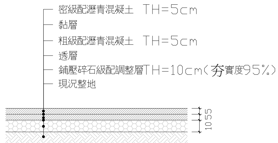
② 熱拌瀝青混凝土 斷面詳圖
