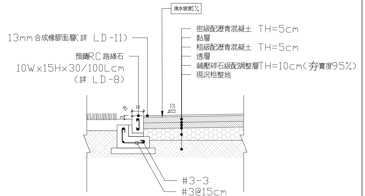
④ 熱拌瀝青混凝土—預鑄RC路緣石 連接斷面詳圖
