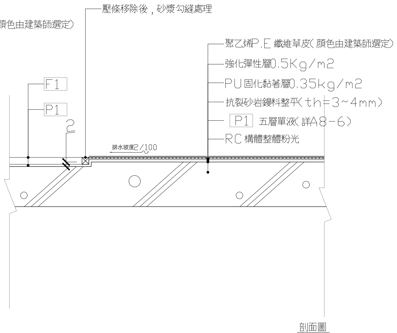
剖面圖
