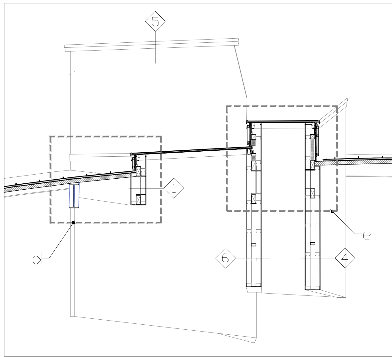
B 型天窗 剖面2 - 細部索引圖
