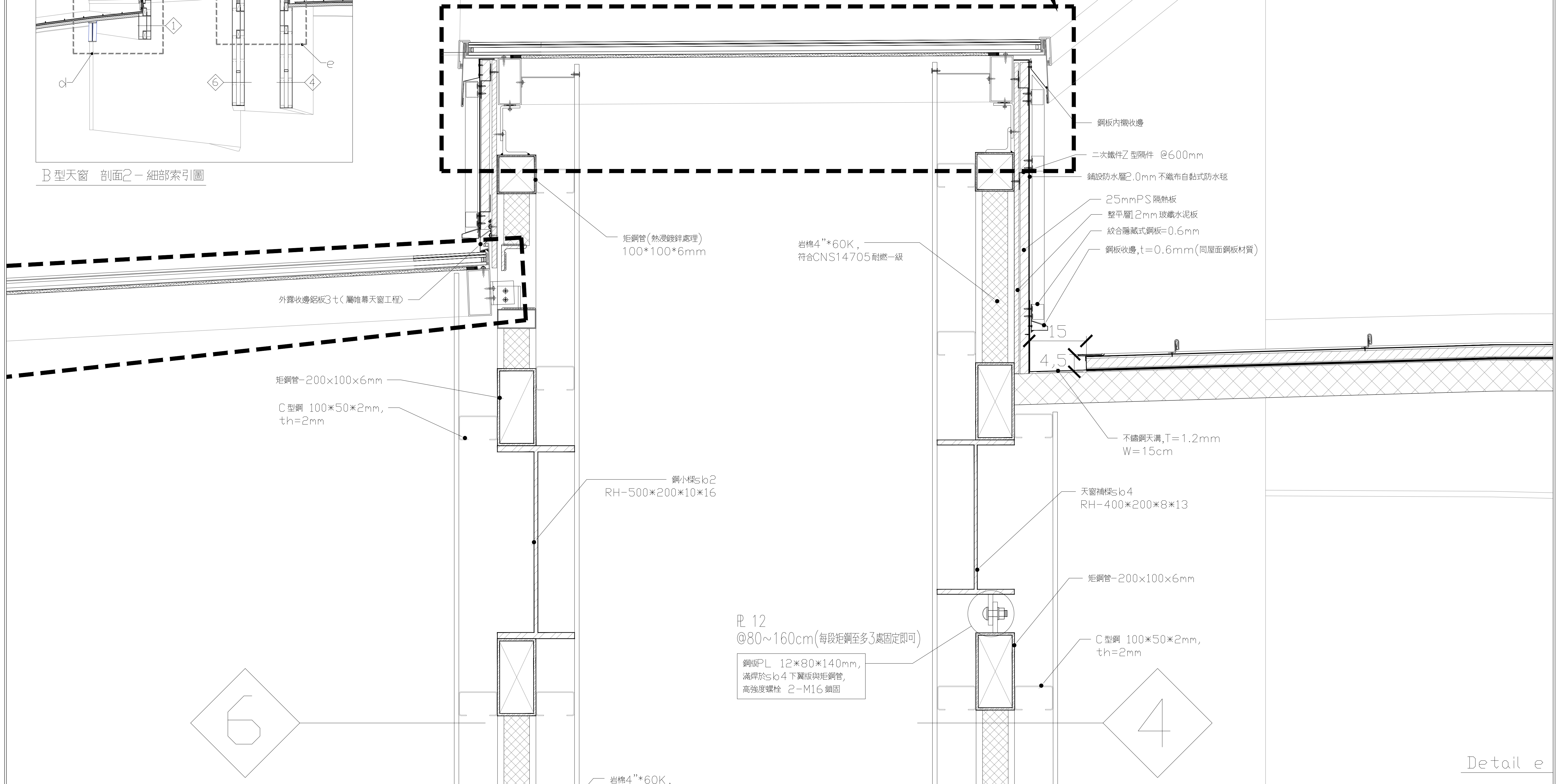
B 型天窗 剖面2 - 細部詳圖
