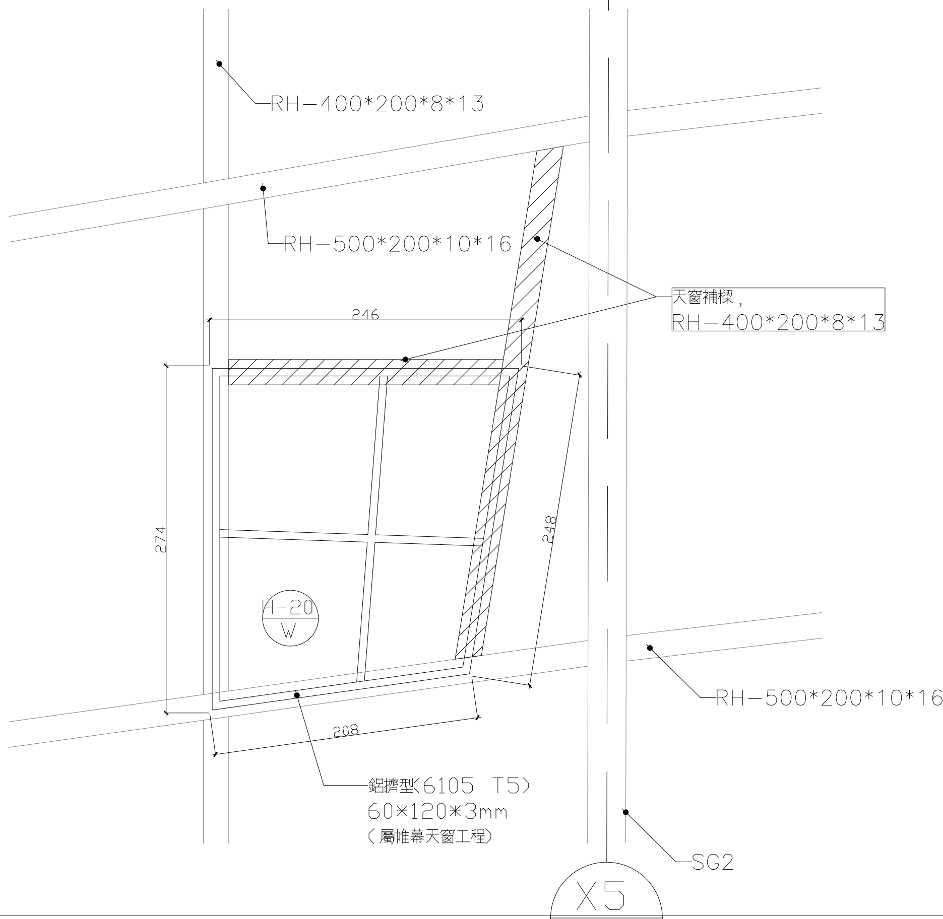
A 型天窗-1
