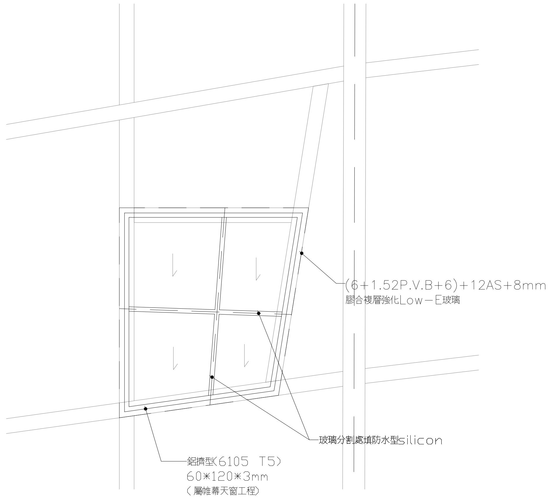
玻璃平面圖
