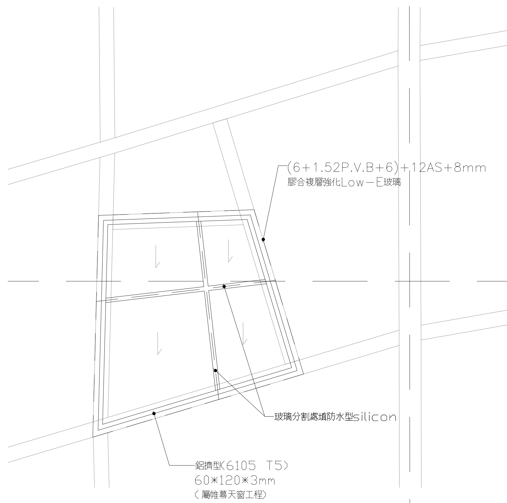
玻璃平面圖
