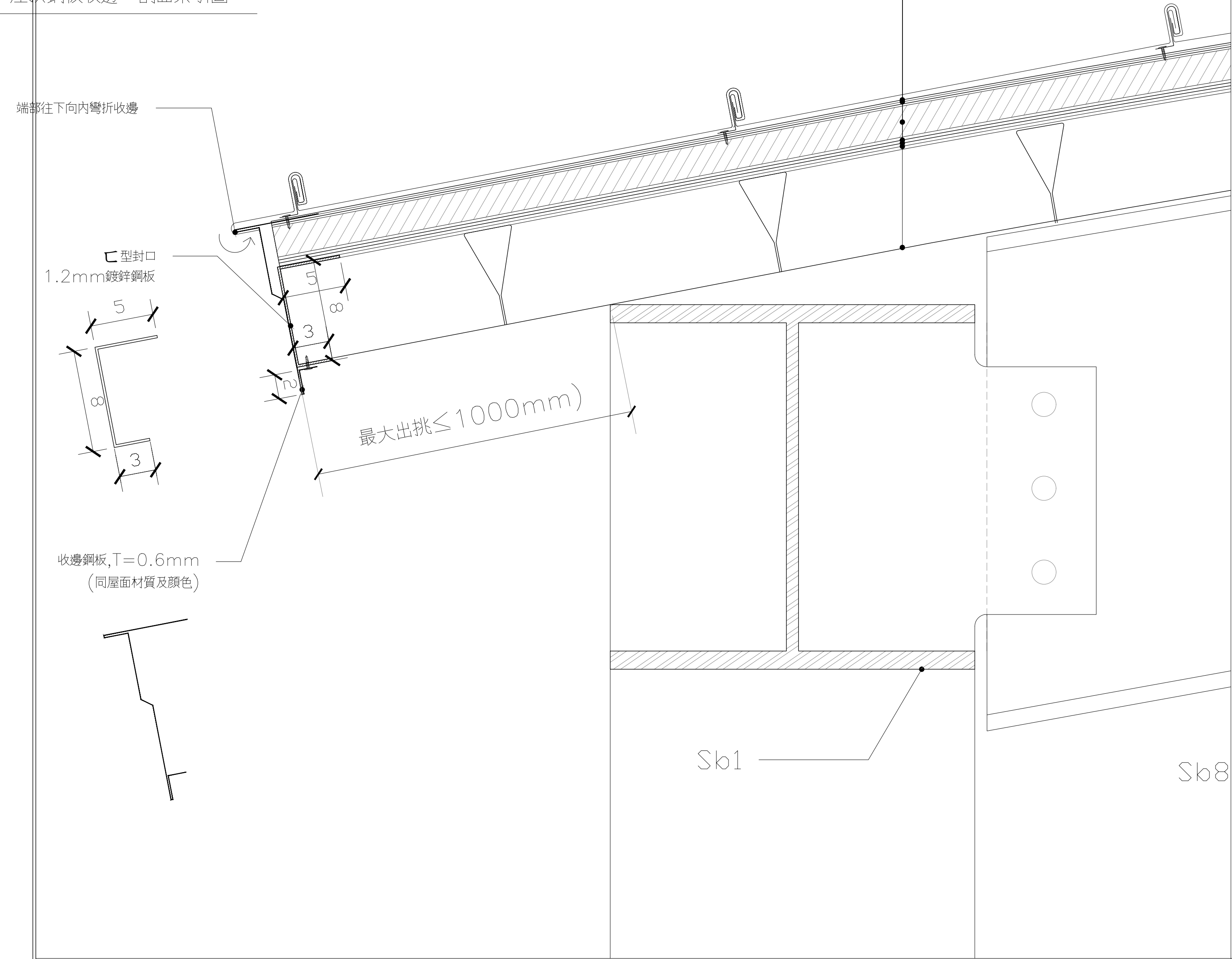
屋緣收邊 C-C' 剖面詳圖
