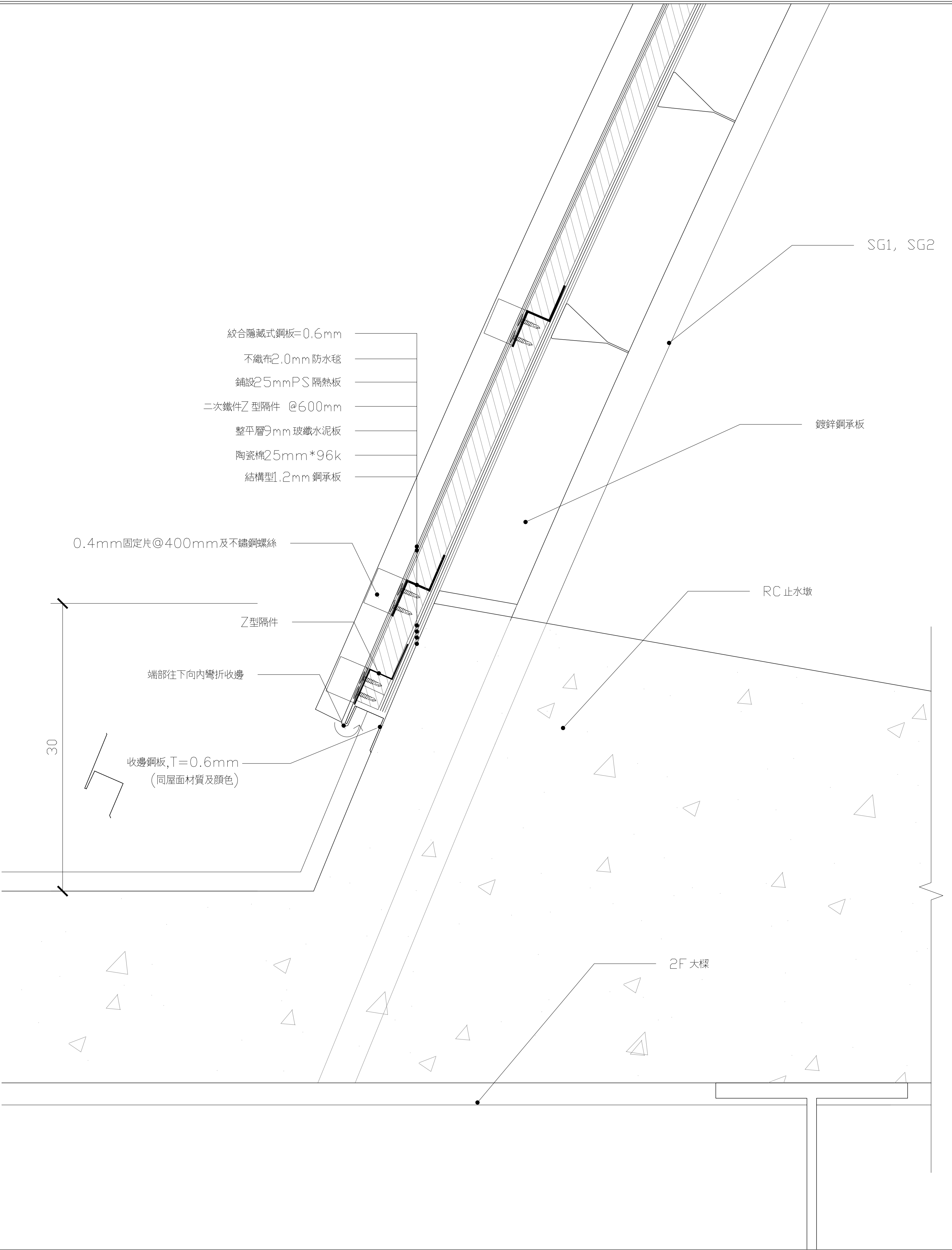
牆面收邊剖面詳圖
