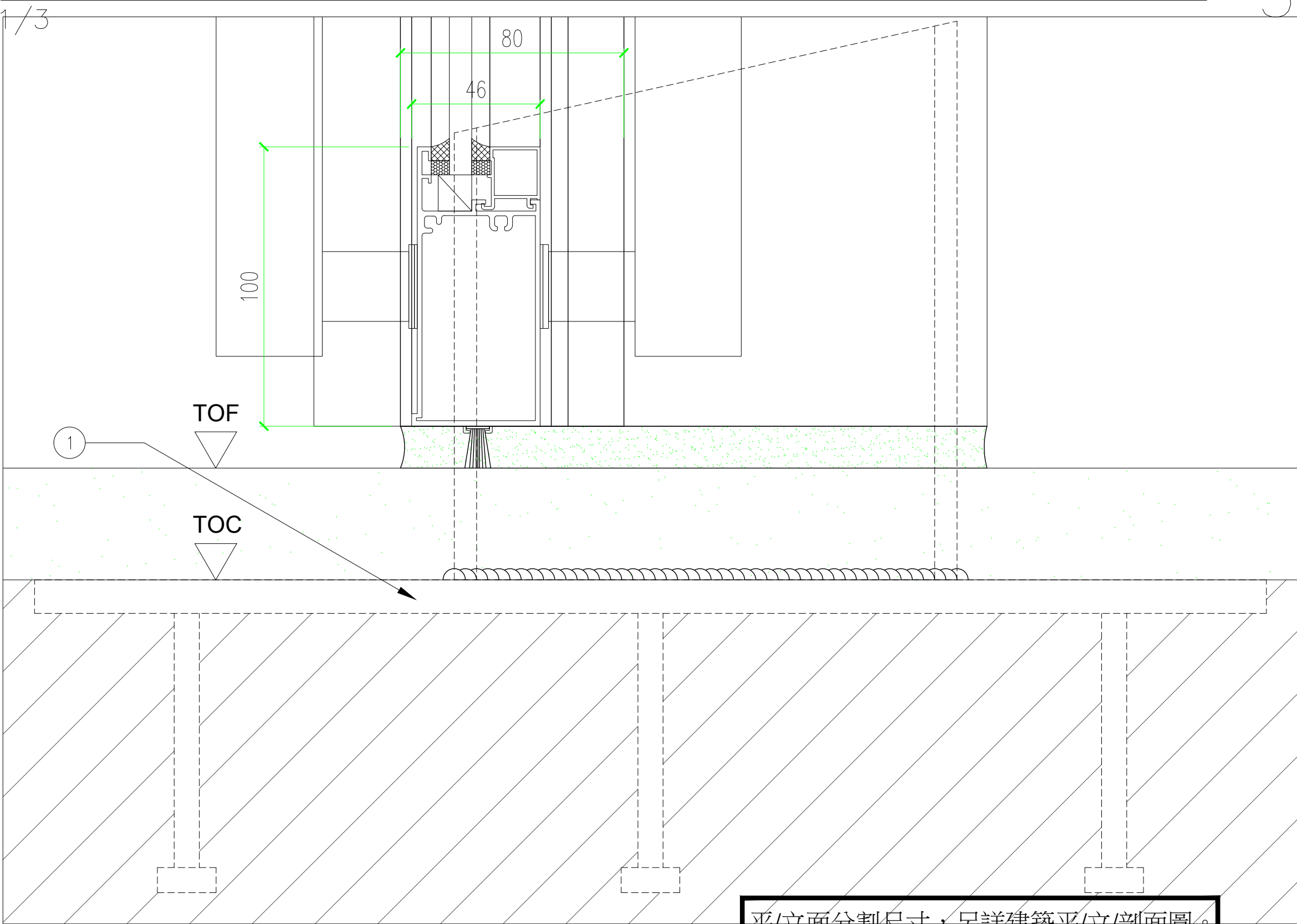
剖面大樣
