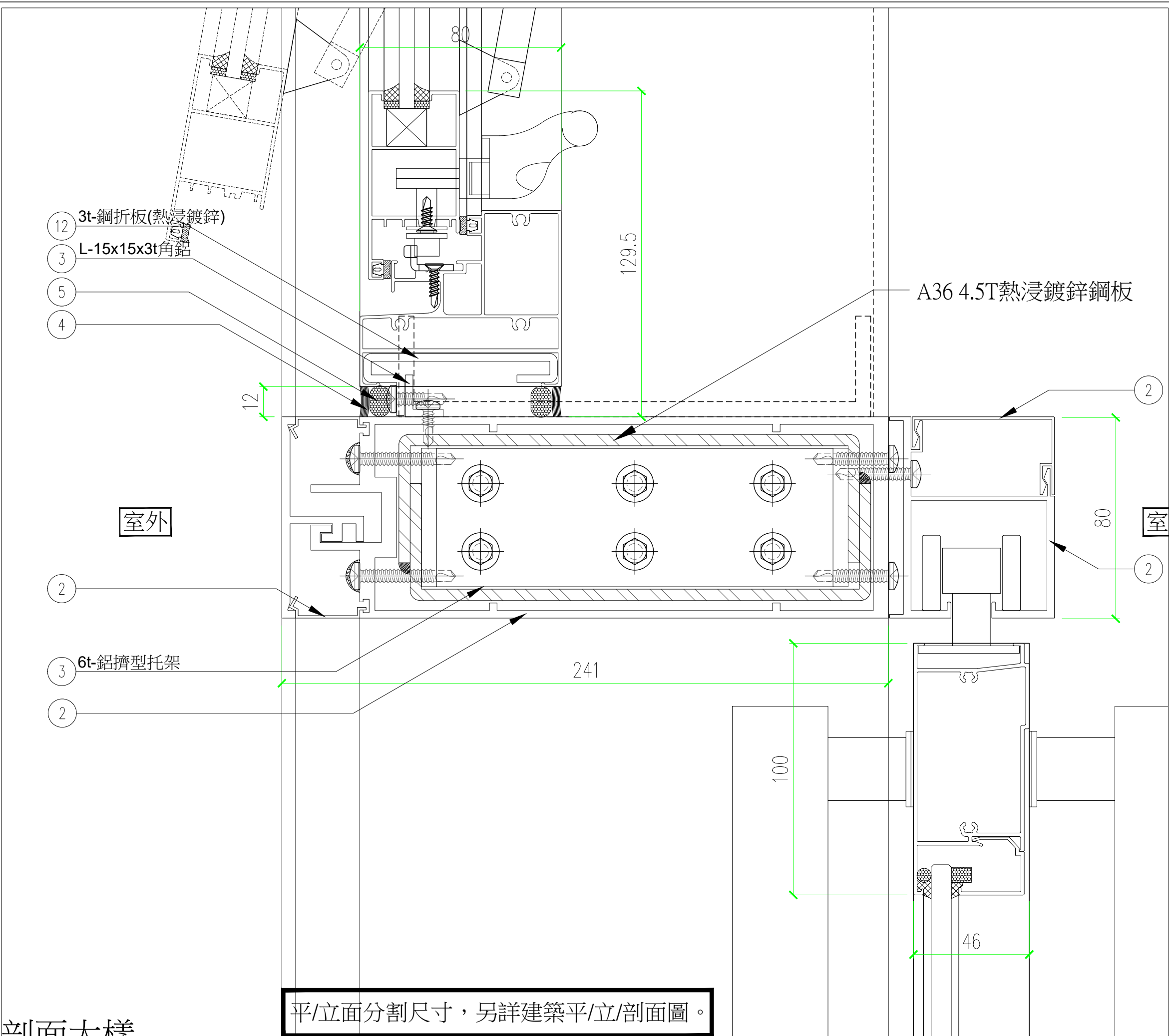
剖面大樣
