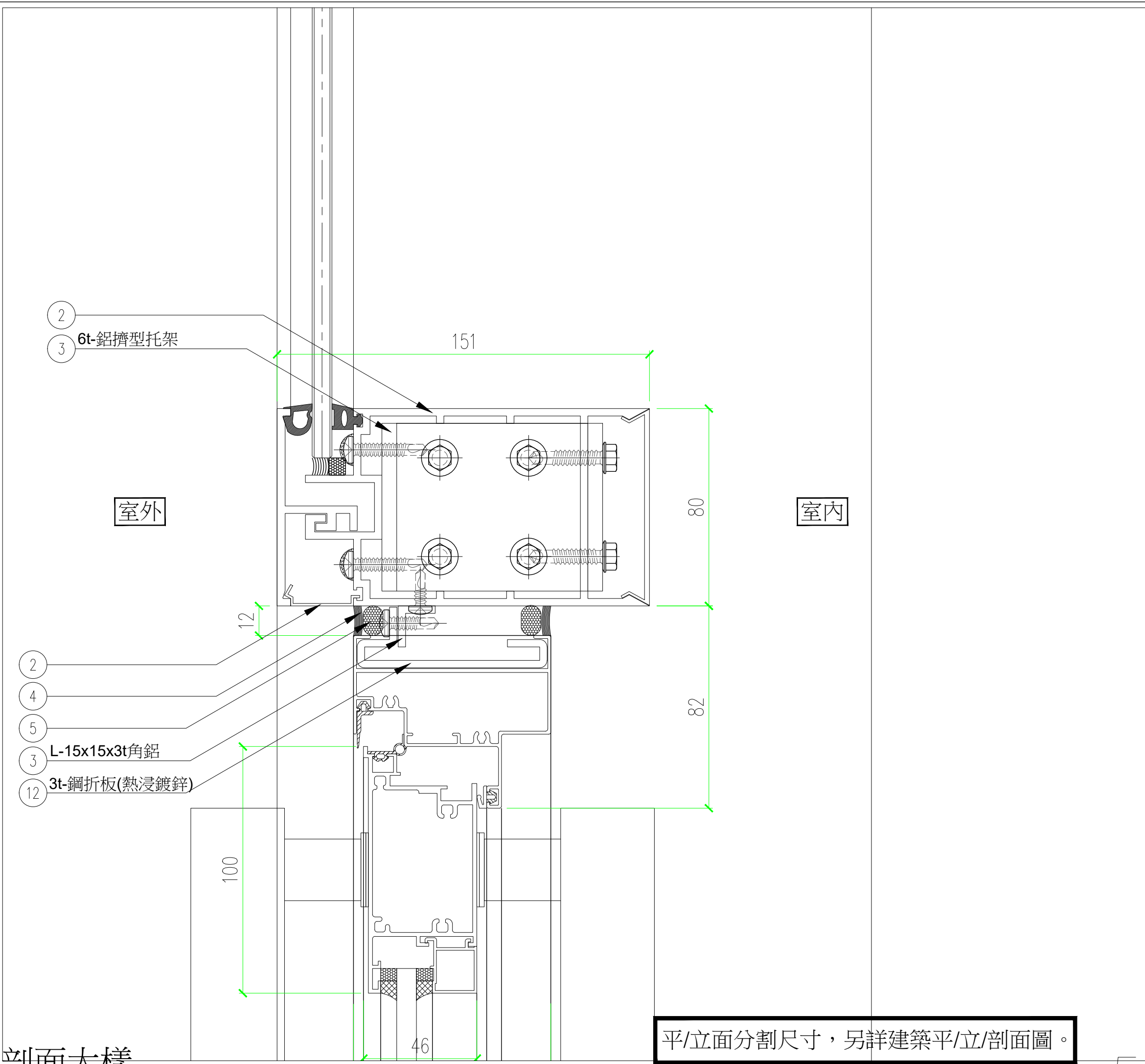
剖面大樣
