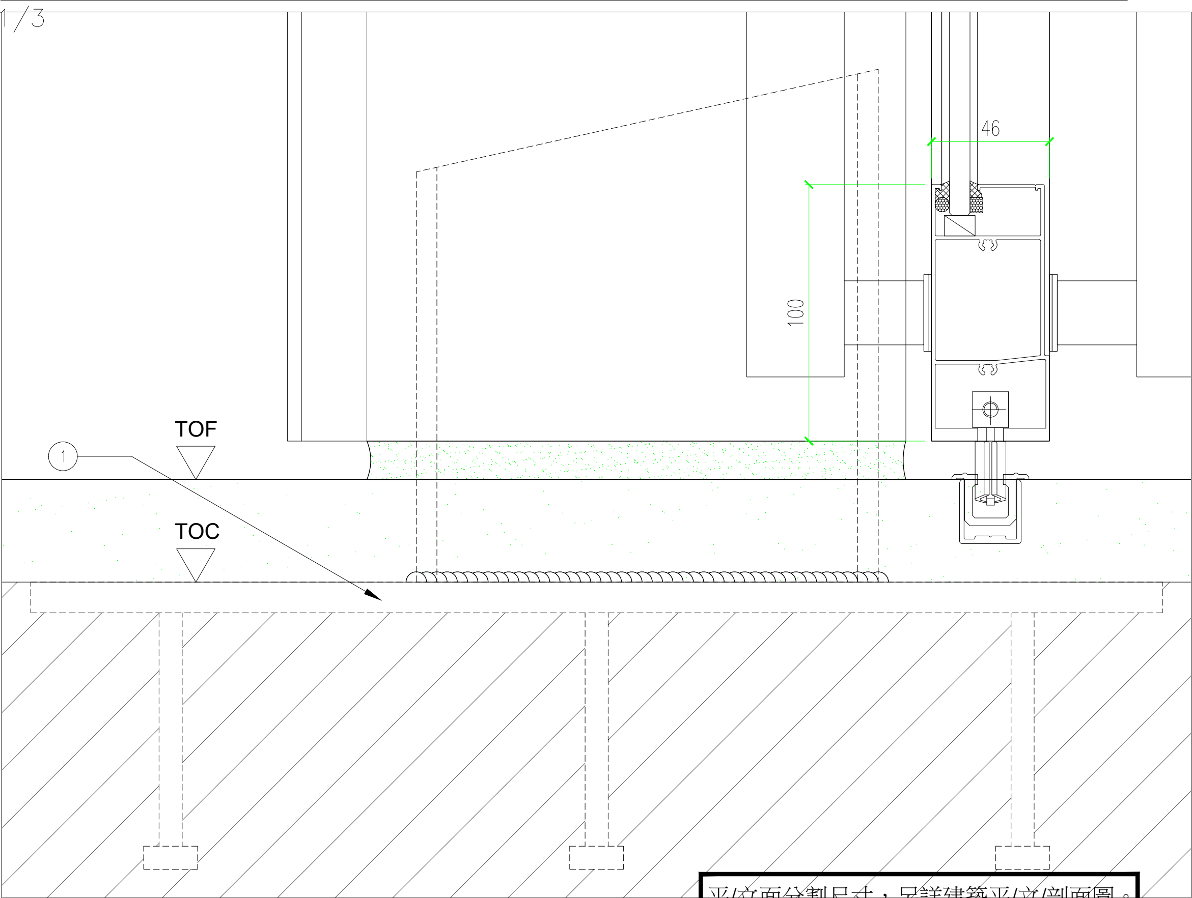
剖面大樣
