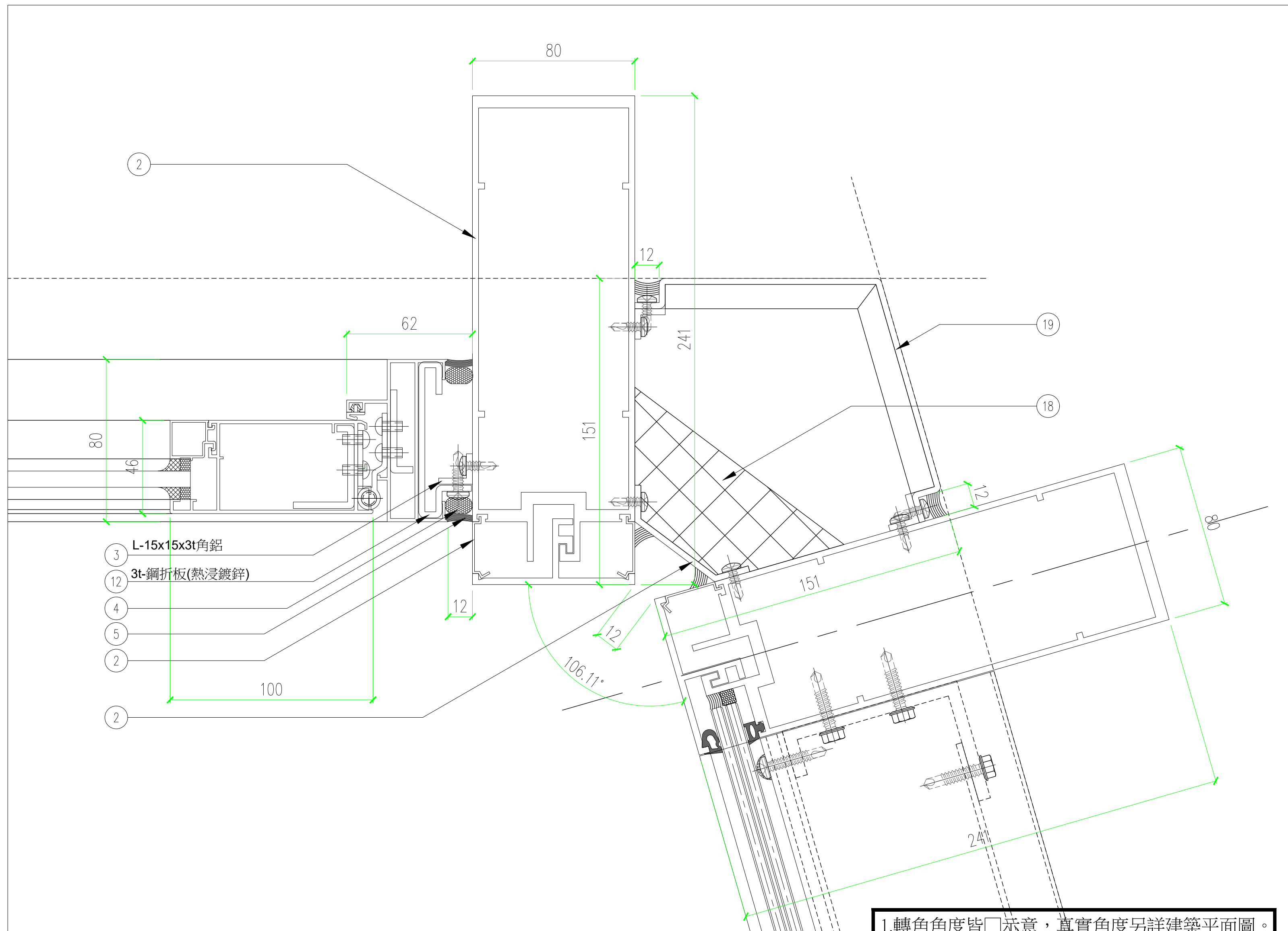
平面大樣 1/3
