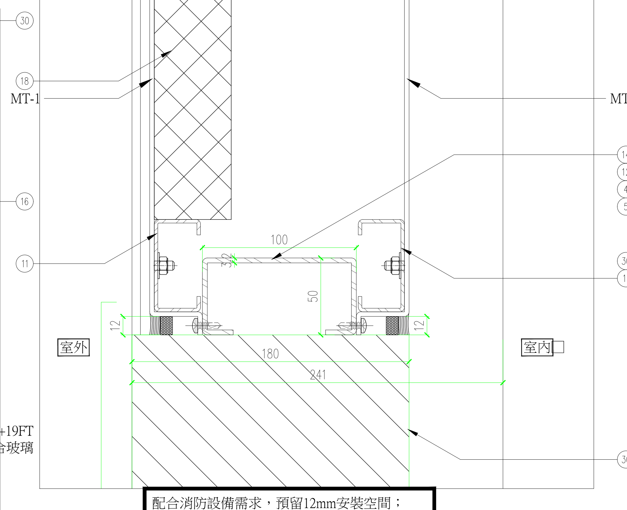
剖面大様
