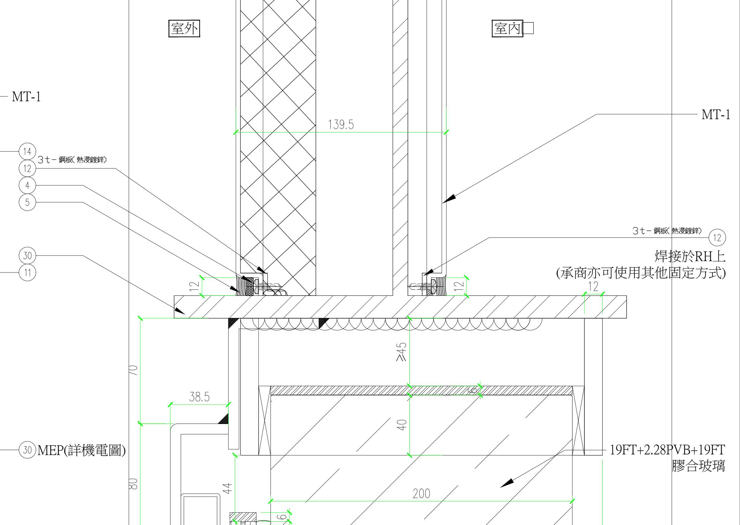
剖面大樣
