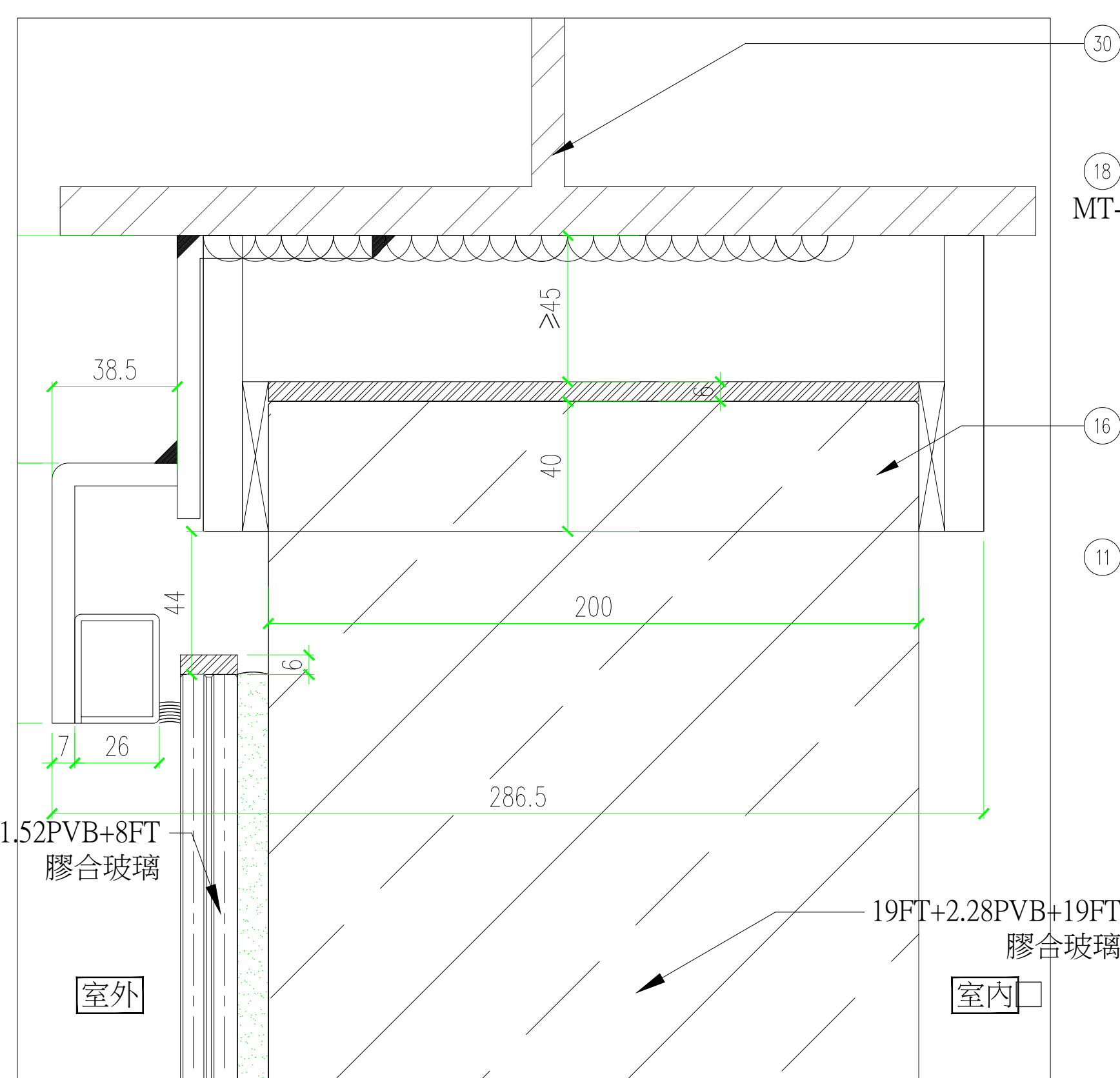
剖面大様
