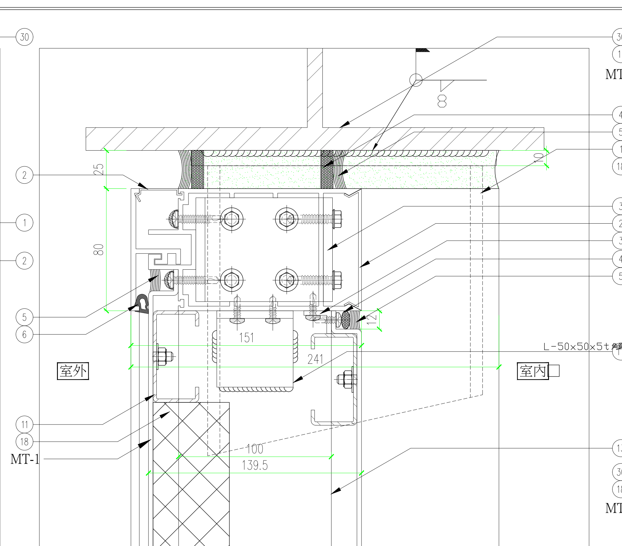
剖面大樣
