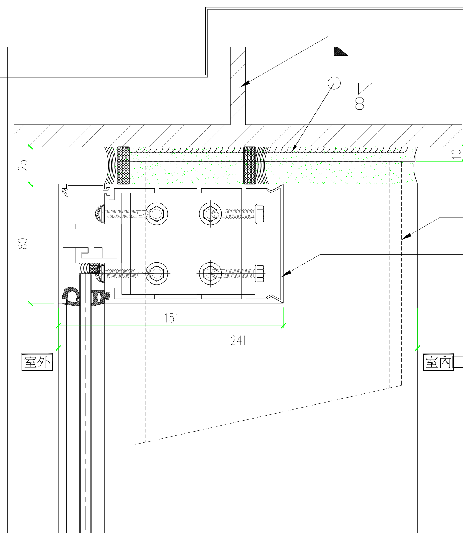
剖面大様
