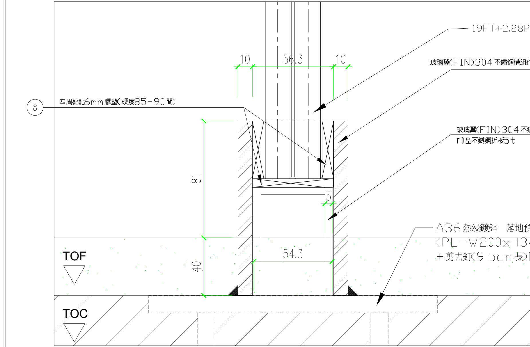
剖面大樣
