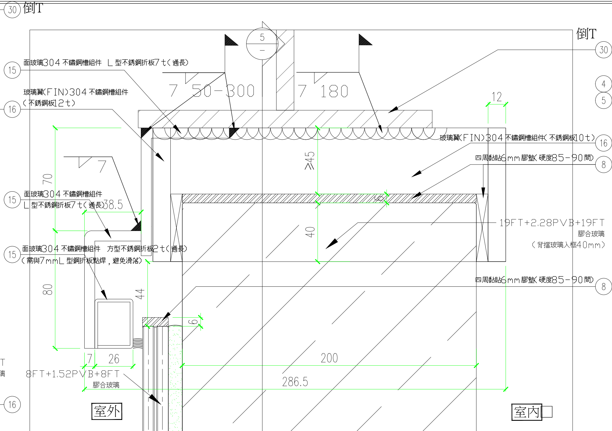
剖面大樣
