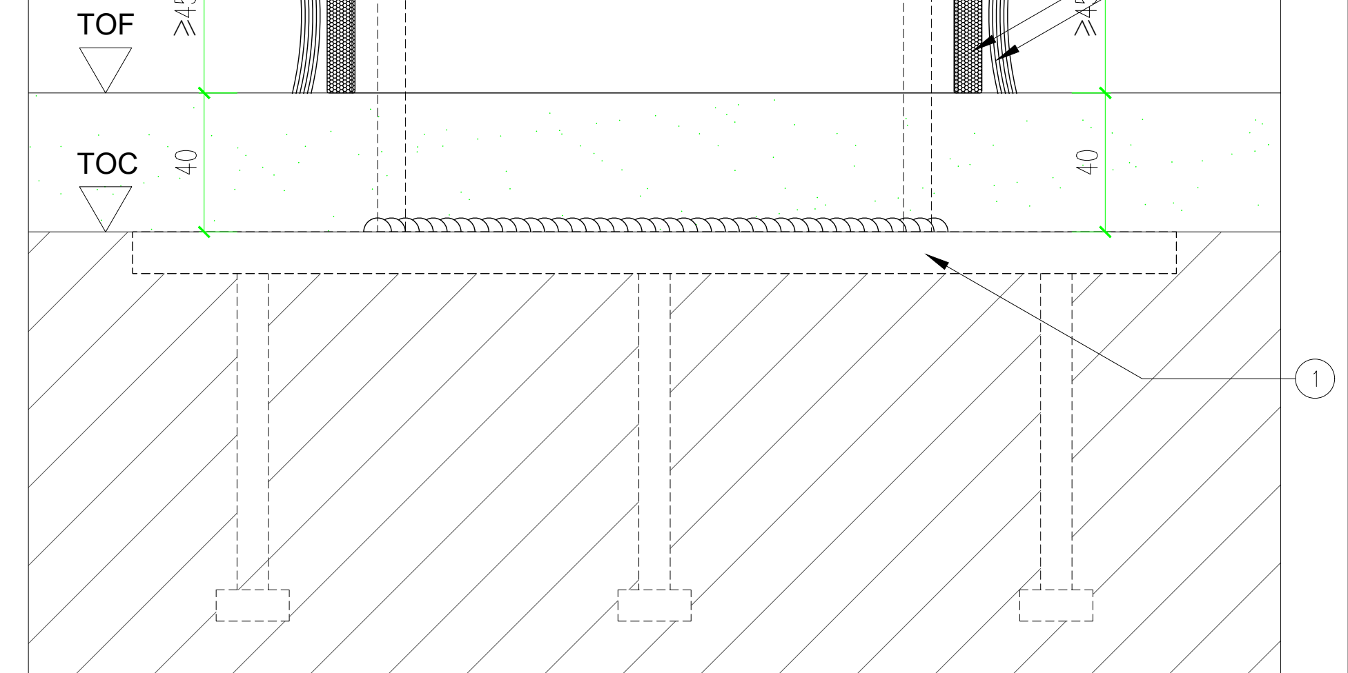
剖面大樣
