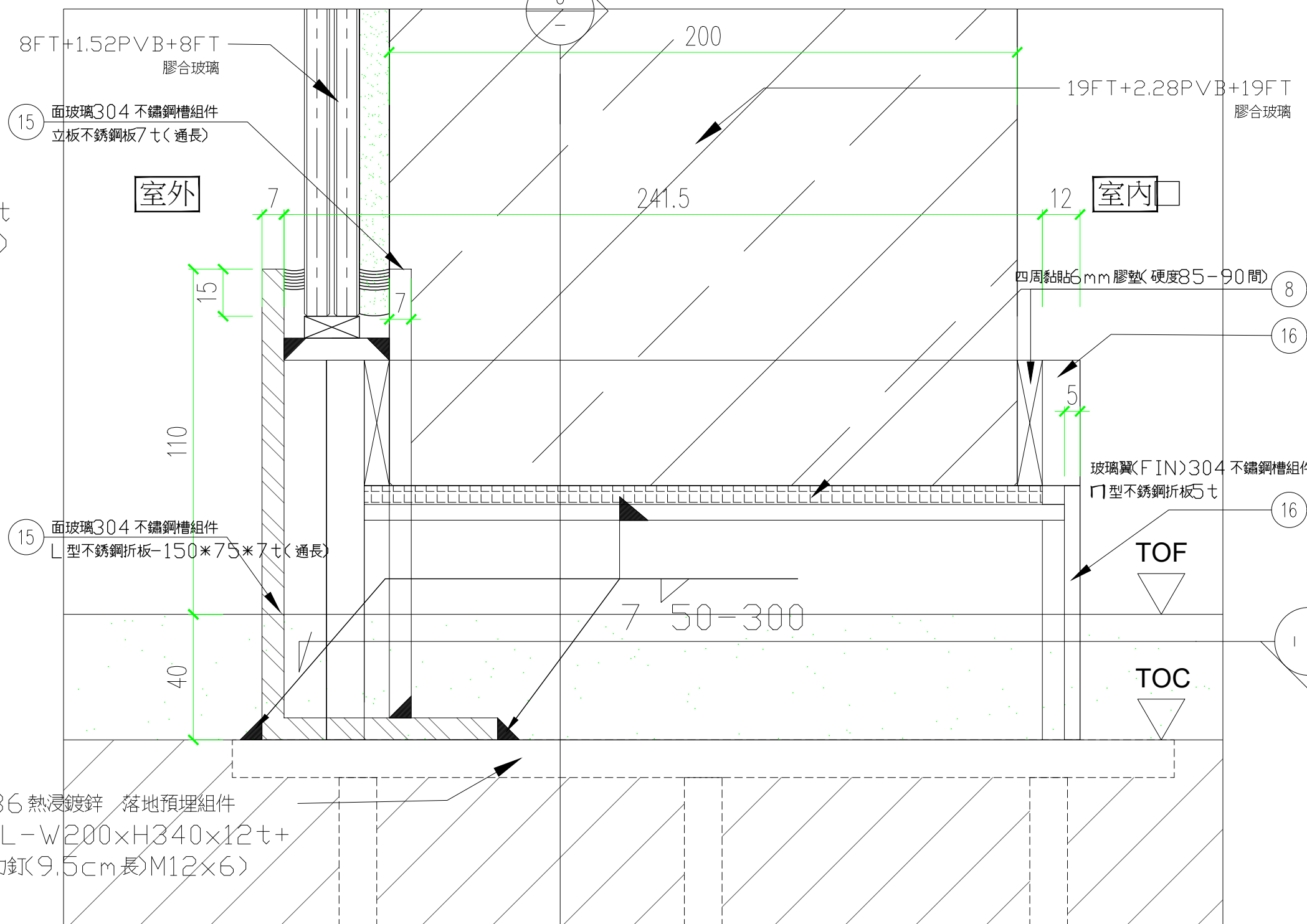
剖面大樣
