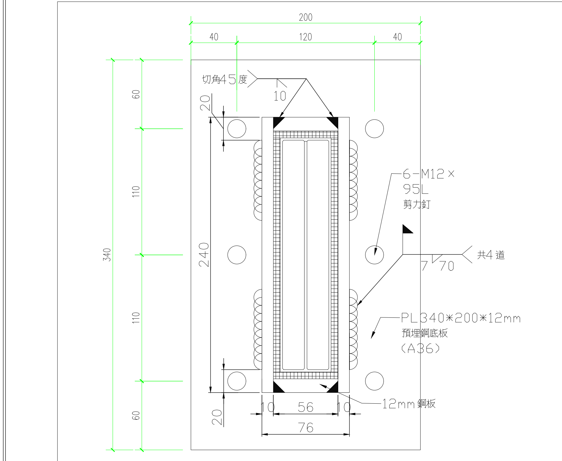
落地預埋組件 大樣
