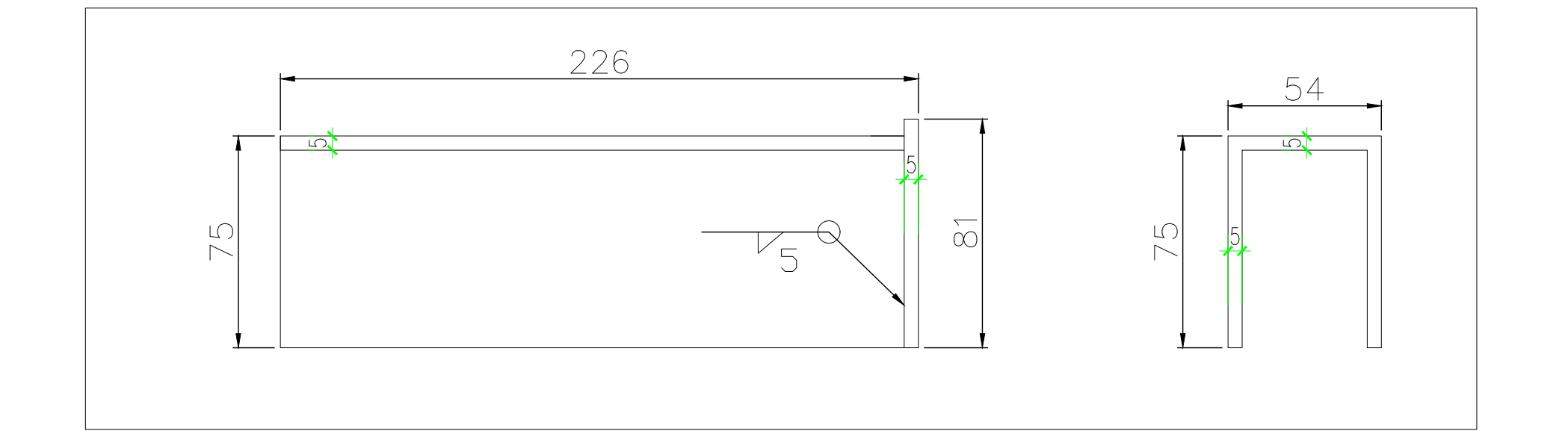
玻璃翼不鏽鋼槽組件 口型不鏽鋼折板 大樣
