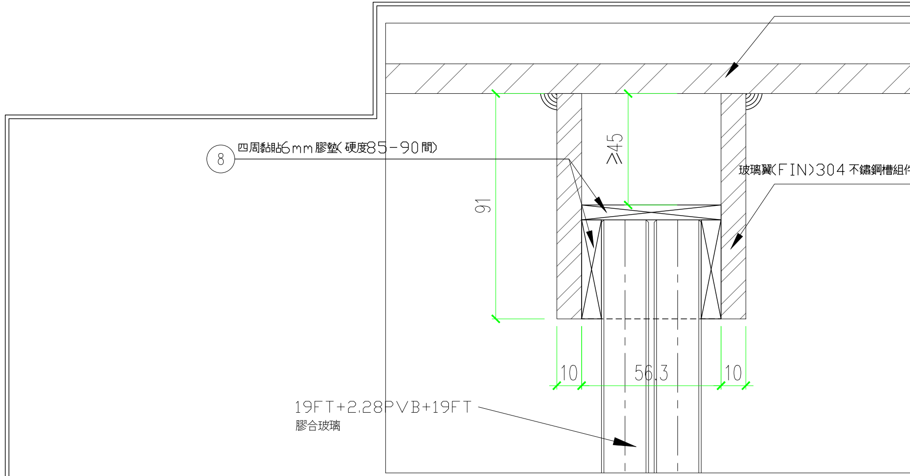
剖面大樣
