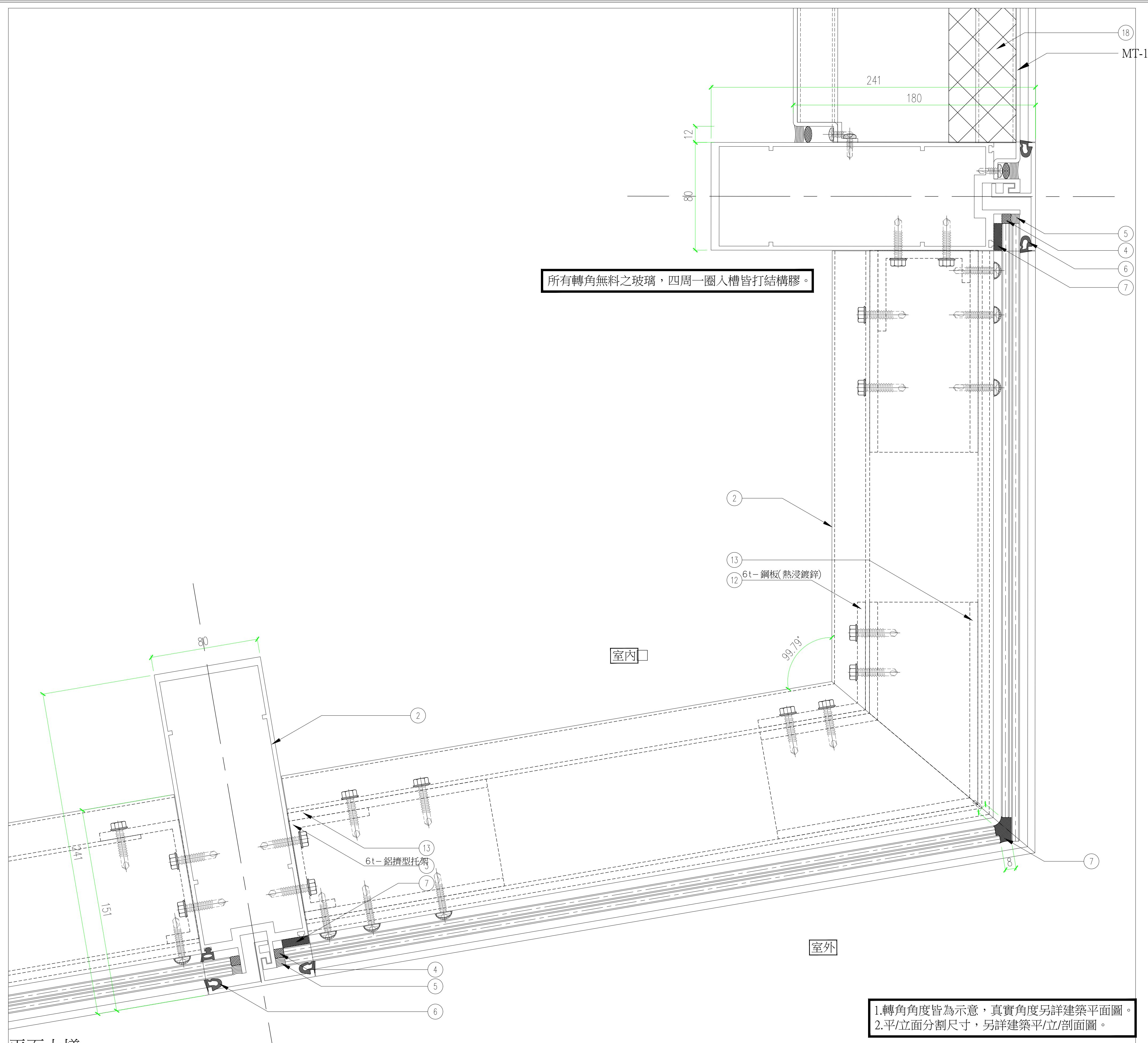
平面大樣 1/3
