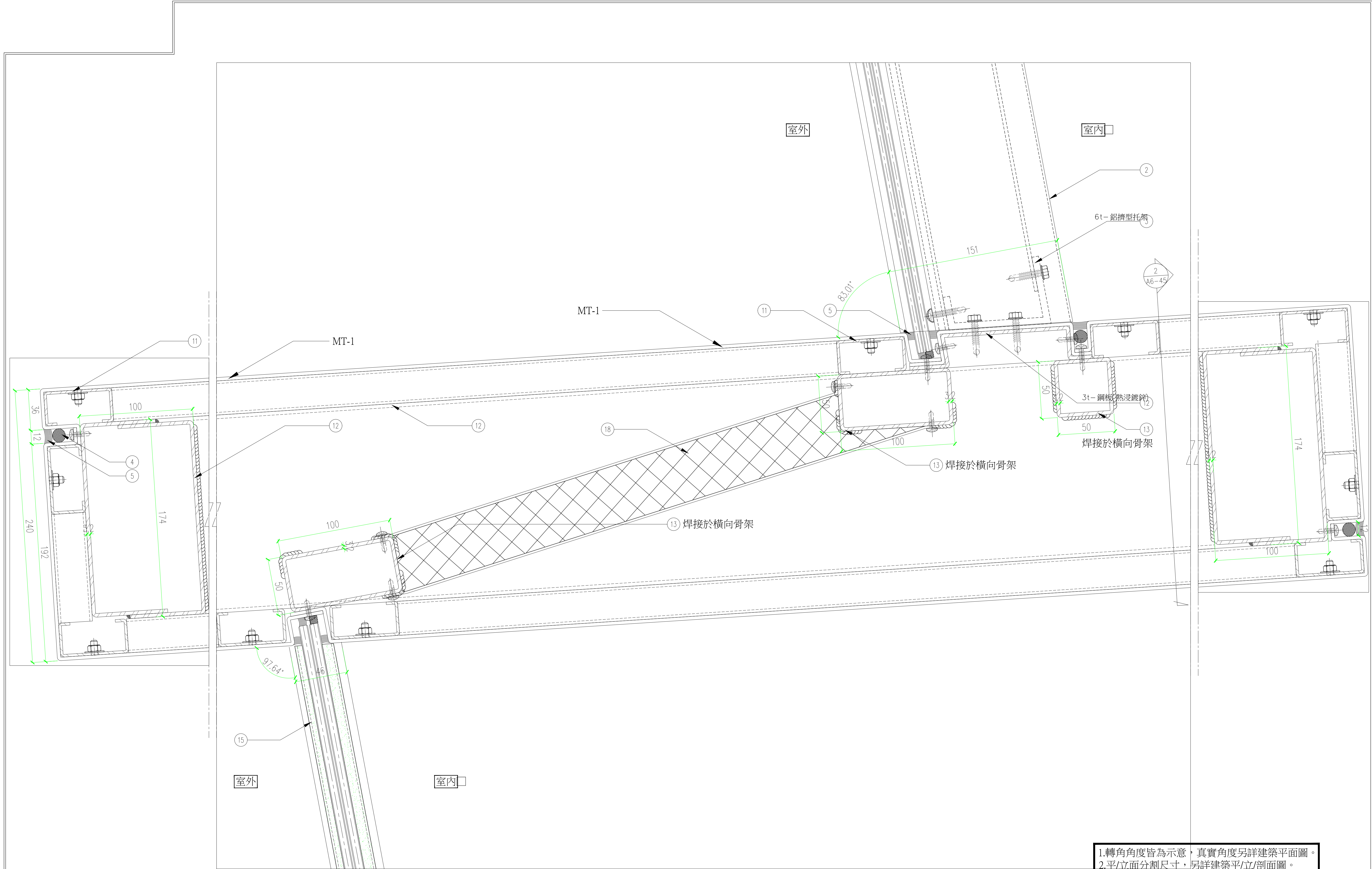
平面大樣 1/3
