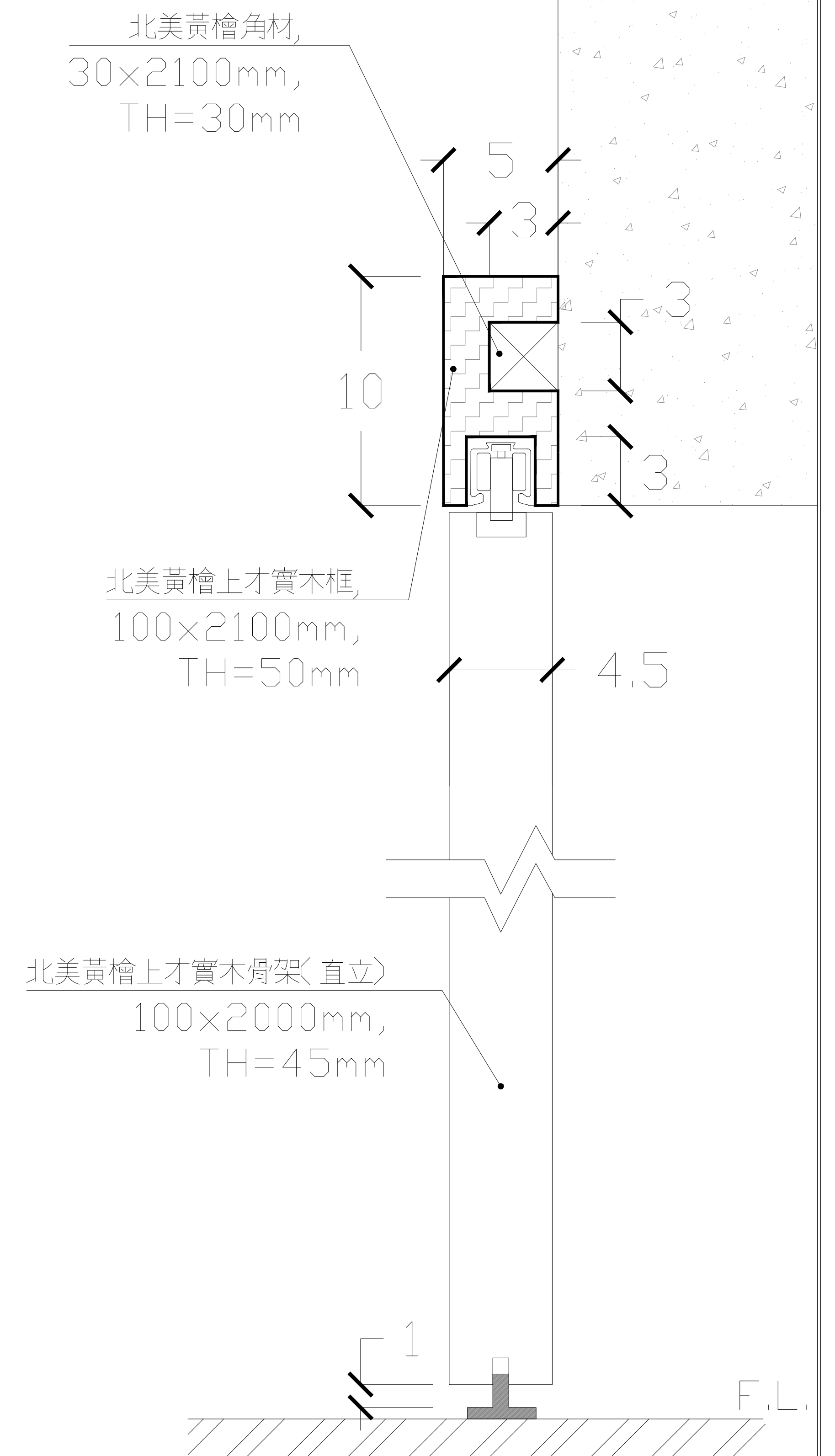
D7 橫拉門門框(含門扇)縱剖 E-E' 剖面詳圖
