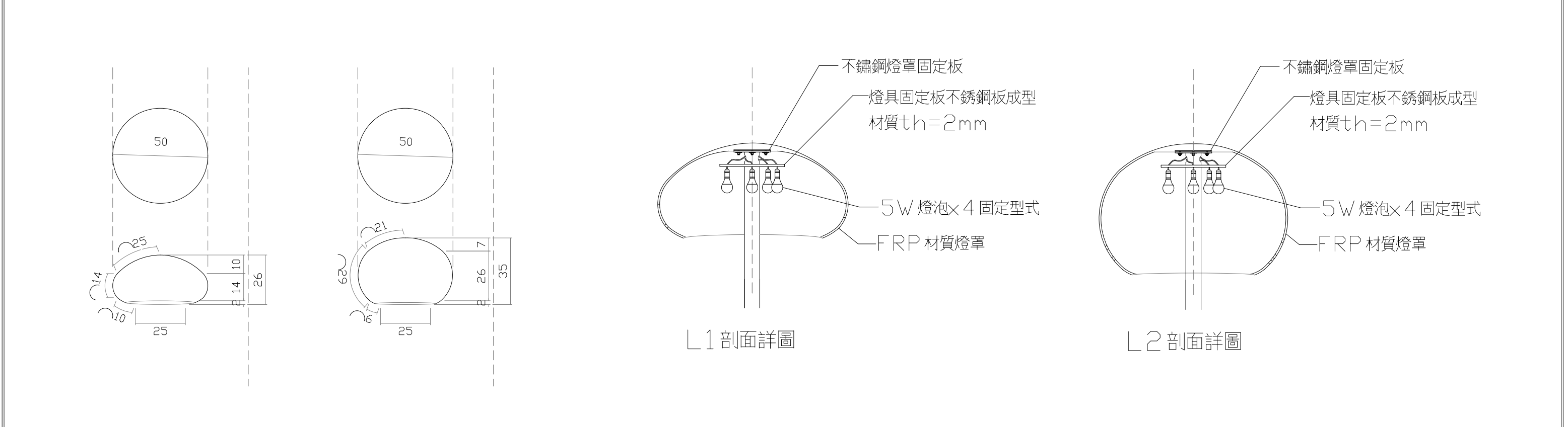
造型矮燈燈罩詳圖
