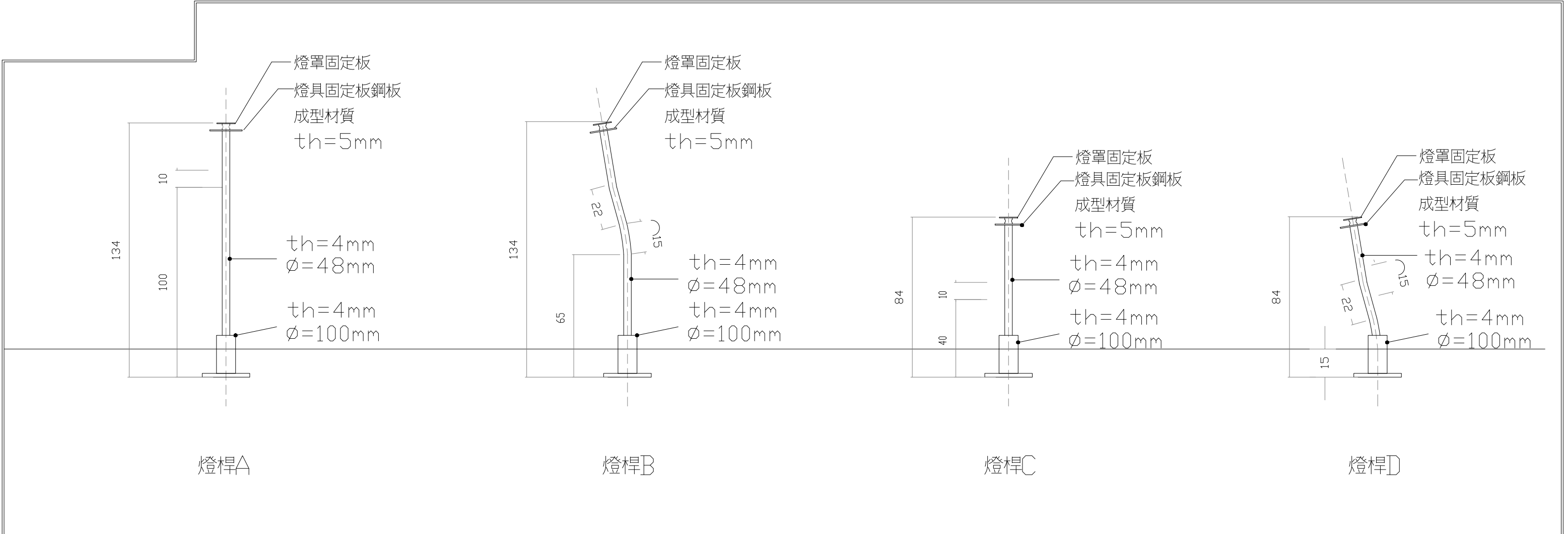
造型矮燈燈桿詳圖
