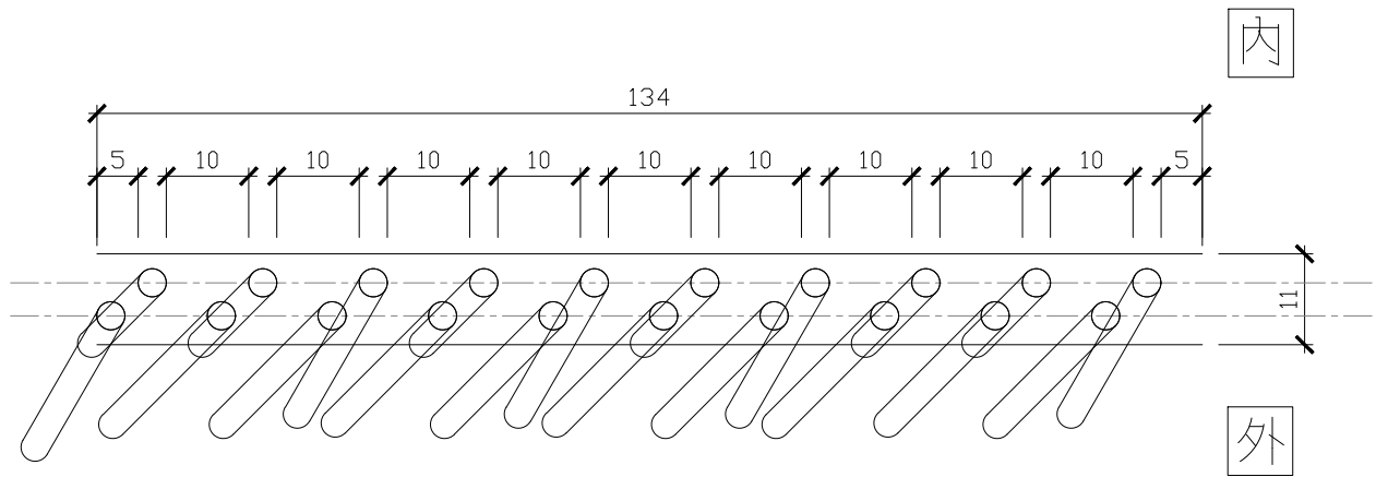
芒草欄杆單元組合詳圖TYPE〈一〉
