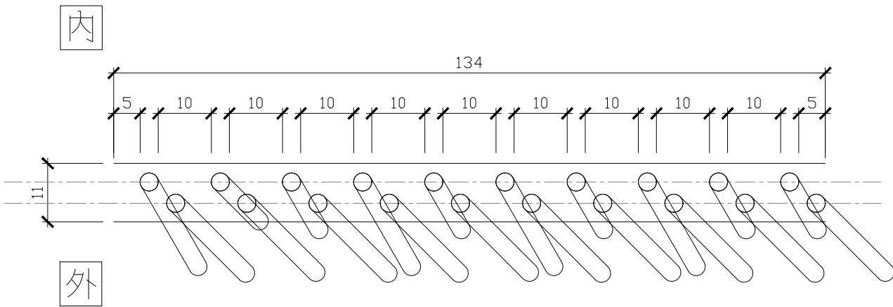
芒草欄杆單元組合詳圖TYPE〈二〉
