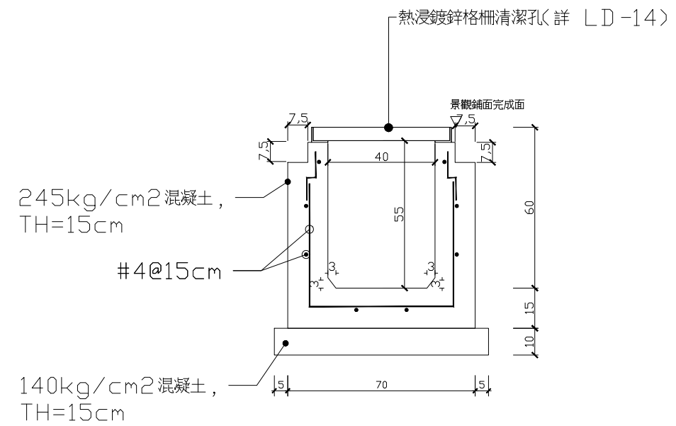
新設陰井B 剖面圖
