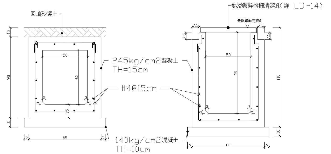
A-A' 剖面圖
