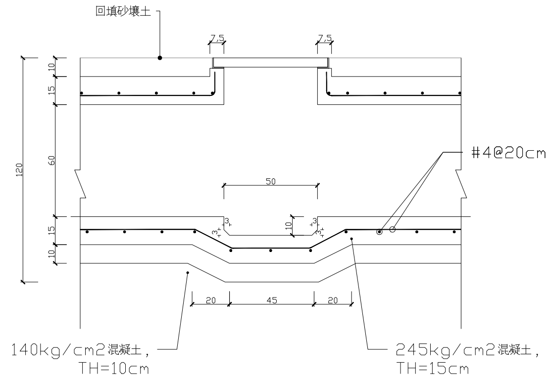
B-B' 剖面圖
