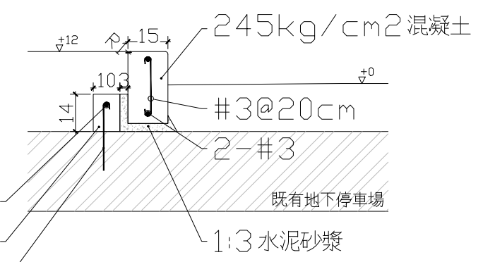
C-C' 預鑄RC路緣石剖面圖
