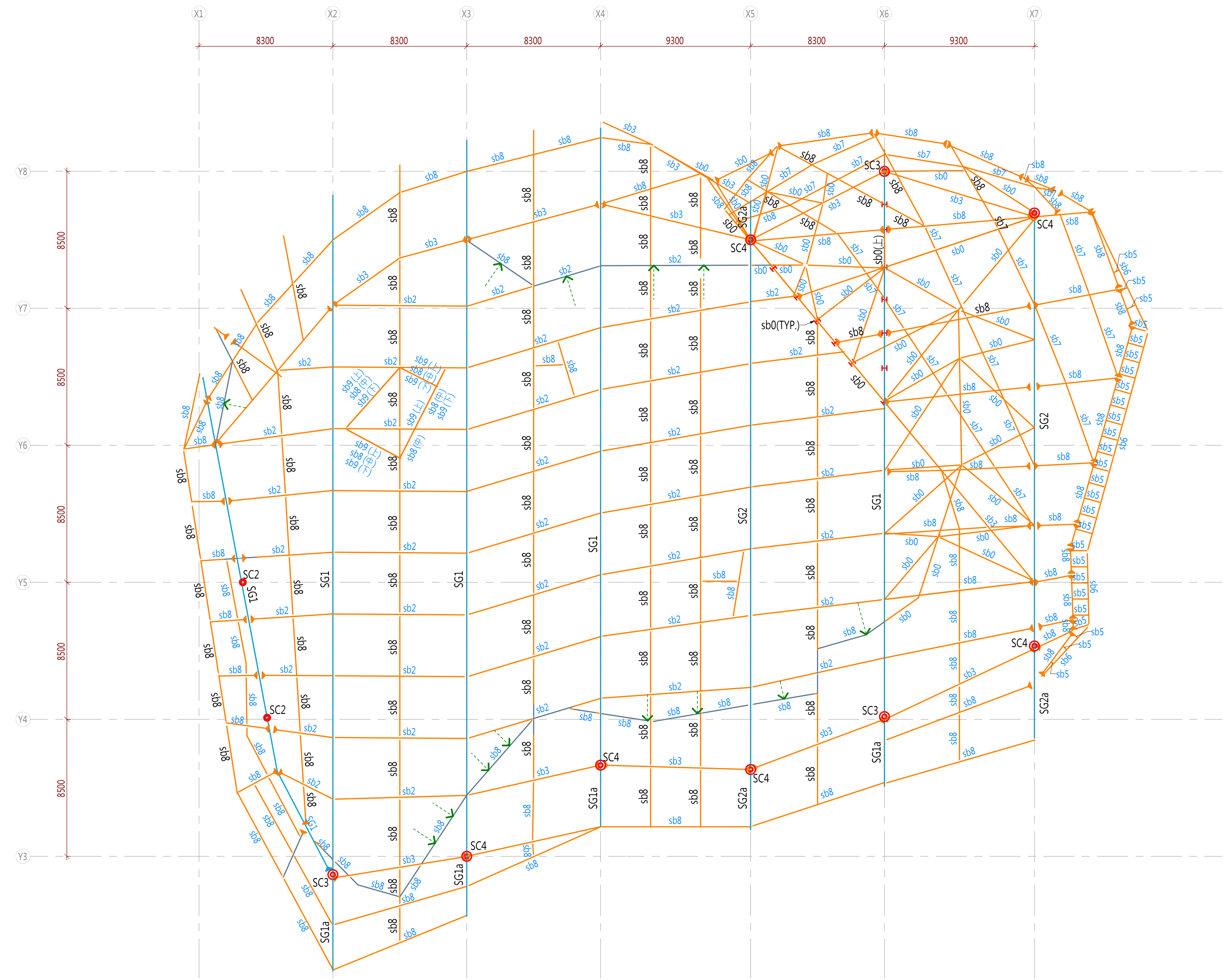
1 S9-30 體育館屋頂鋼構結構平面圖 1:150
