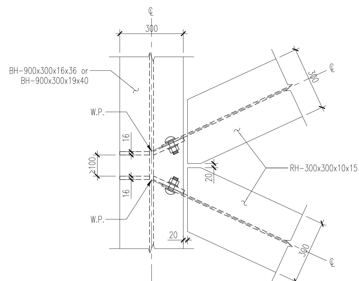
5A RH-300x300斜桿頂部接合詳圖(二) S9-22 S:1/10
