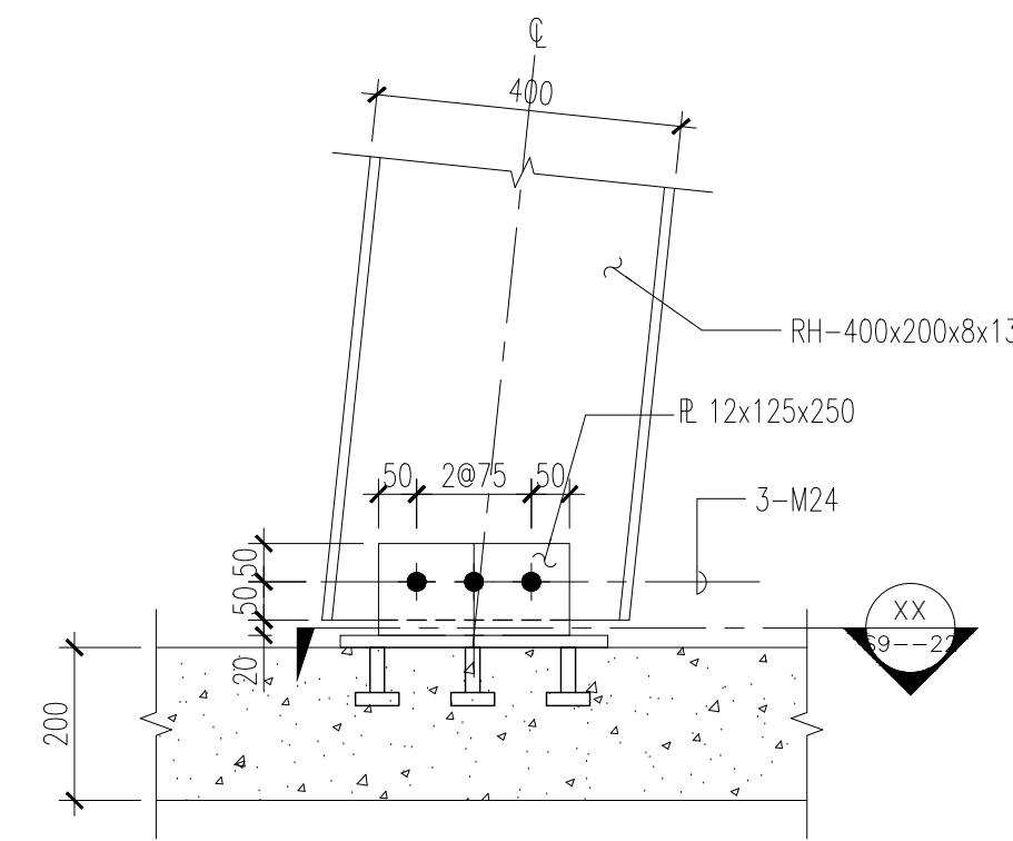
3 RH400x200與樓版接合詳圖(一) S9-22 S:1/10
