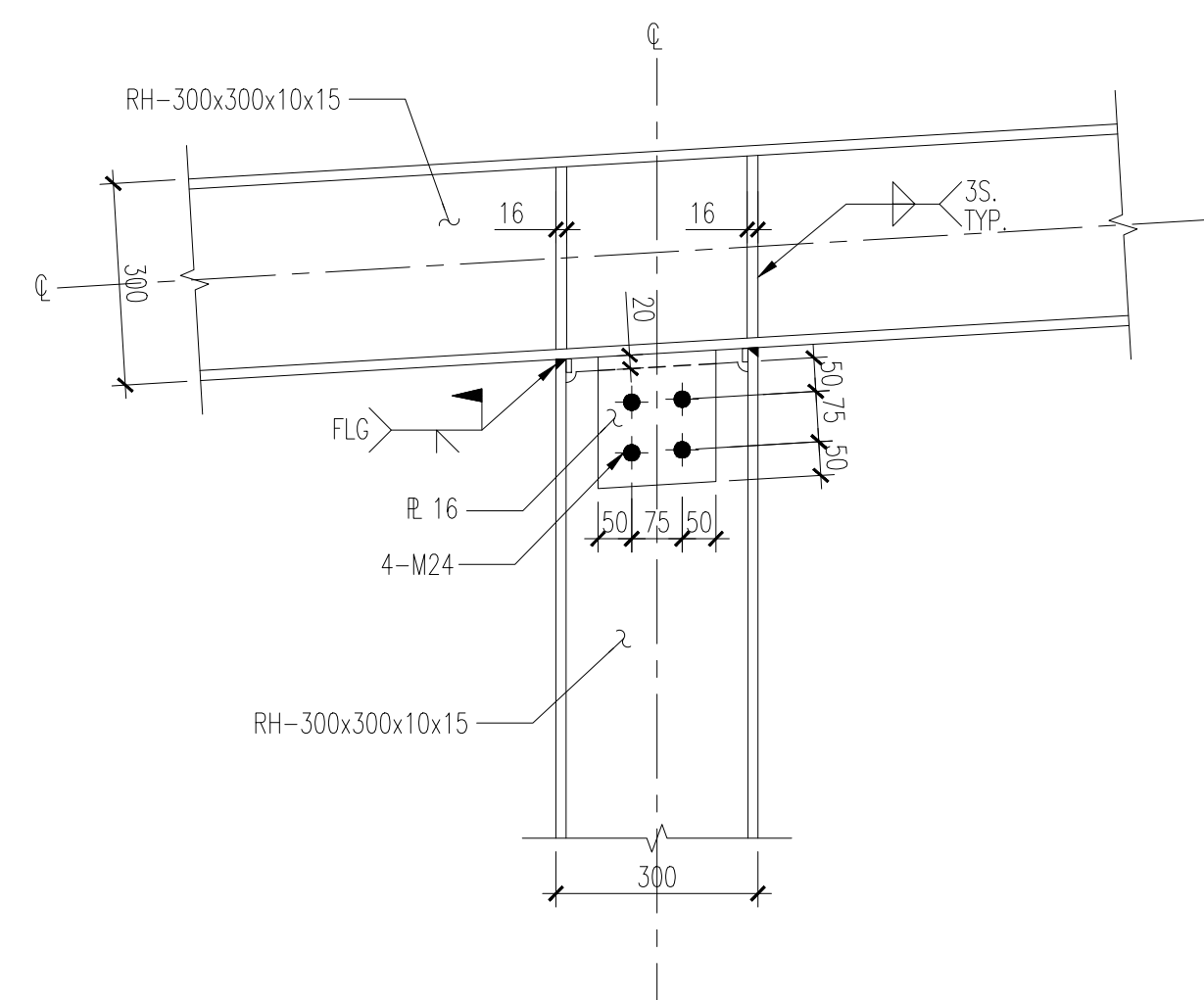
6B RH-300x300柱頂接合詳圖 S9-22 S:1/10
