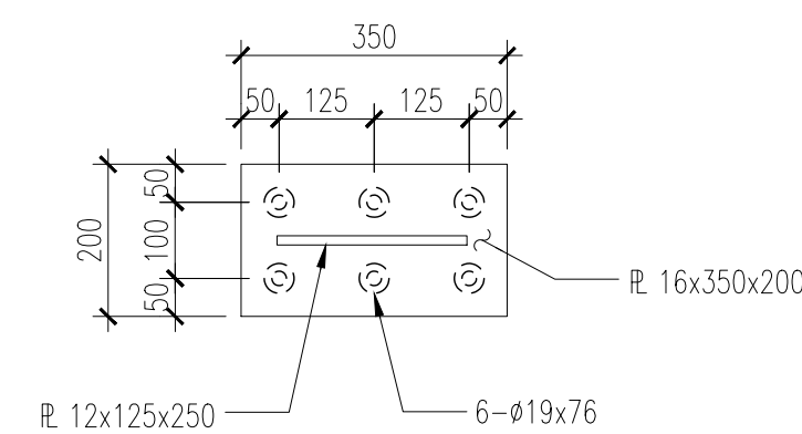
3A RH400x200與樓版接合詳圖(二) S9-22 S:1/10
