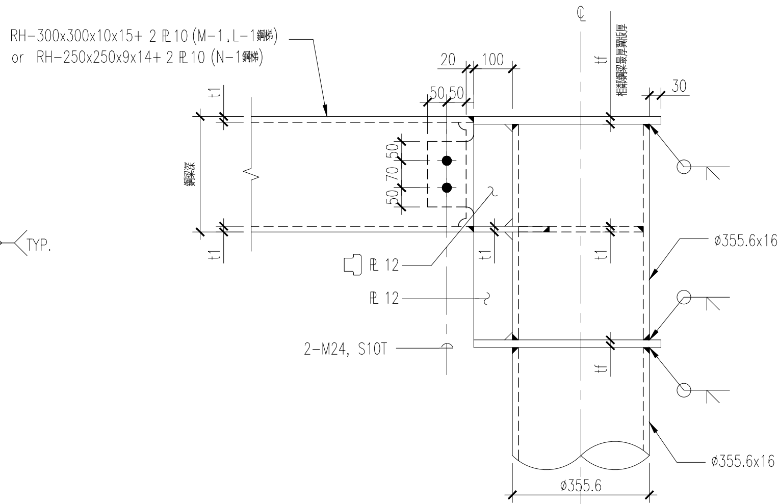
3 鋼樓梯詳圖(三) S9.02 S:1/10
