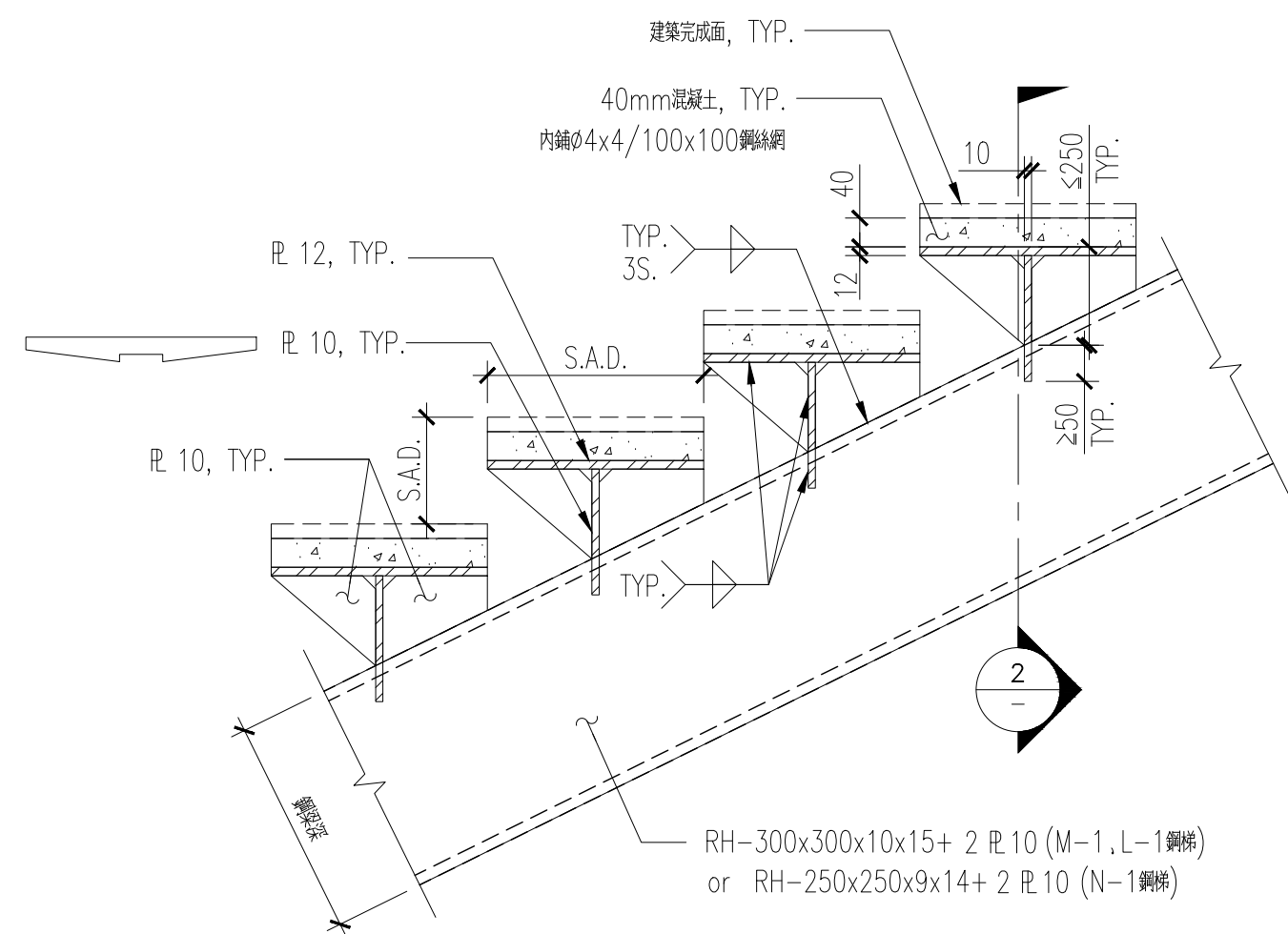
1 鋼樓梯詳圖(一) S9.02 S:1/10
