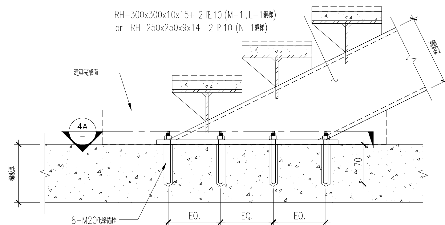
5 鋼樓梯詳圖(五) S9.02 S:1/10
