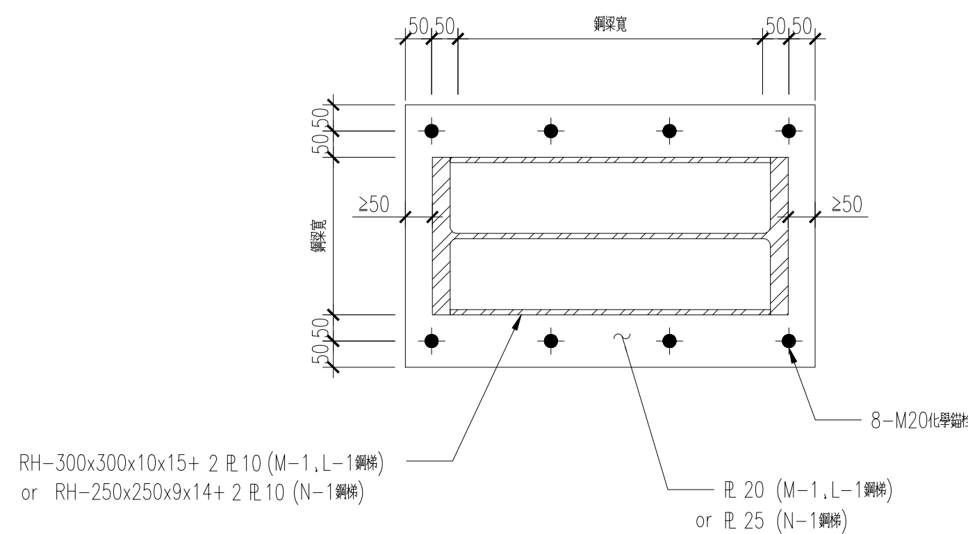
4A 鋼樓梯詳圖(六) S9.02 S:1/10
