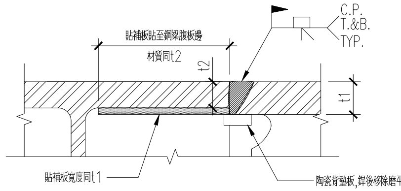
3A 固接板厚差細部詳圖
