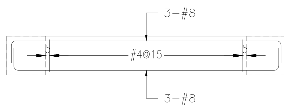
2F B150 (30x50)
