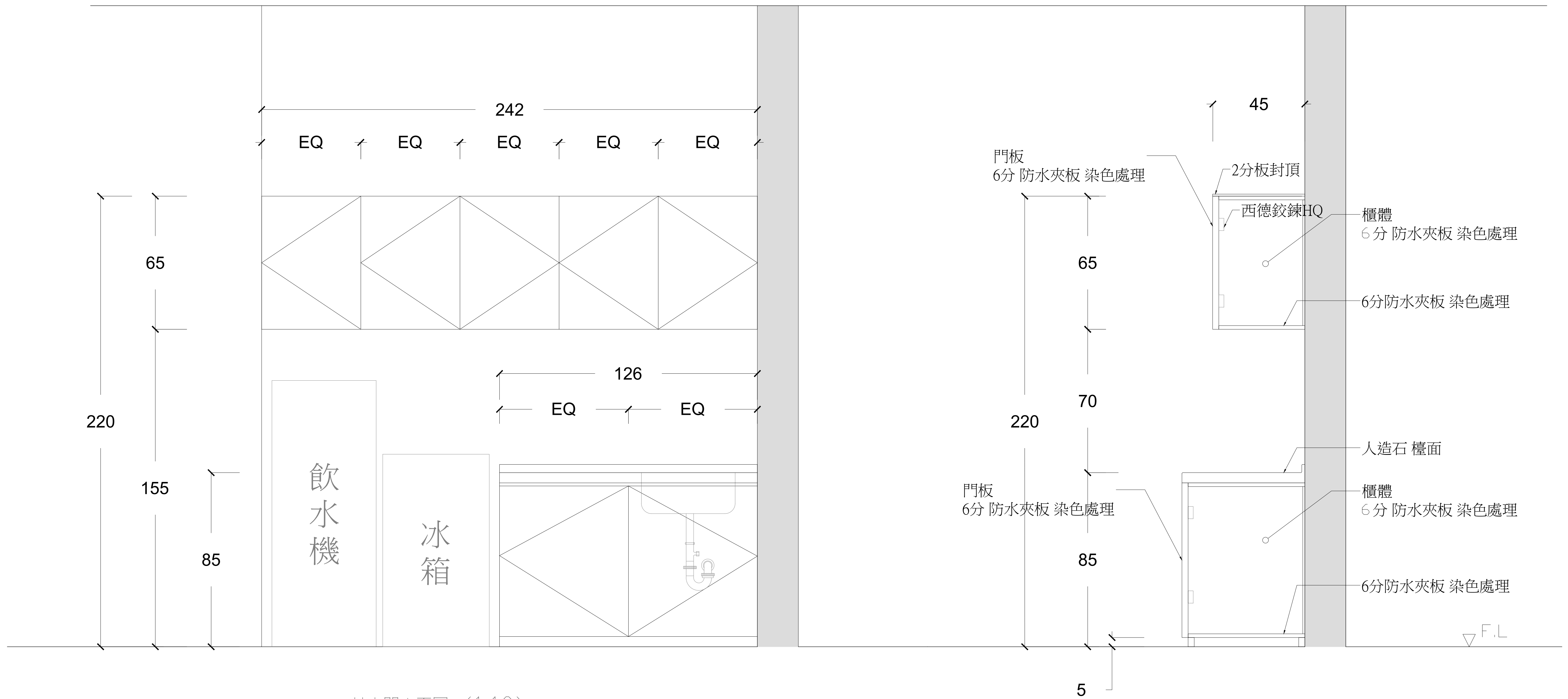
茶水間 木櫃剖面圖 〈1:10〉
