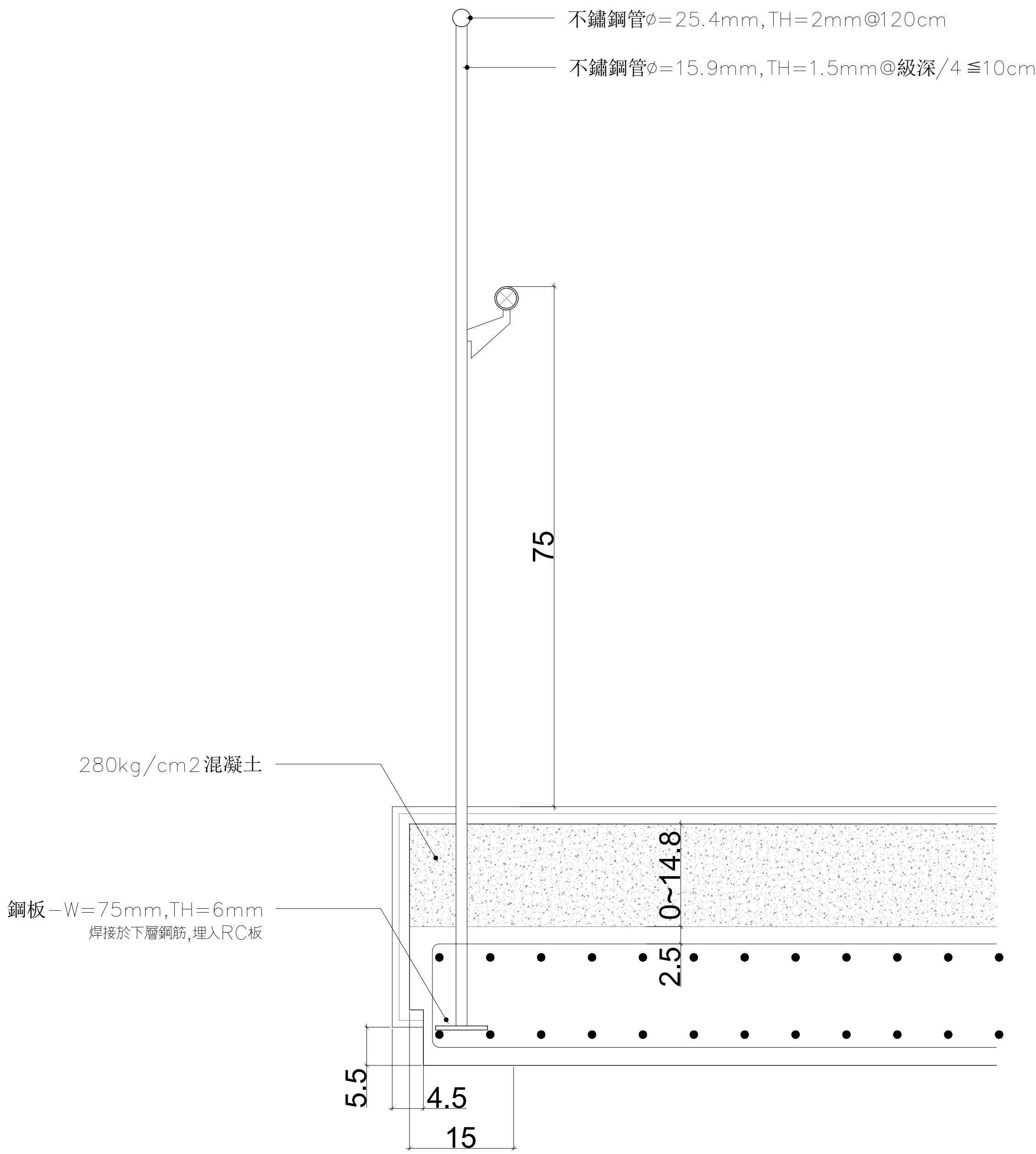
02 不銹鋼欄杆C 樓梯段剖面圖 S1/10
