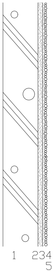
W3 外牆面1:3 水泥砂漿摻無機色粉( 色另定) 嵌1,2 分蛇紋石+ 寒水石+ 特白石
