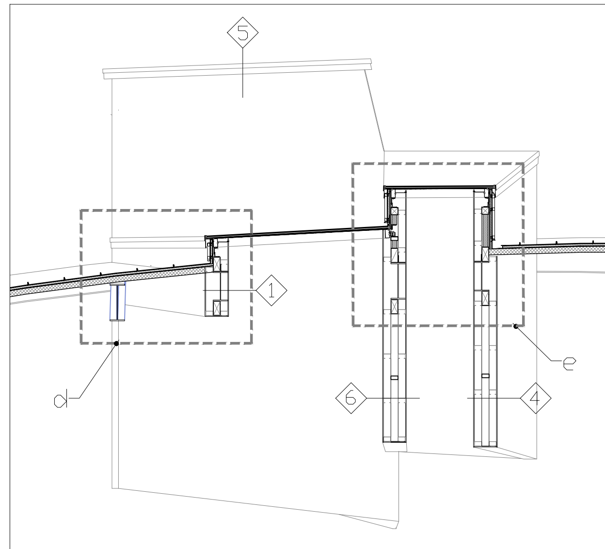
B 型天窗 剖面2-1 細部索引圖
