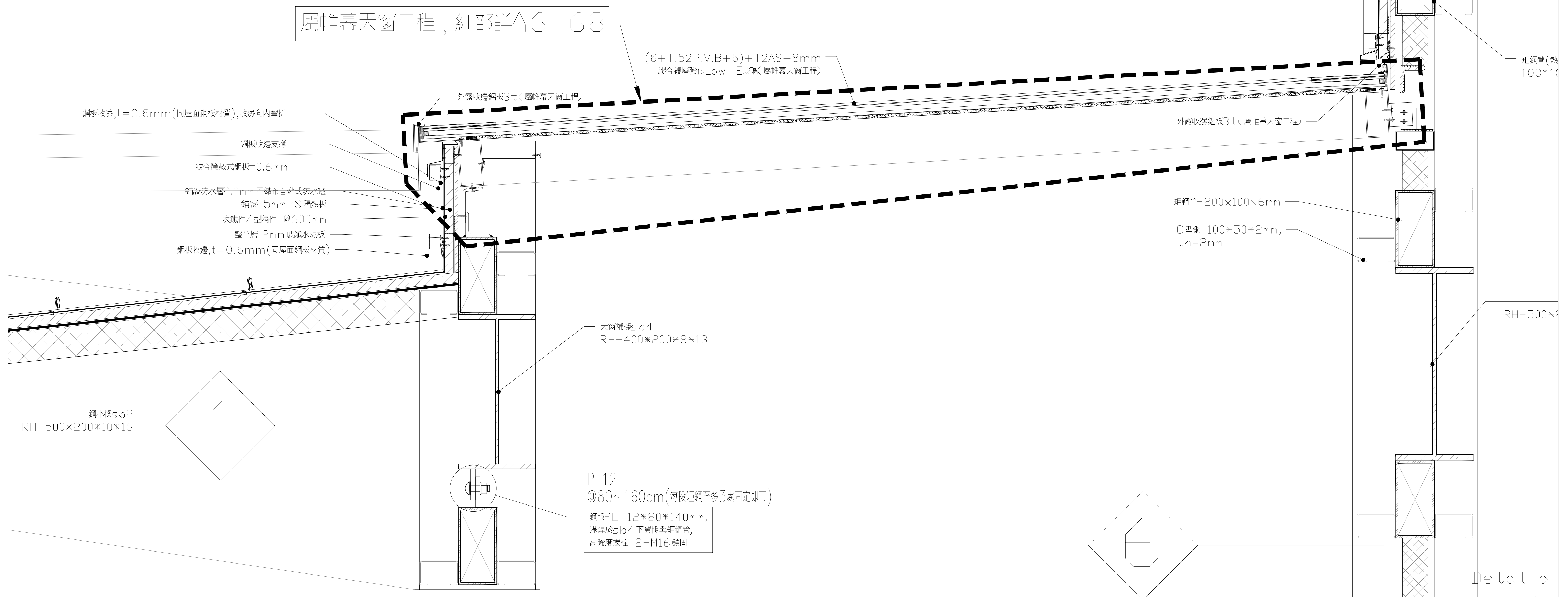
B 型天窗 剖面2-細部詳圖
