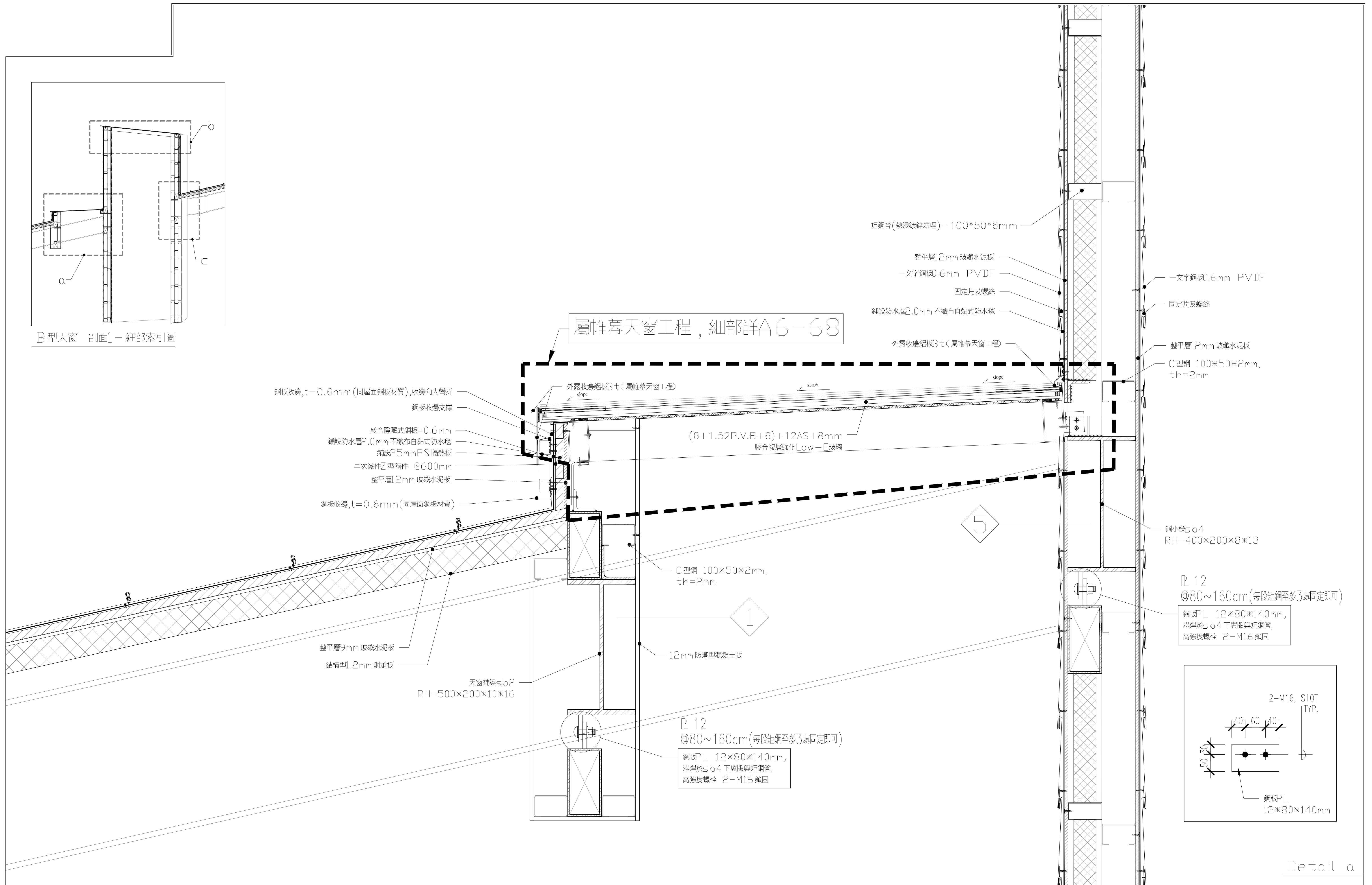
B型天窗 剖面1-細部詳圖
