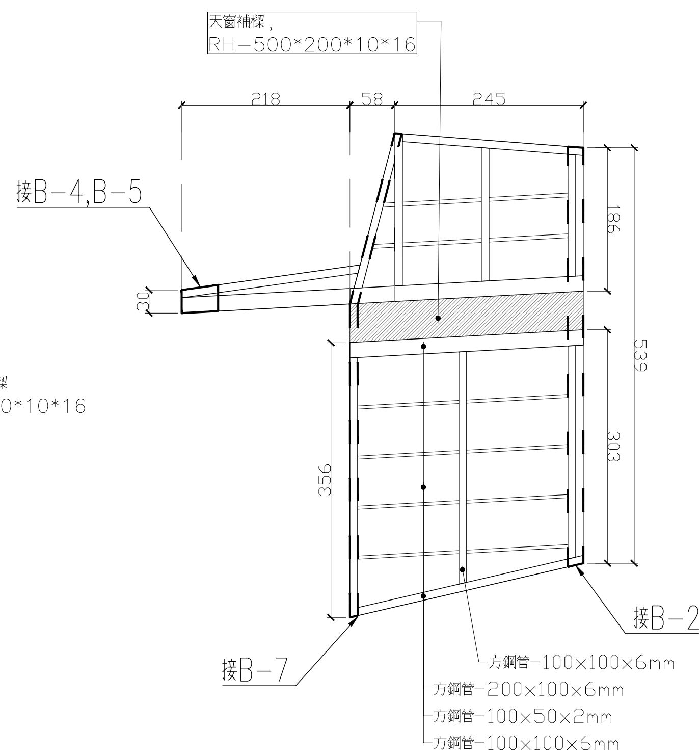
③ B-3 ( 室外紋合隱藏式鋼板,12mm 防潮型混凝土版 )
