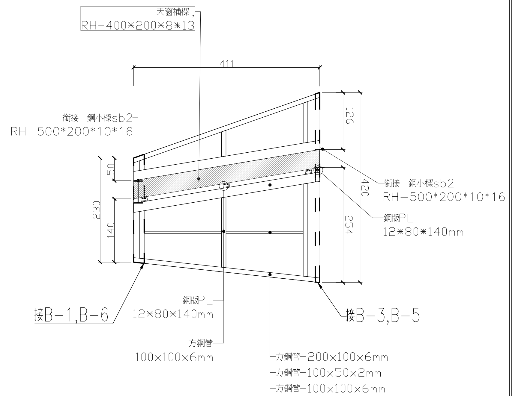
④ B-4 ( 室外紋合隱藏式鋼板,12mm 防潮型混凝土版 )
