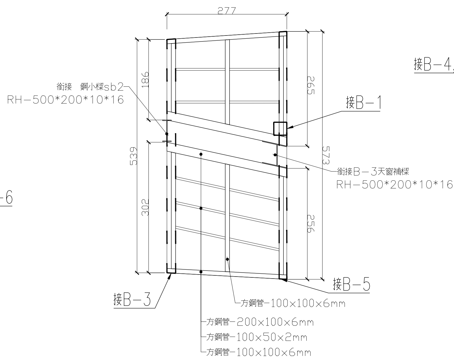
② B-2 ( 室外紋合隱藏式鋼板,12mm 防潮型混凝土版 )
