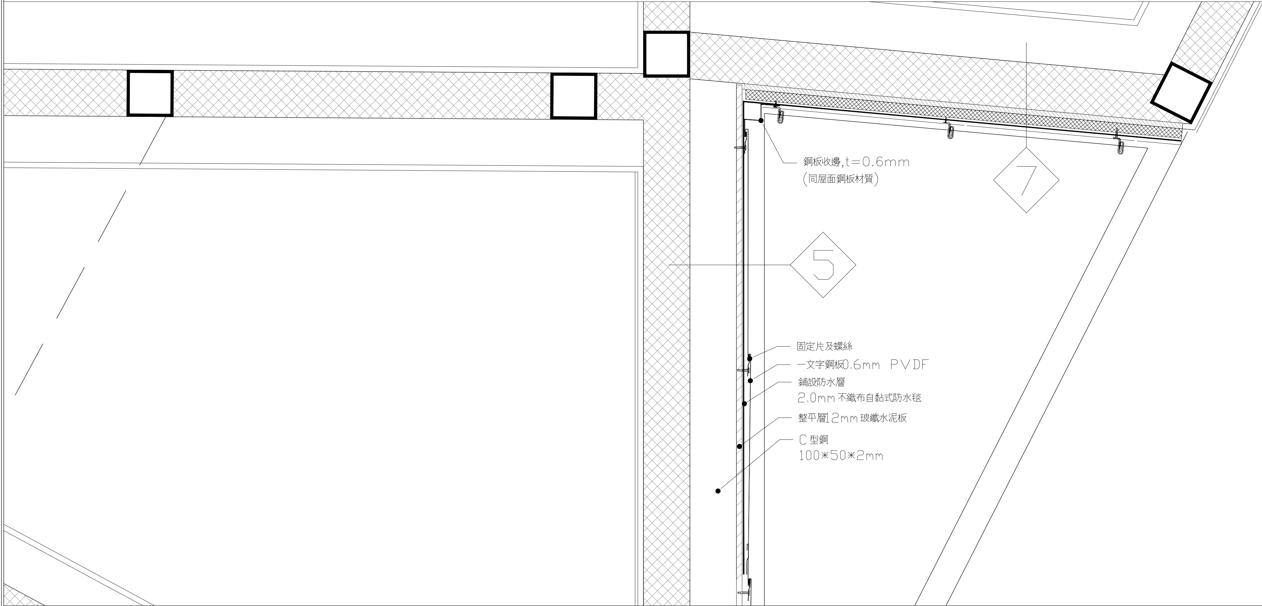
B 型天窗牆面 一文字橫式／鉸合隱藏式銅板收邊詳圖
