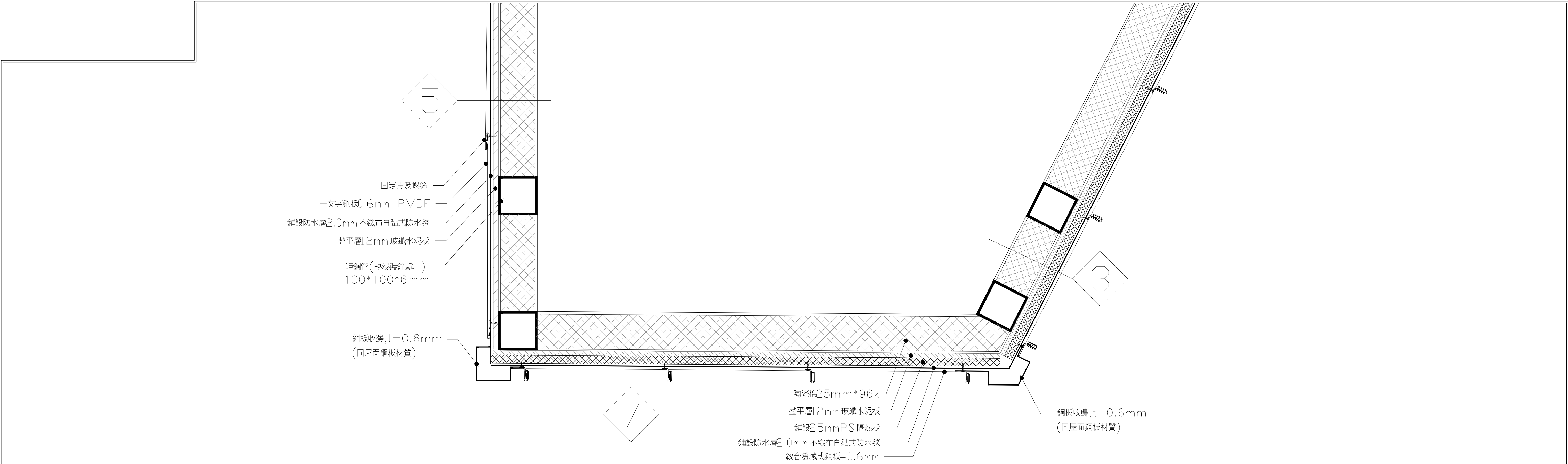
B-3,B-5,B-7 陽角銅板收邊詳圖
