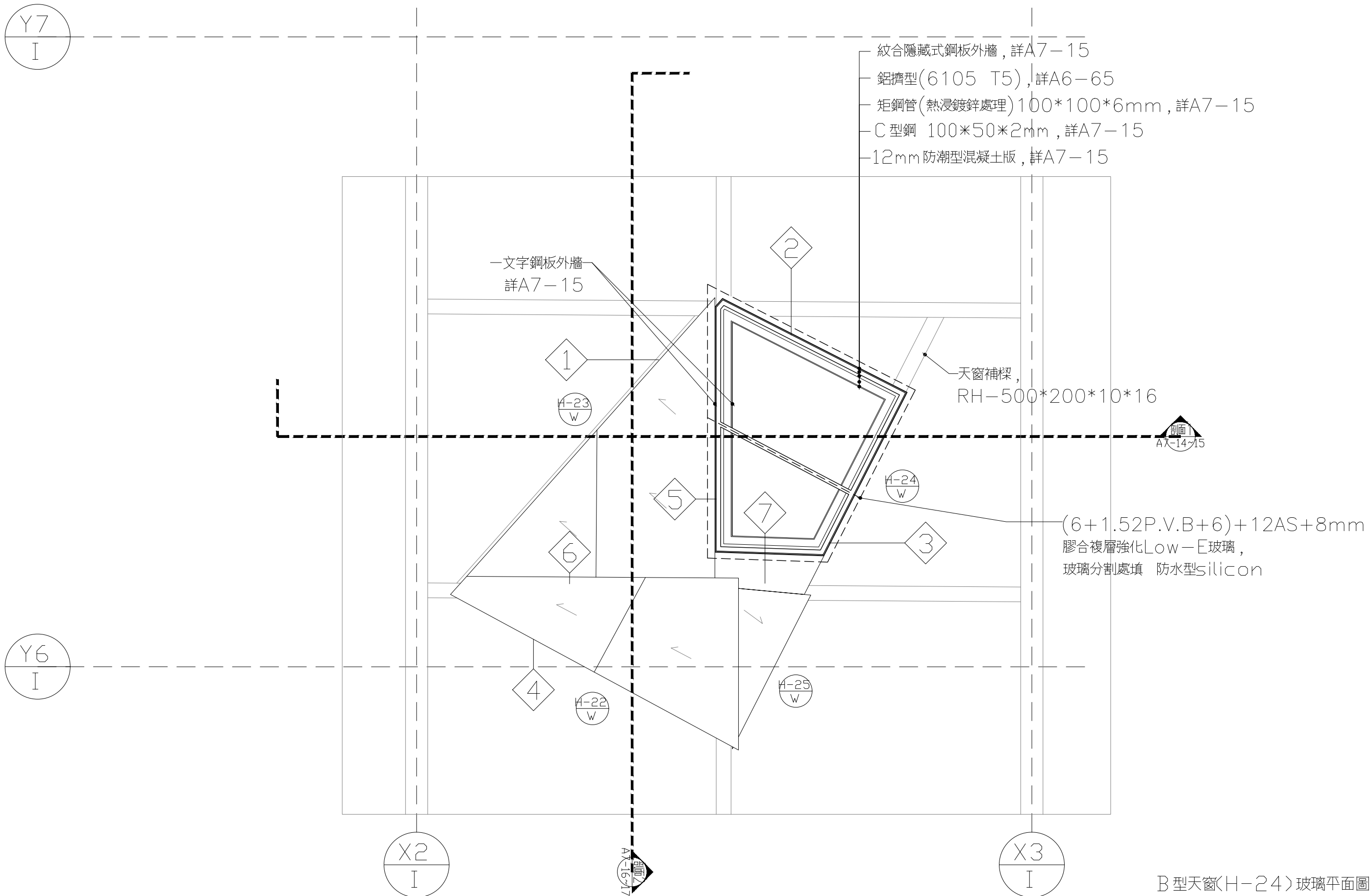
B 型天窗(H-24)玻璃平面圖
