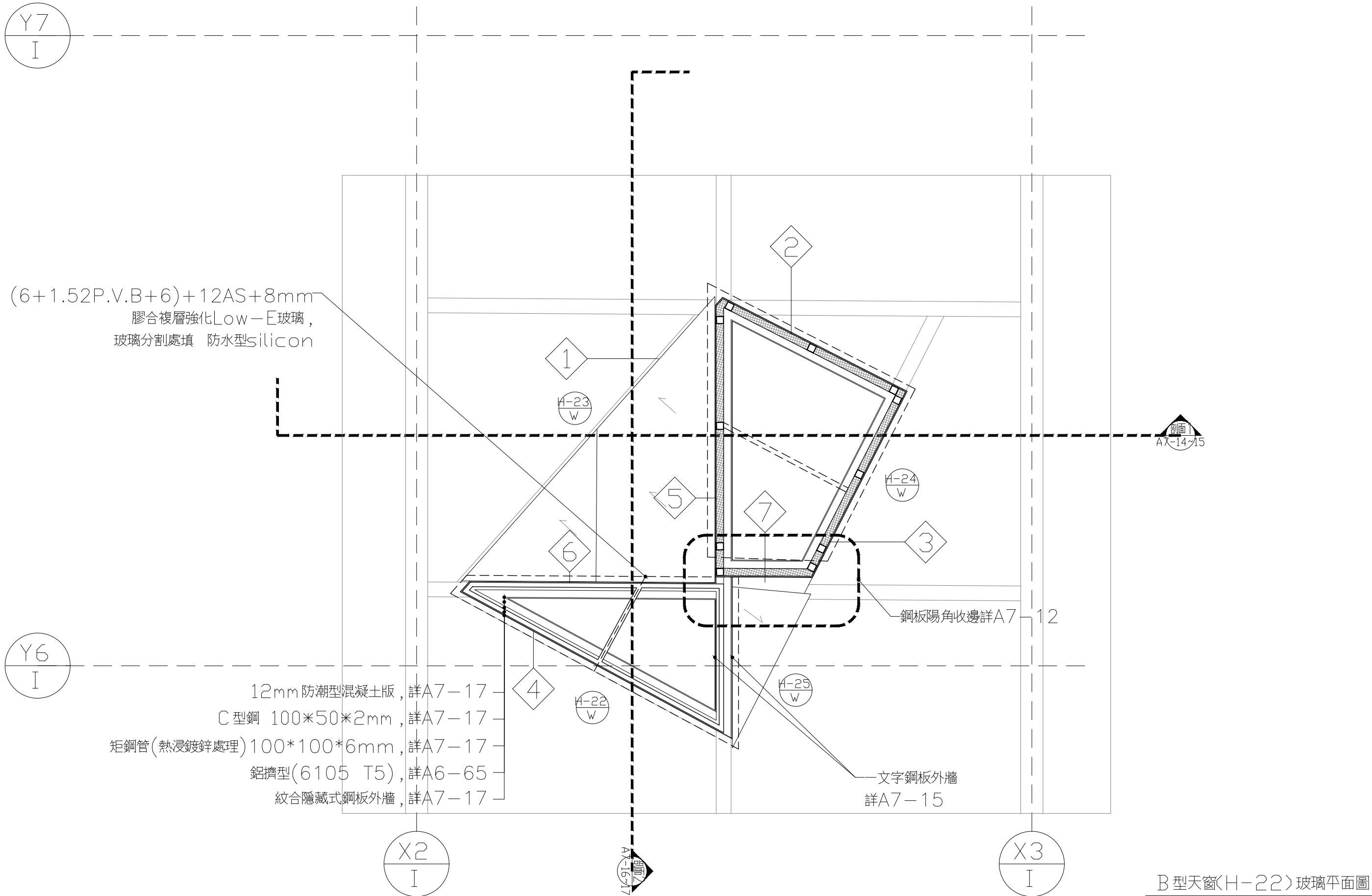
B 型天窗(H-22)玻璃平面圖
