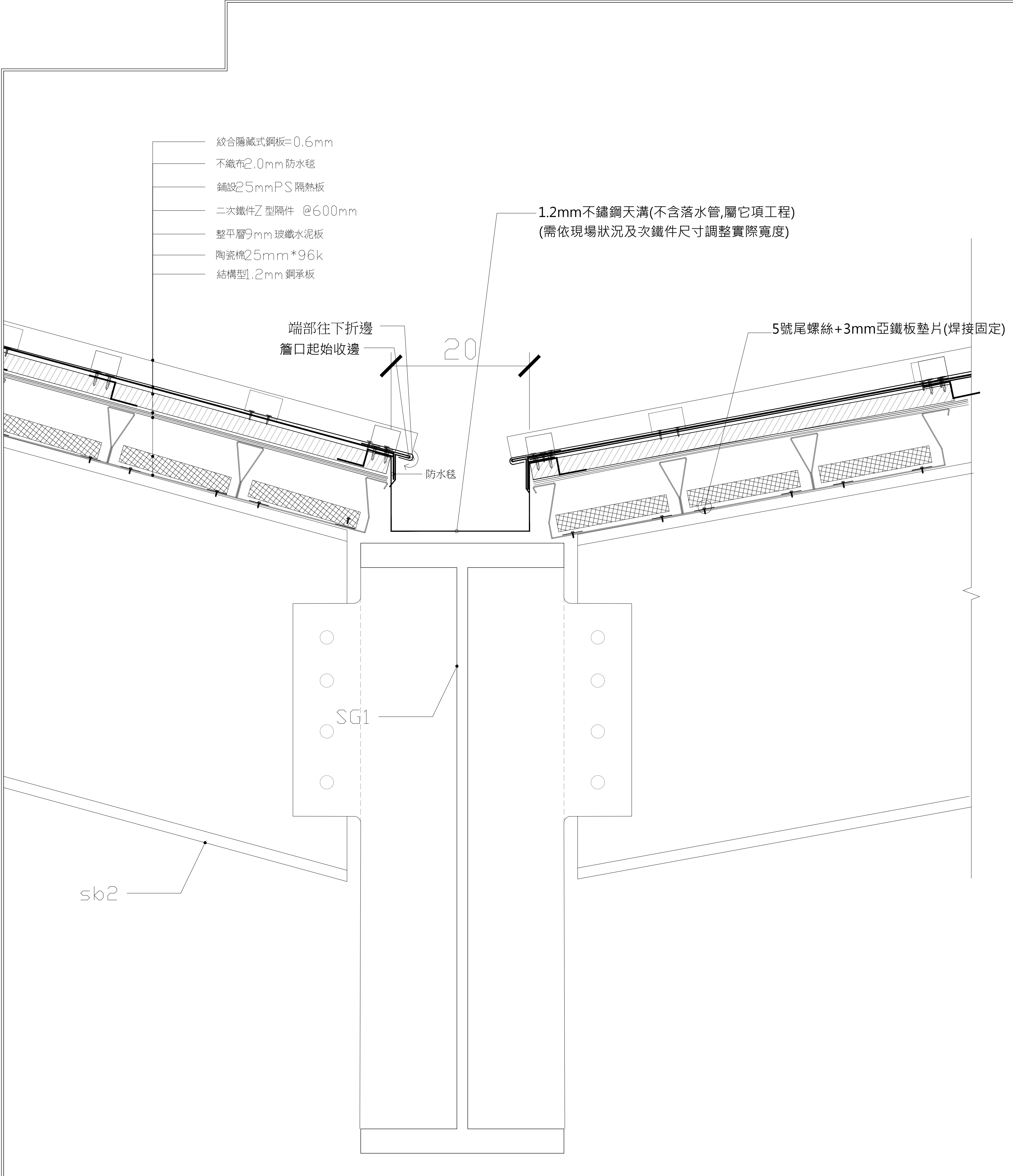
D 型截水溝剖面詳圖
