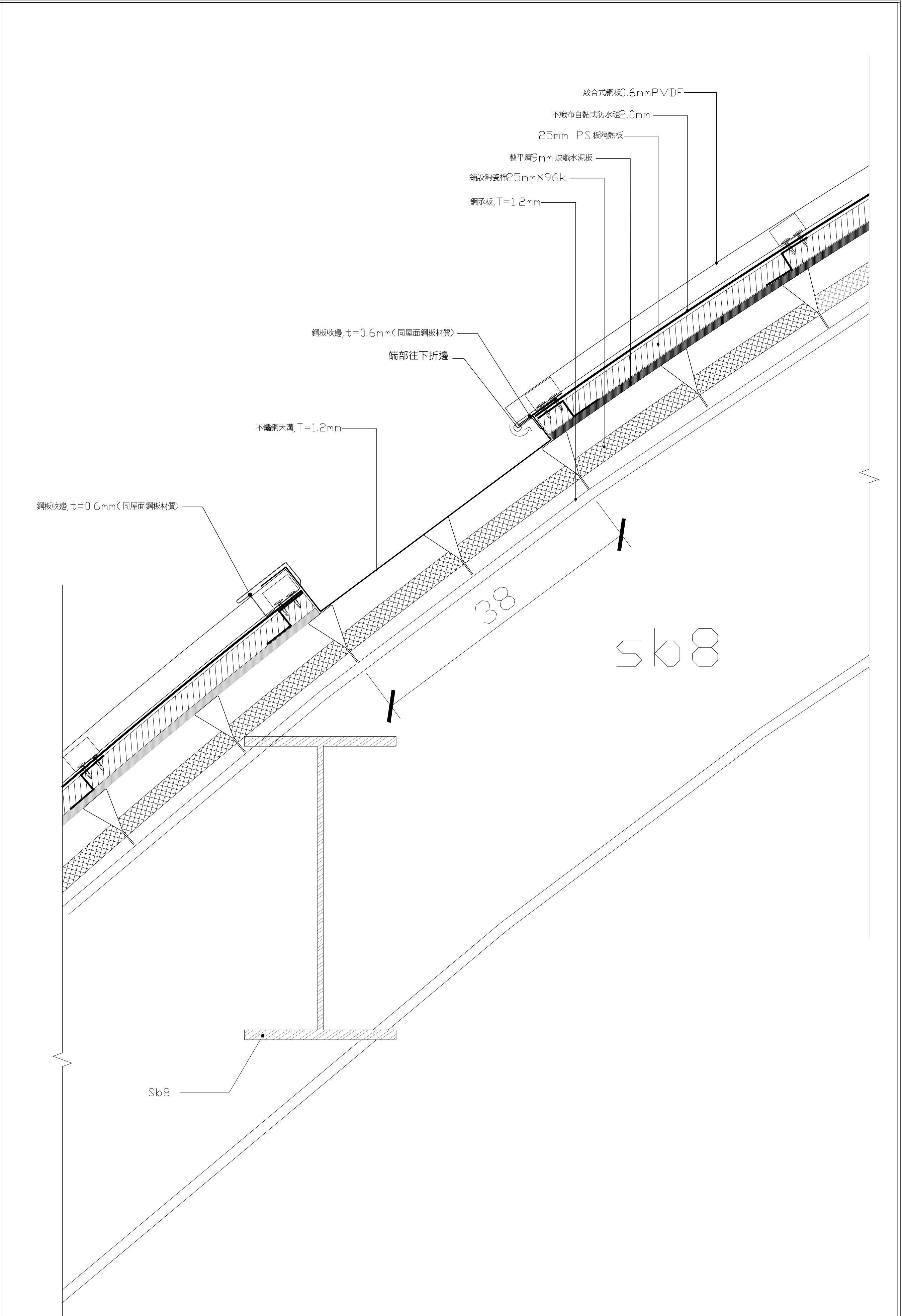
E 型截水溝剖面詳圖
