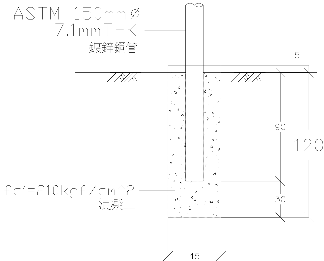
告示牌基礎圖 (單位:cm)
