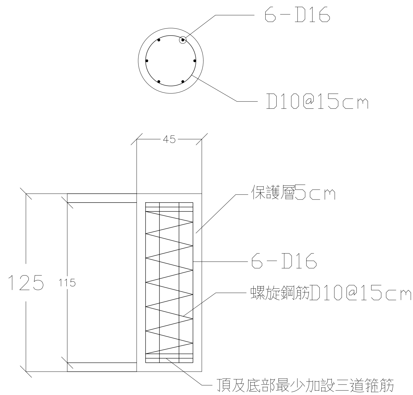
基礎詳圖 (單位:cm)
