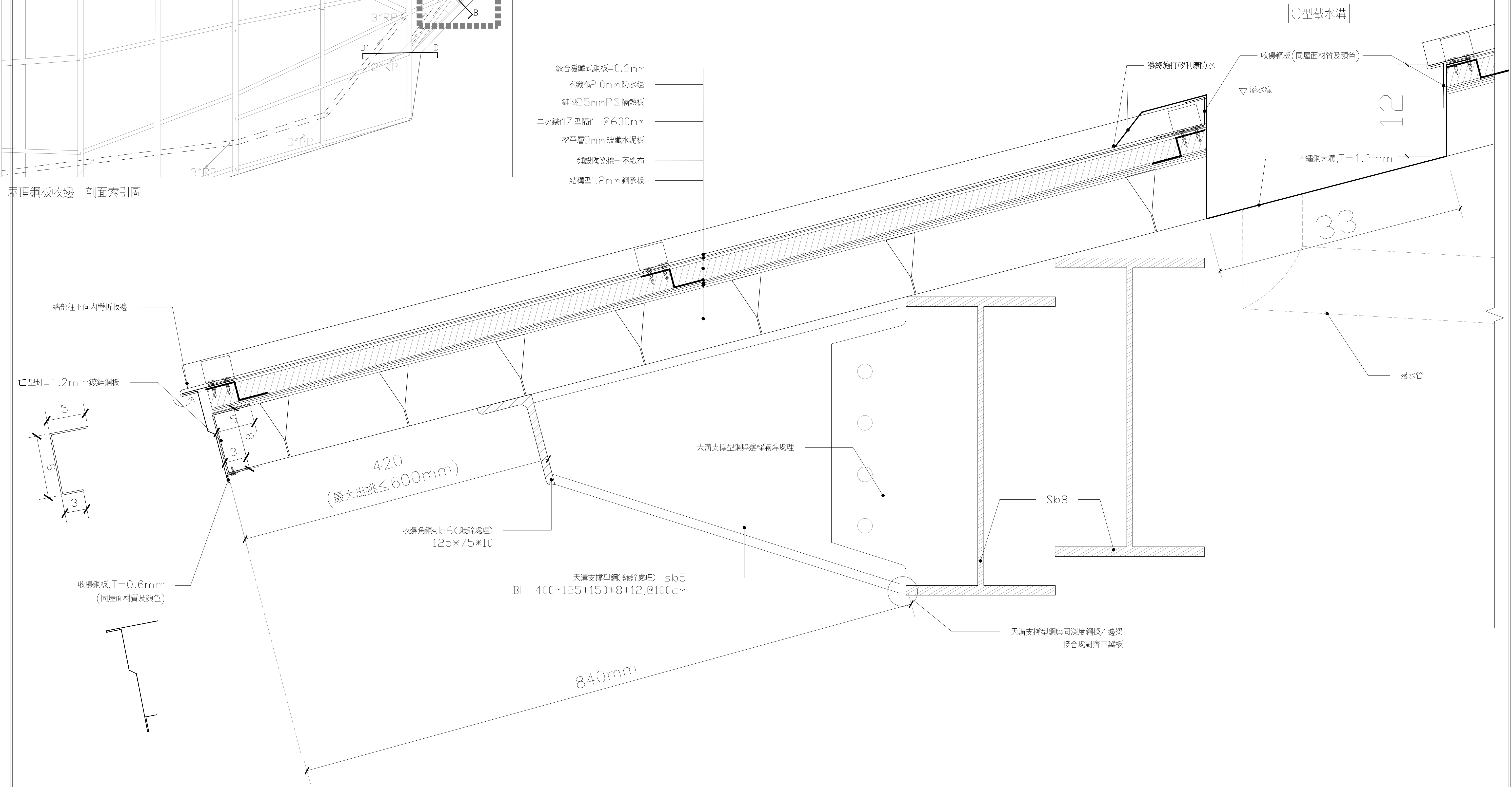
BH出挑收邊 B-B'剖面詳圖
