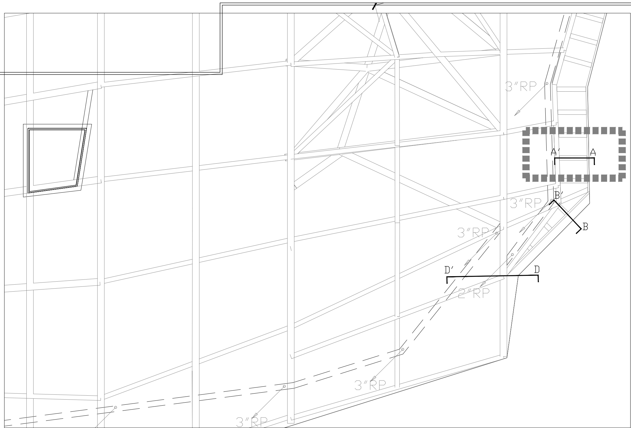
屋頂鋼板收邊 剖面索引圖
