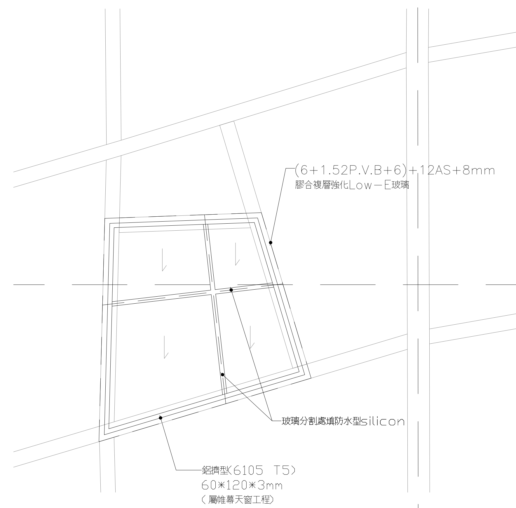
玻璃平面圖
