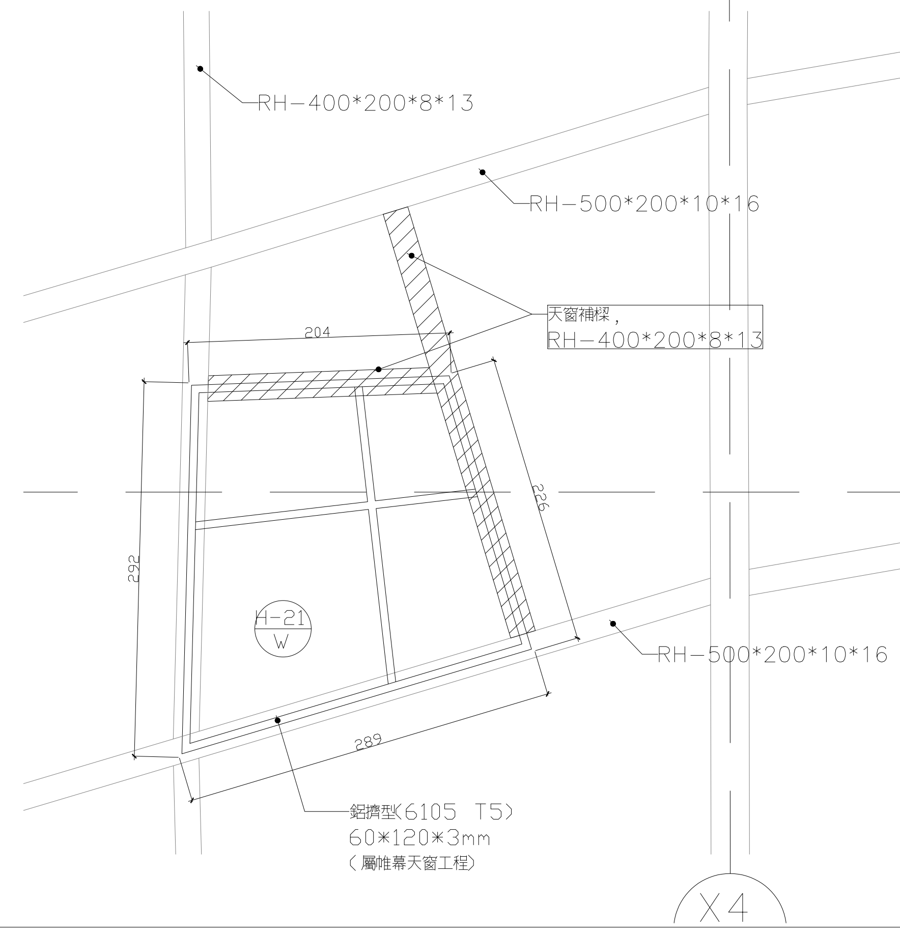
A 型天窗-2
