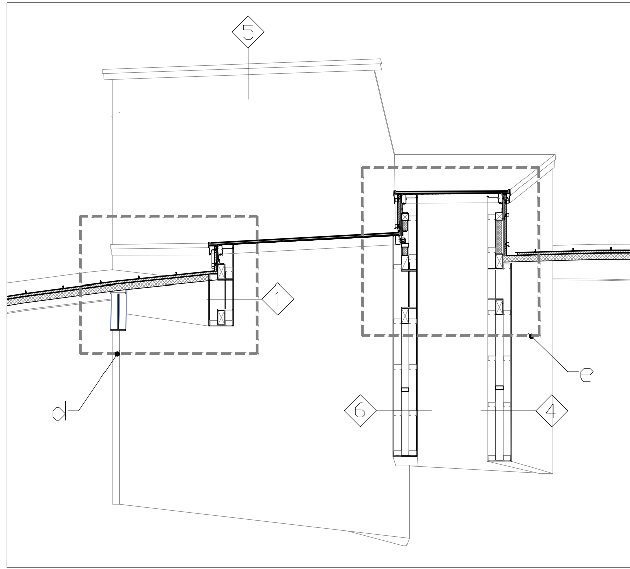
B 型天窗 剖面2－細部索引圖
