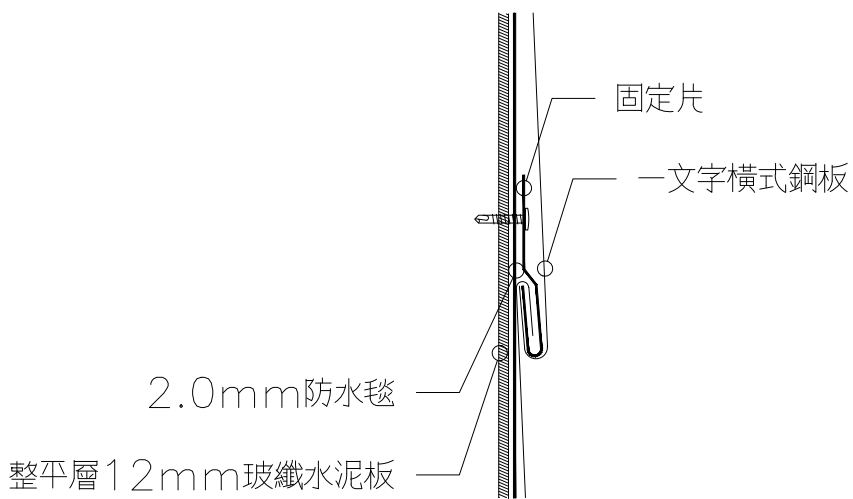
剖面固定詳圖
