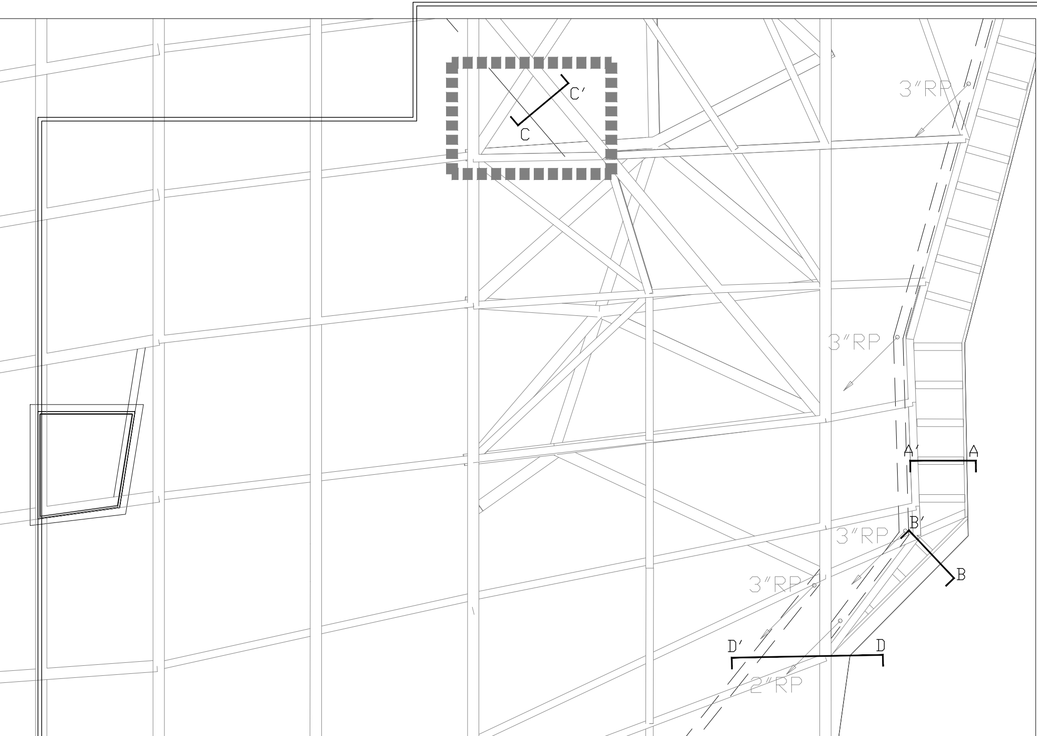
屋頂銅板收邊 剖面索引圖
