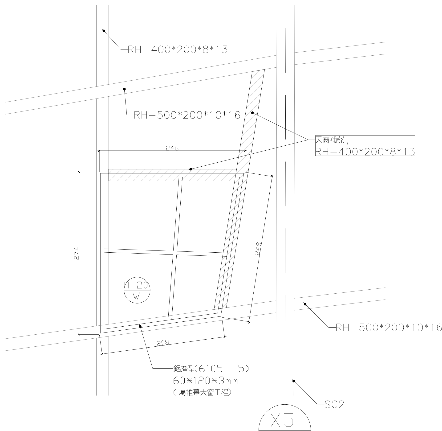
A 型天窗-1
