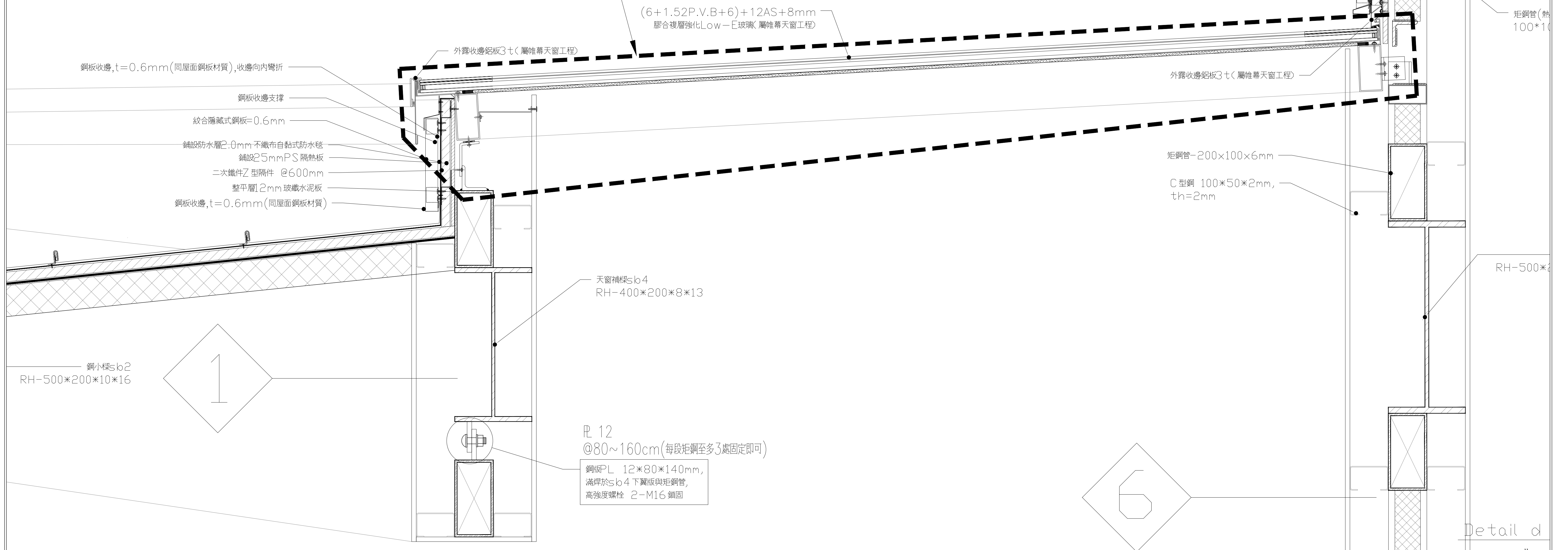
B 型天窗 剖面2－細部詳圖
