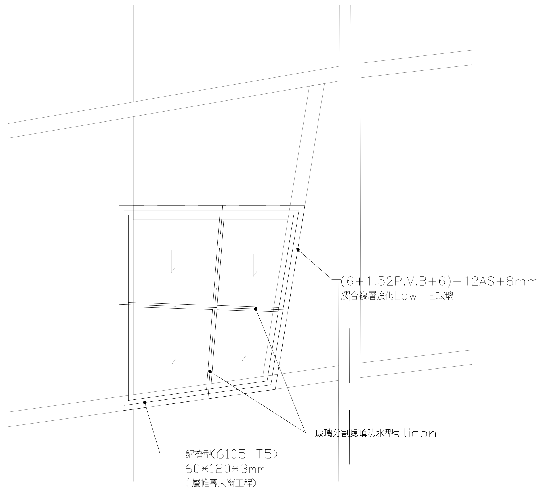
玻璃平面圖
