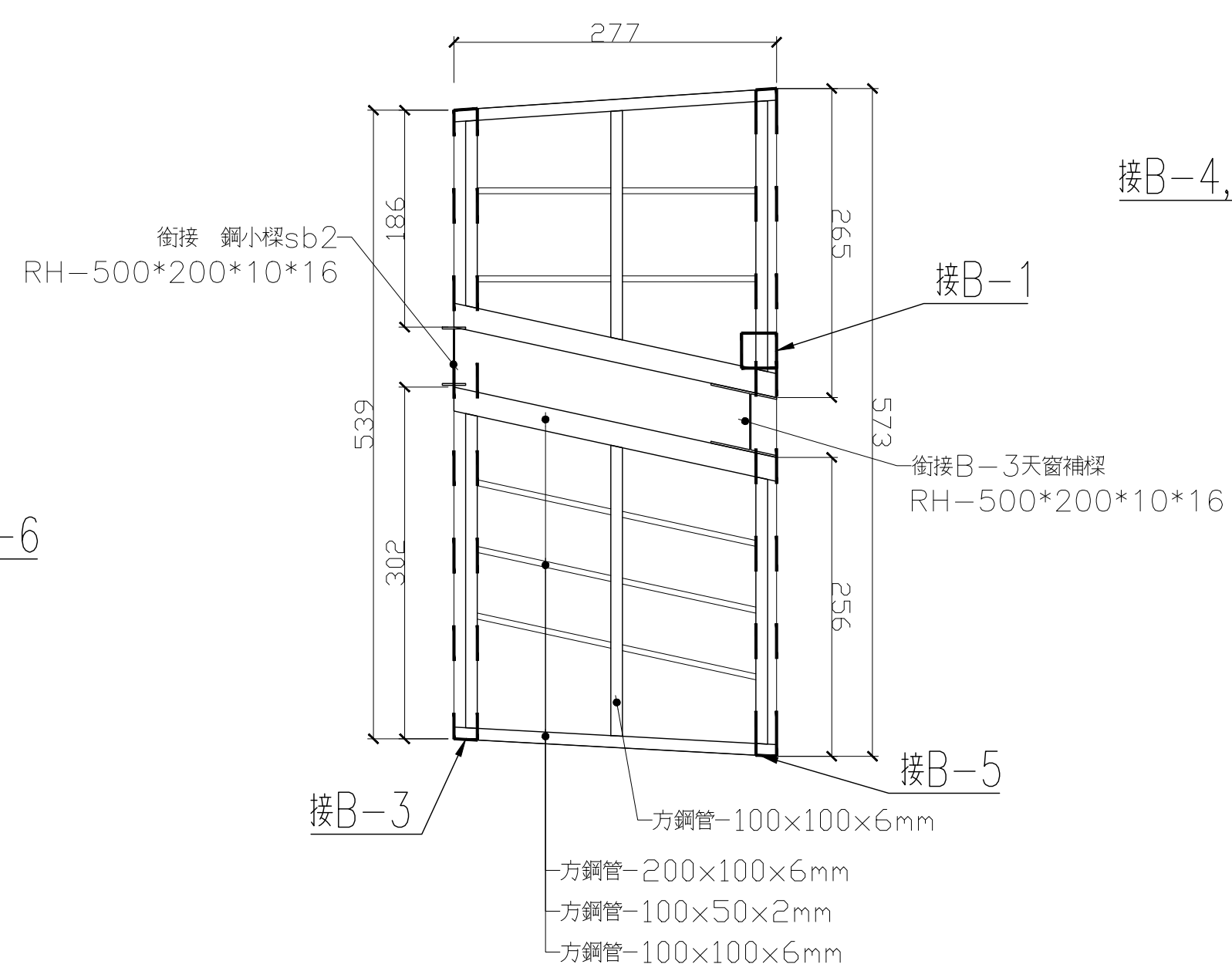
◈ B-2 ( 室外絞合隱藏式鋼板, 12mm 防潮型混凝土版 )
