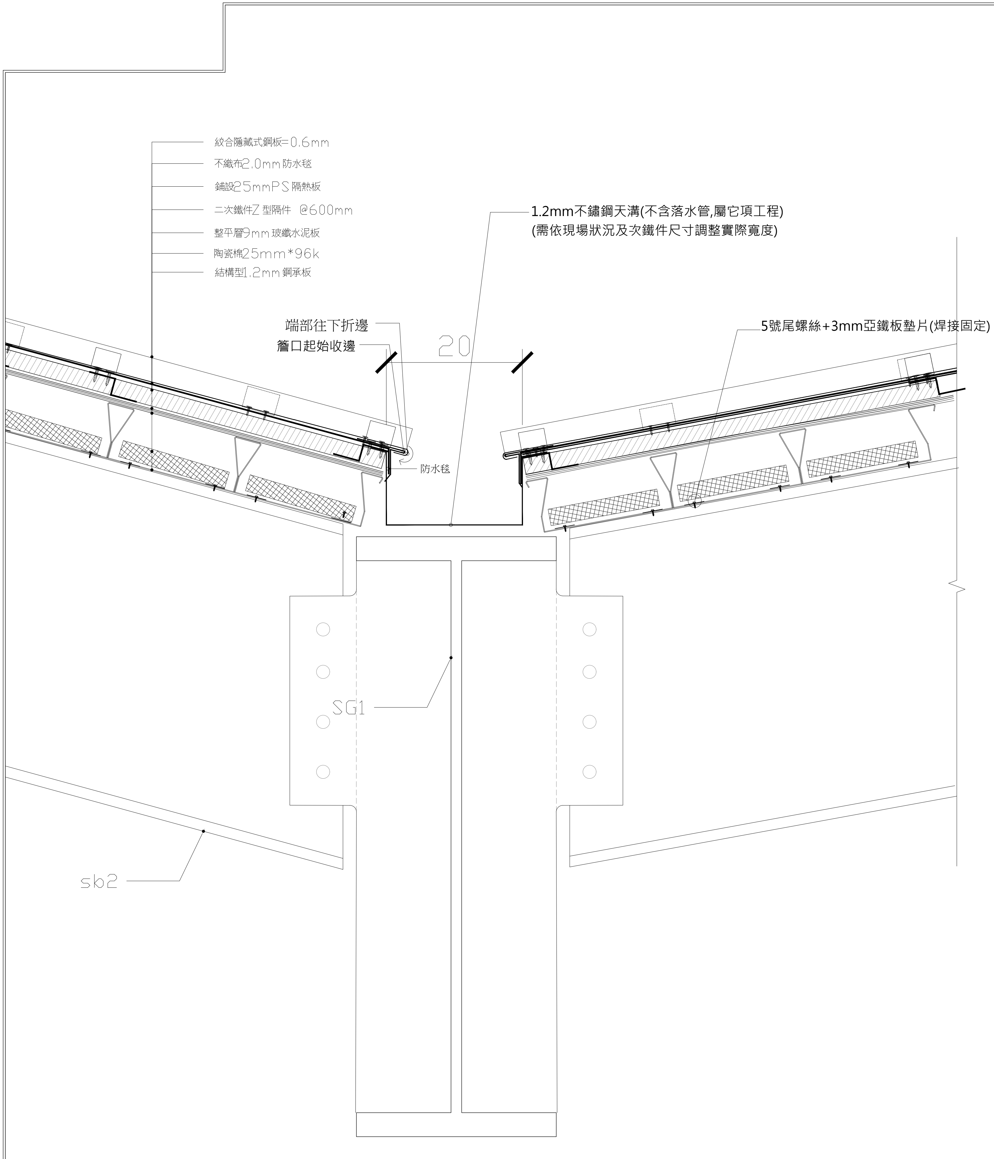
D 型排水溝剖面詳圖
