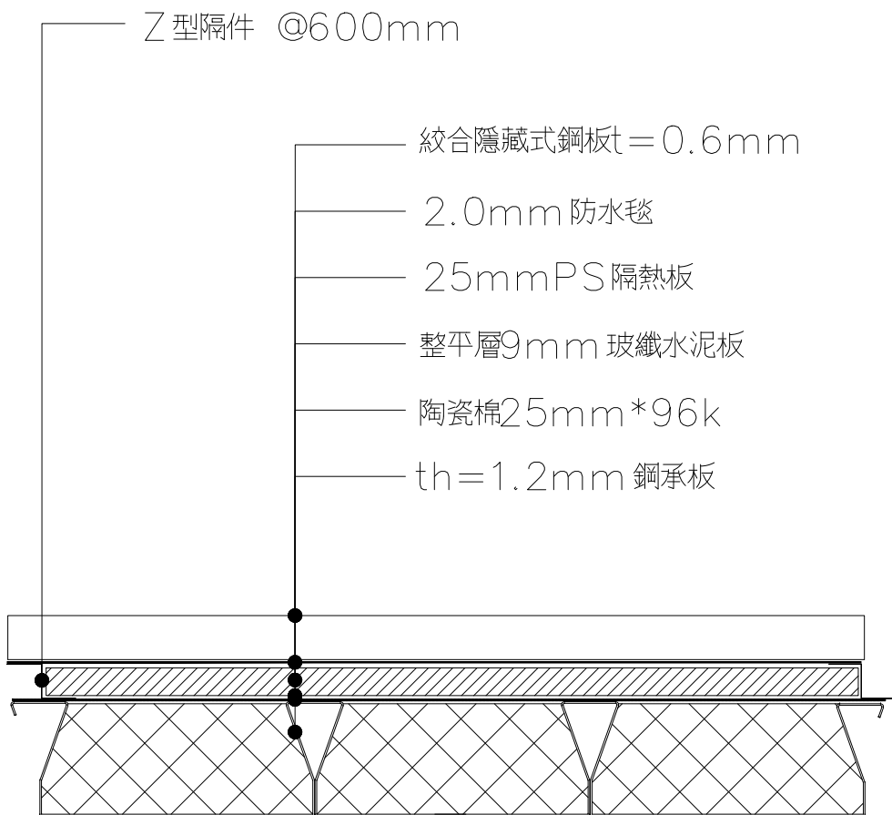
縱向剖面詳圖
