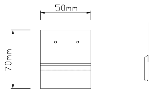
隱藏式固定扣件大樣
