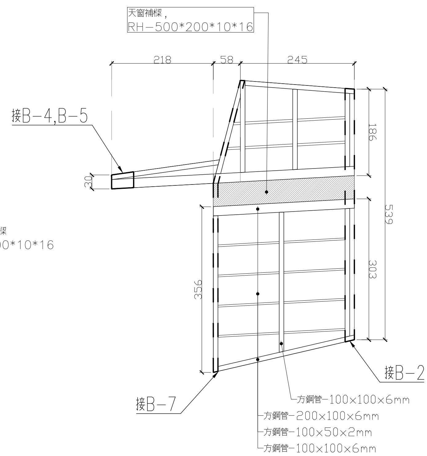
◈ B-3 ( 室外絞合隱藏式鋼板, 12mm 防潮型混凝土版 )
