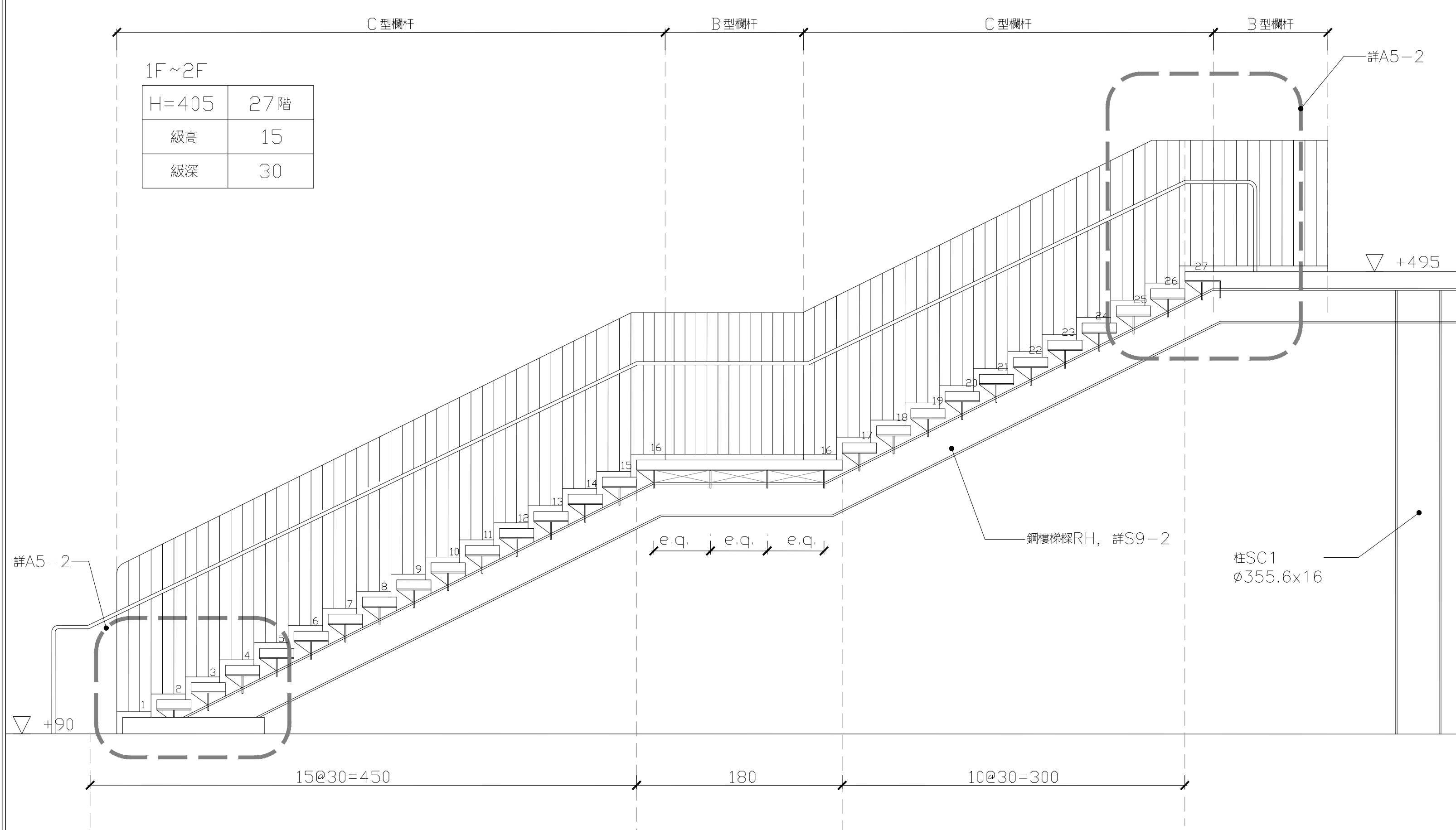
② 樓梯 L 剖面圖
