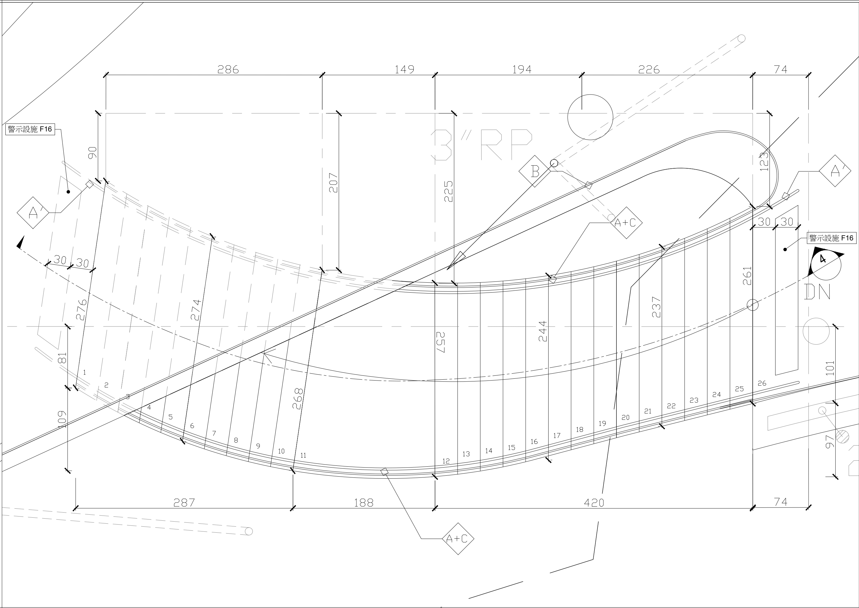
③ 樓梯 M 平面圖
