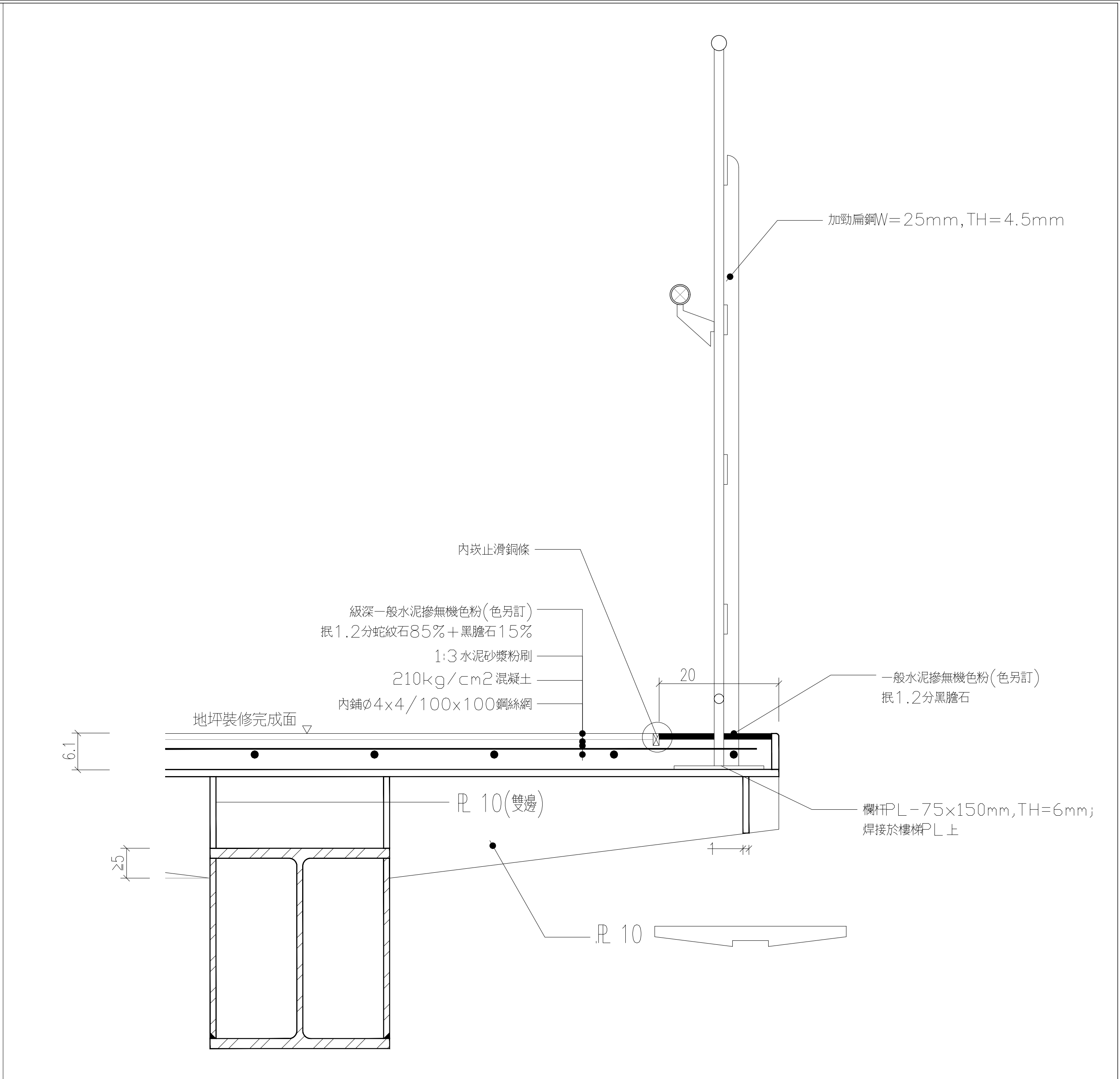
② 鋼樓梯踏接與欄杆C 細部詳圖
