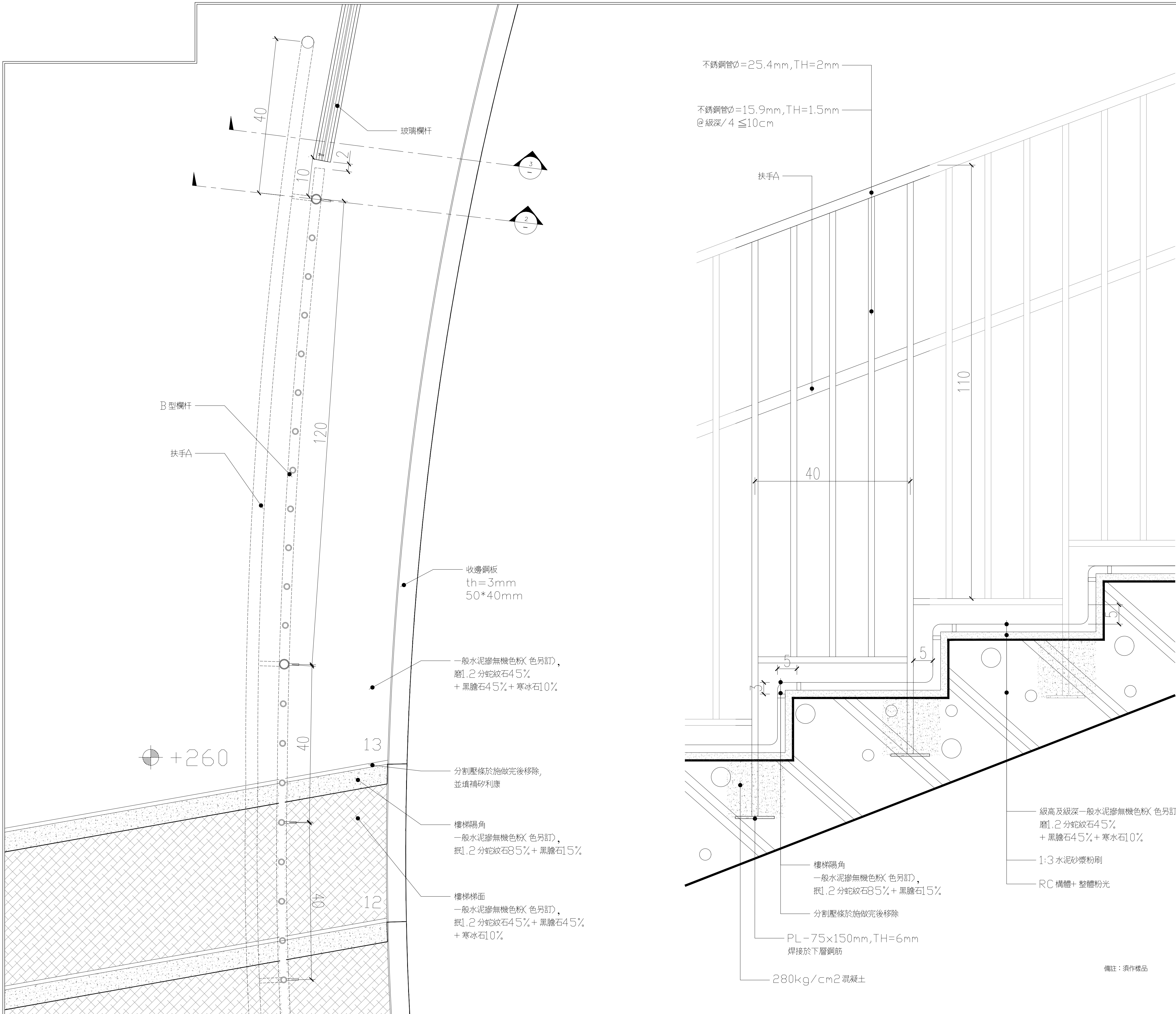
① 樓梯 N 細部詳圖-1
