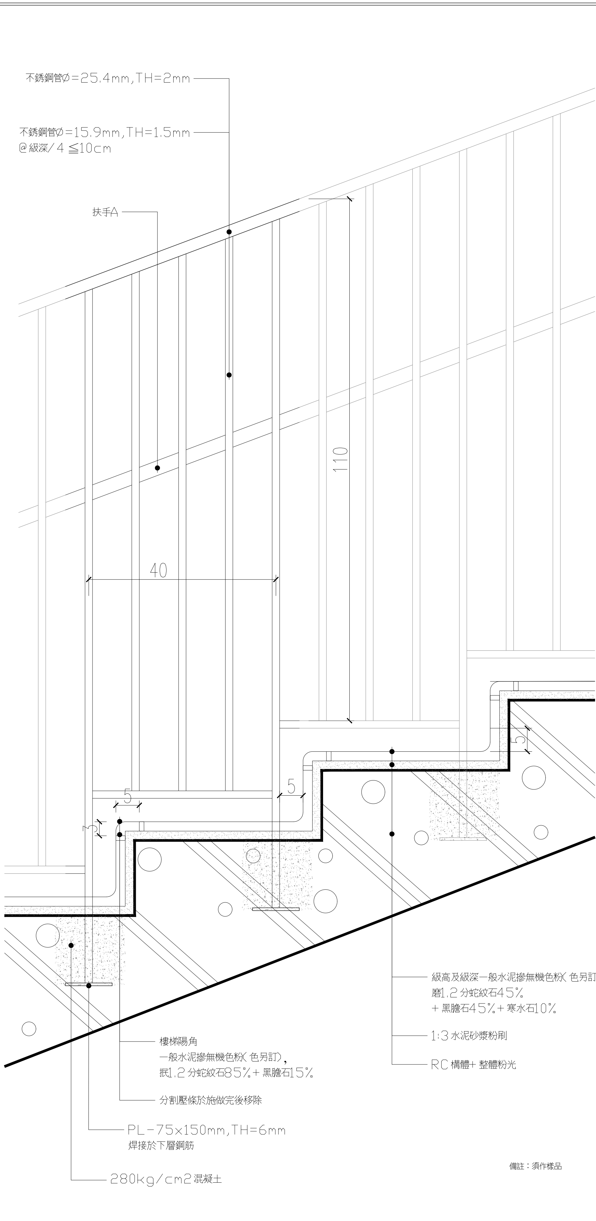
② 樓梯 N 細部詳圖-2
