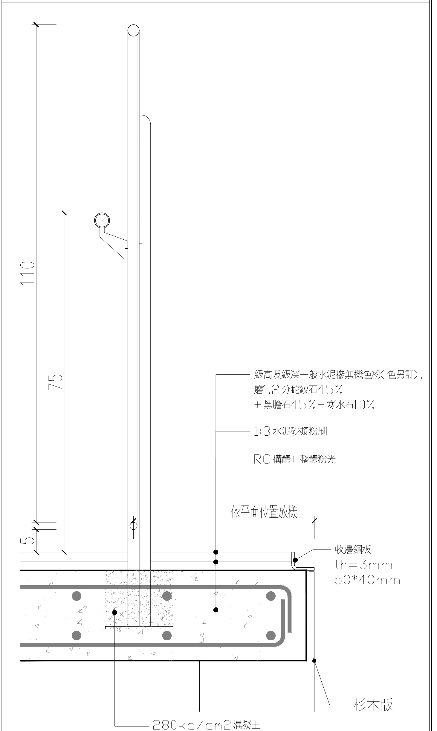
④ 樓梯 N 細部詳圖-3
