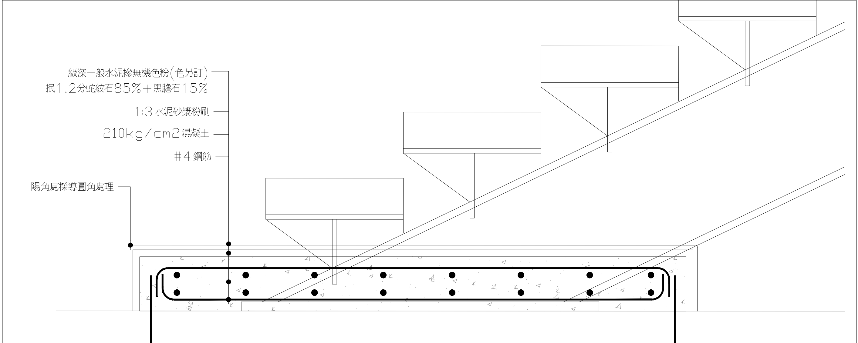
③ 鋼樓梯地面層踏階細部詳圖
