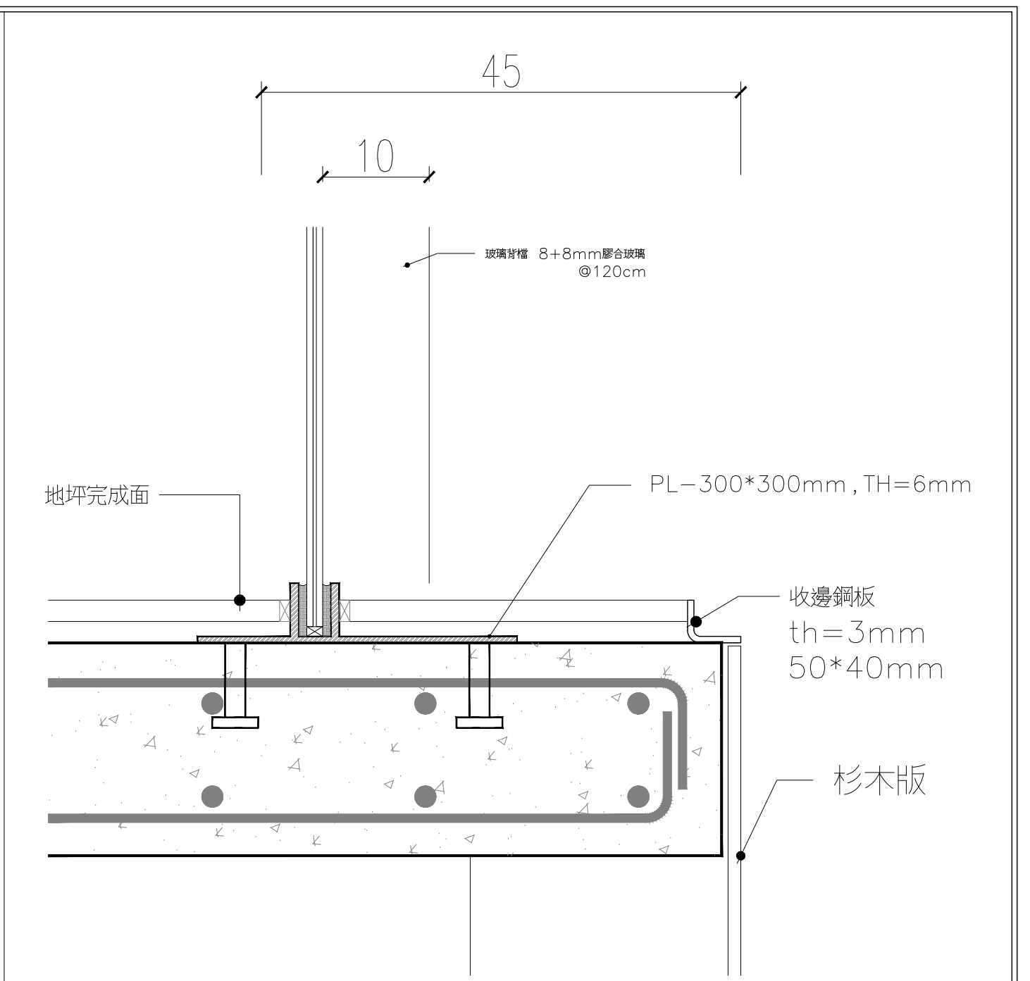
③ 樓梯 N 細部詳圖-3
