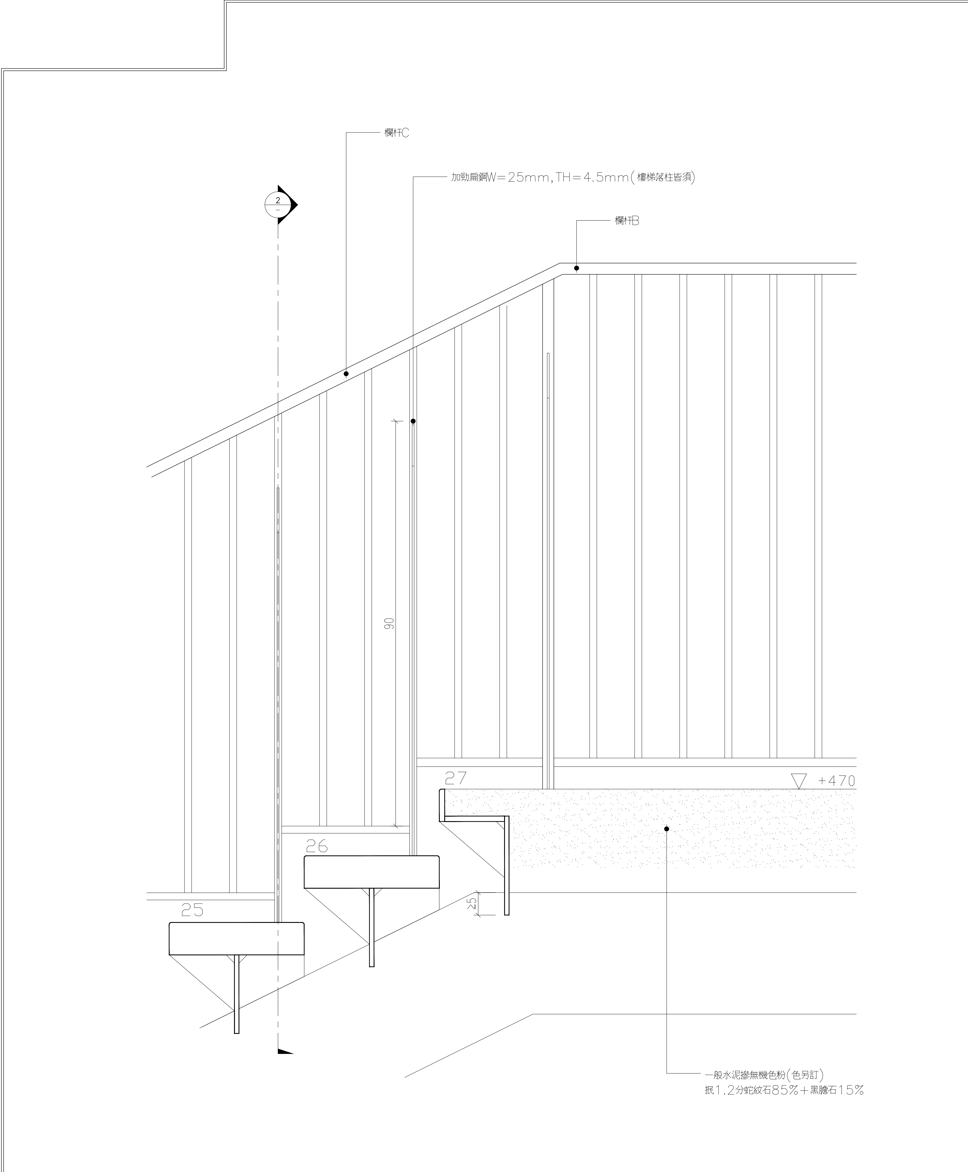
① 鋼樓梯細部詳圖
