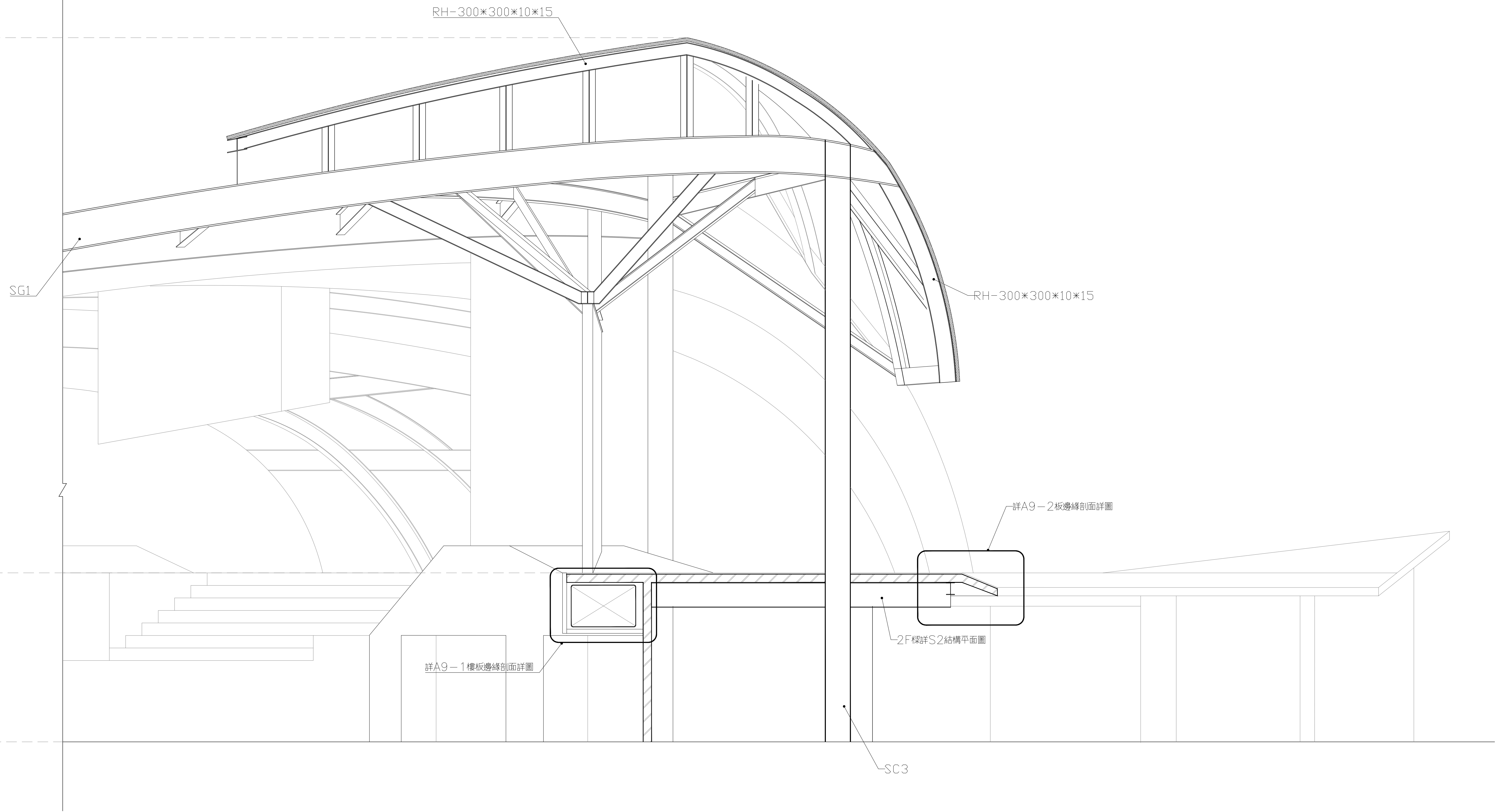
03 H棟X3 構架局部剖面 S:1/50
