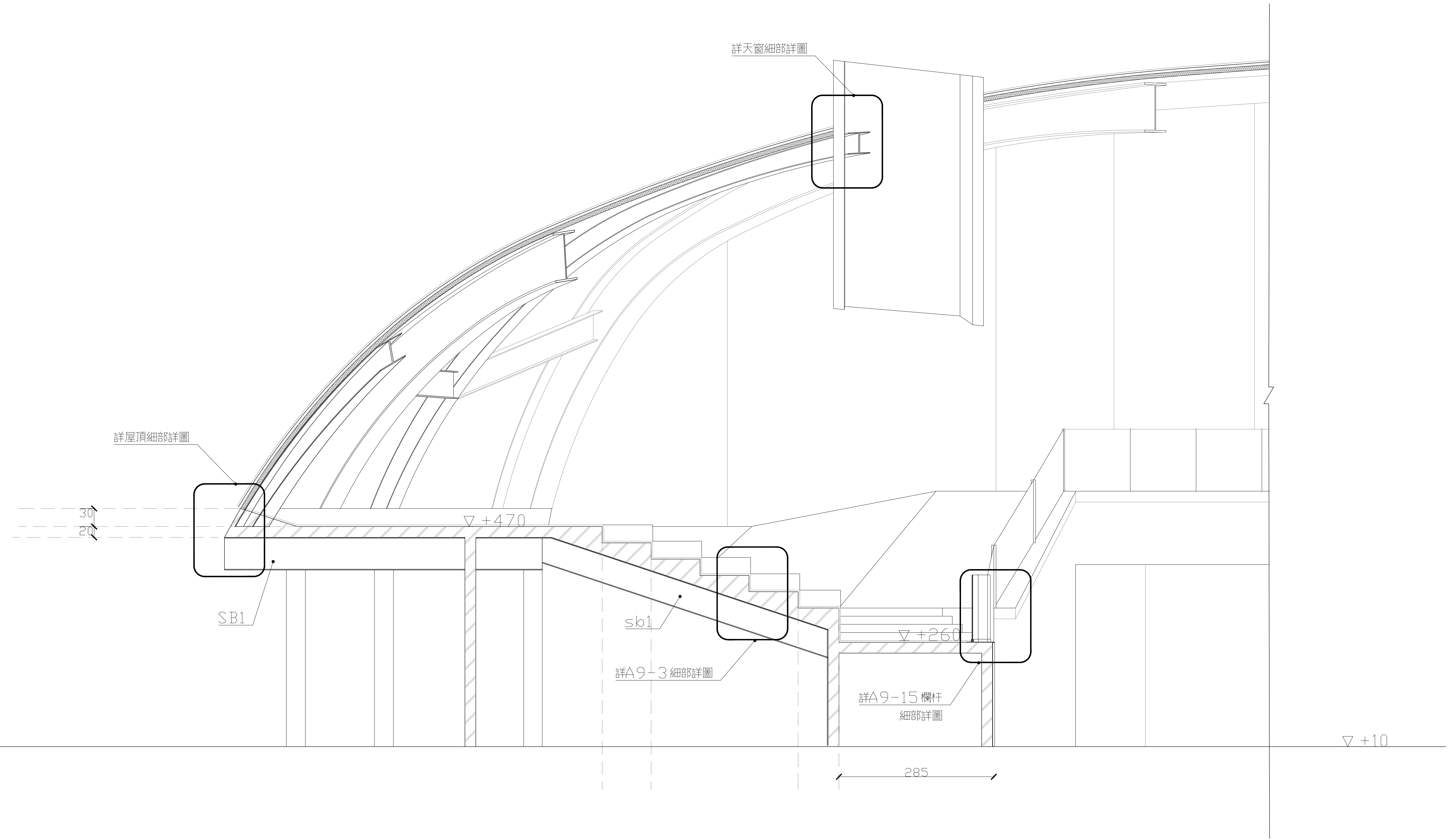
04 H棟局部剖面 S:1/50
