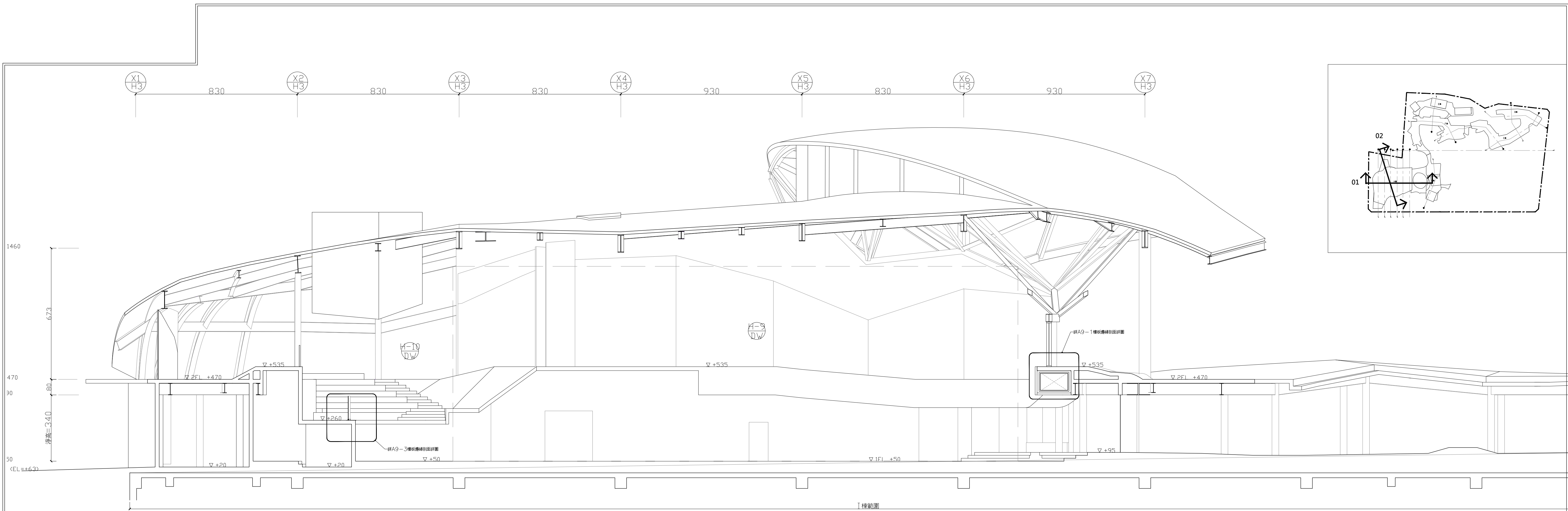
01 H棟長向剖面 S:1/100
