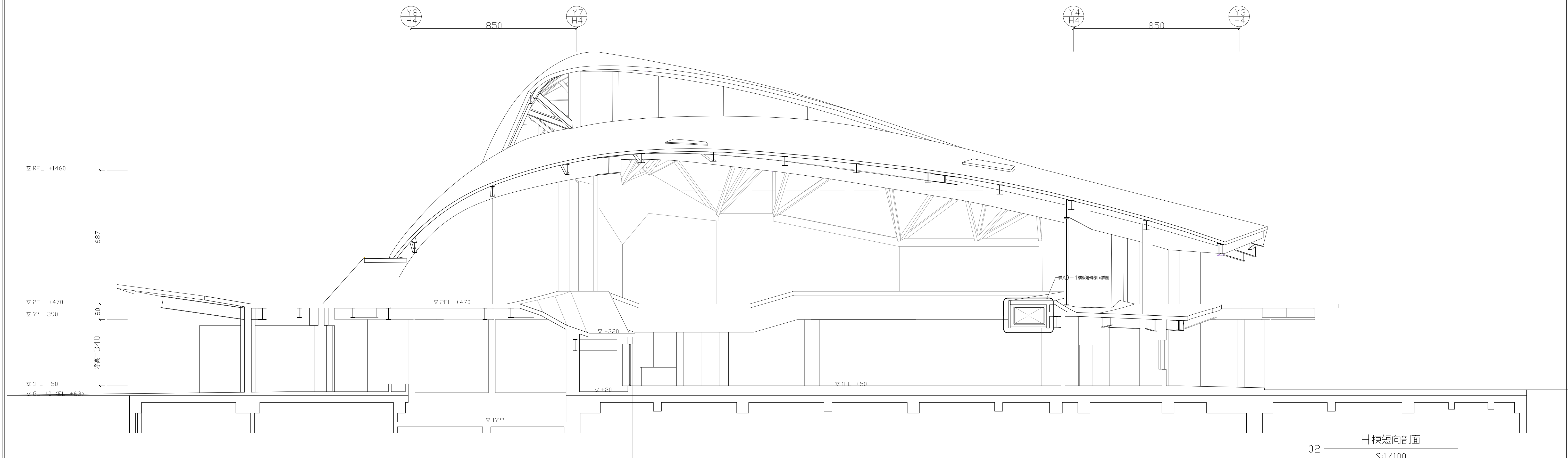
01 H棟長向剖面 S:1/100
