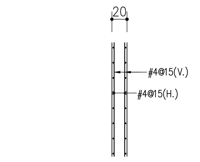
WT20剖面配筋圖 3 RC結構牆配筋剖面示意圖 (非結構牆配筋另詳圖S7-06)
