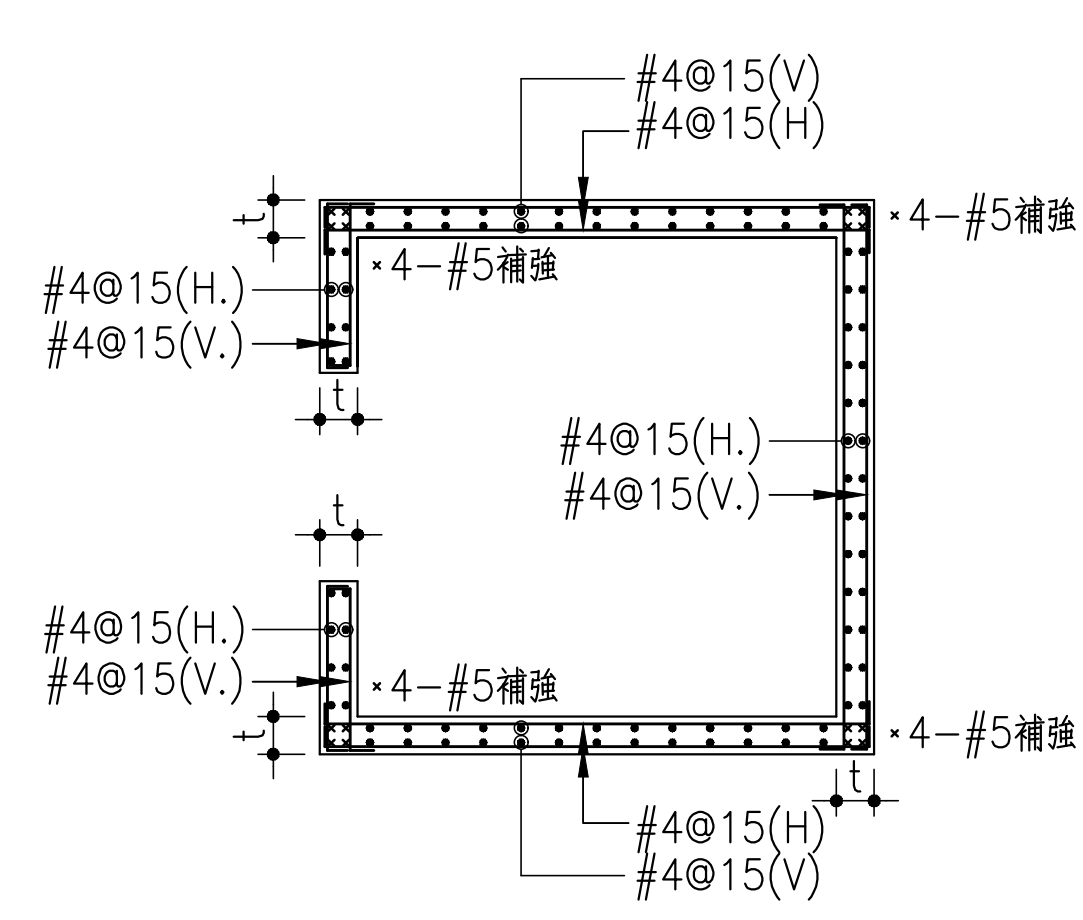
2 電梯牆配筋圖 註: "t" 詳平面厚度
