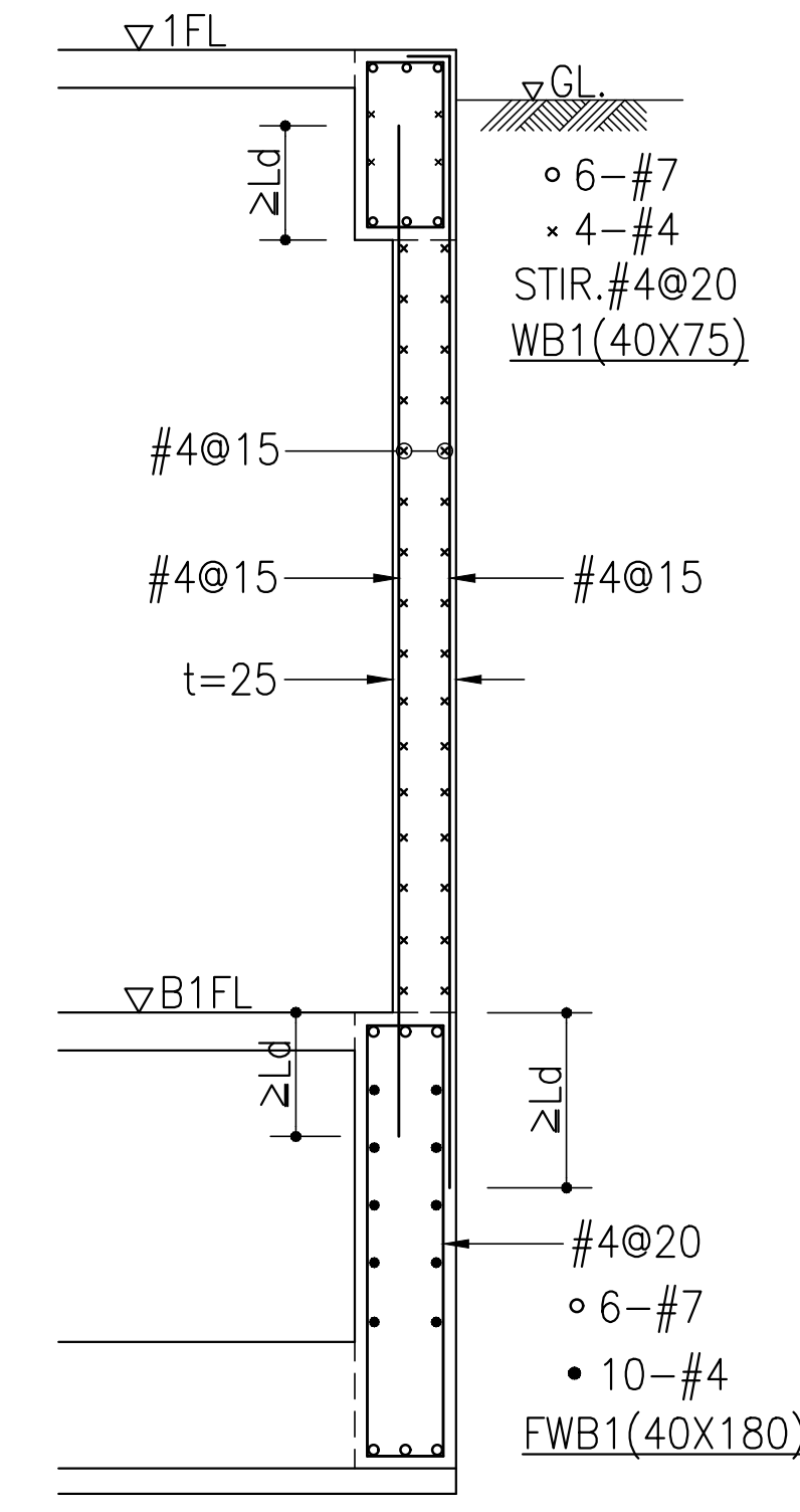
1 地下室外牆及邊梁配筋圖
