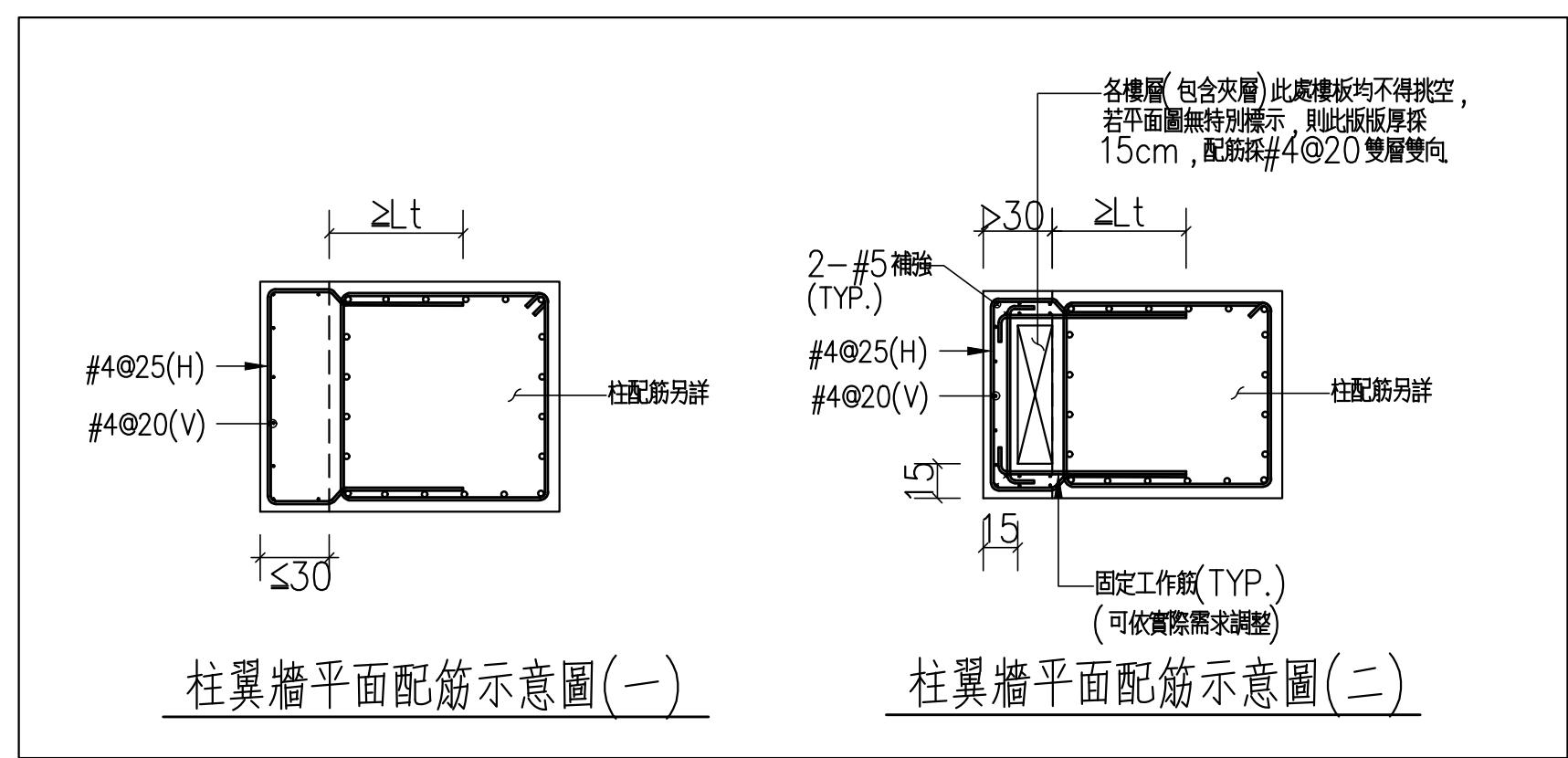
4 柱翼牆配筋示意圖
