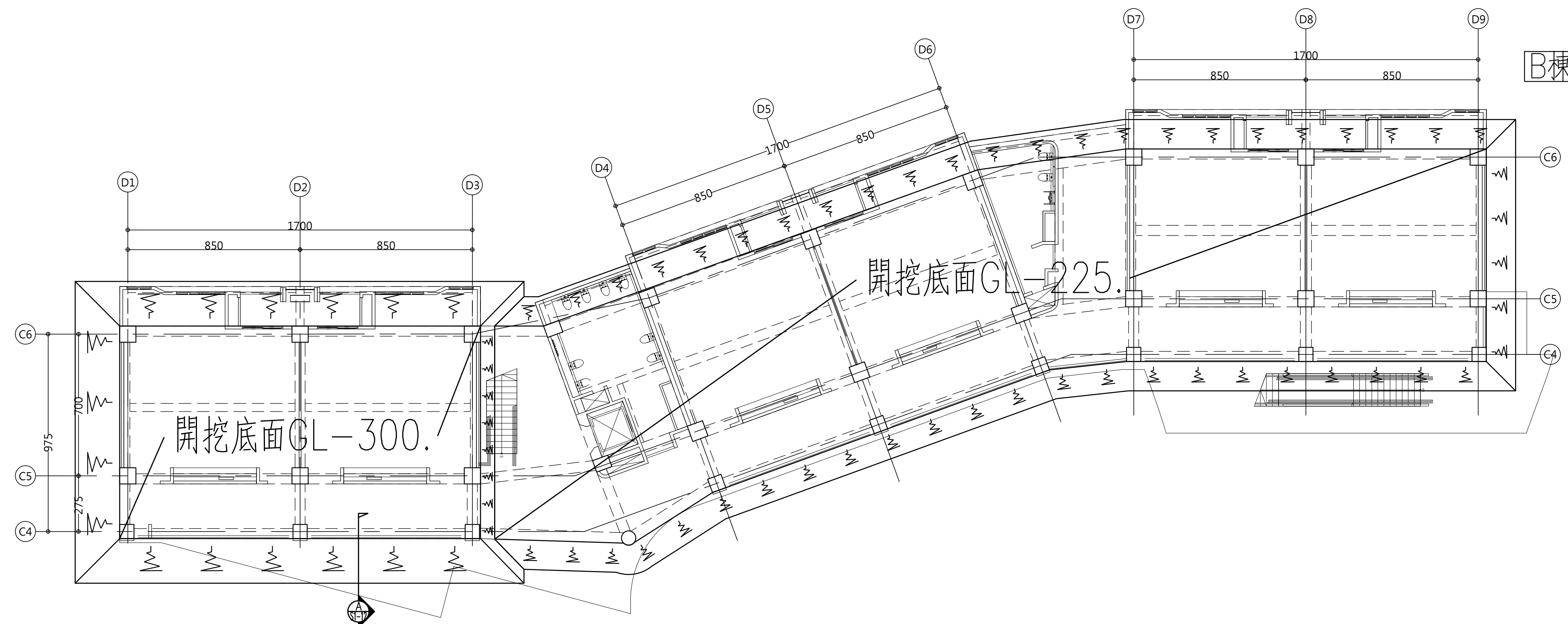
B棟 開挖擋土平面圖(二) A3:1/300 A1:1/150
