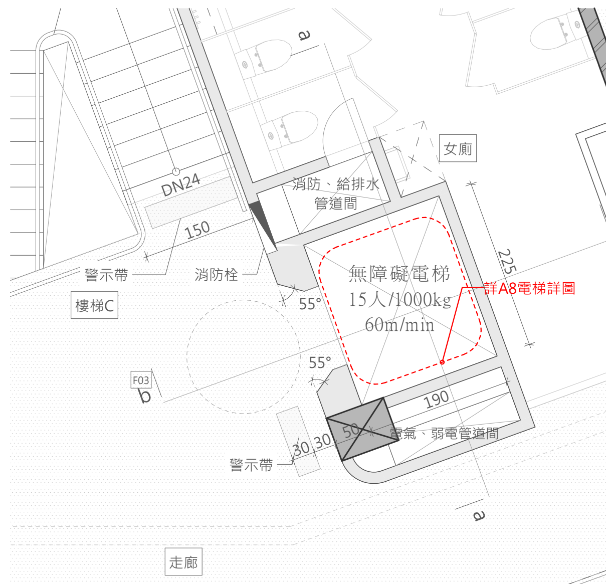
四樓電梯平面詳圖 A1SCALE=1/50 A3SCALE=1/100
