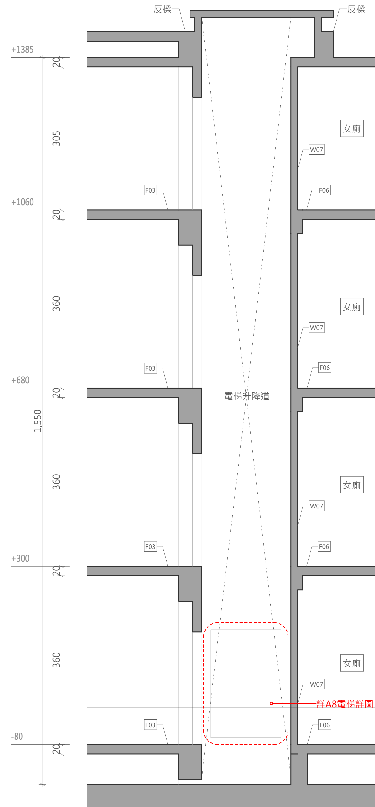
B棟電梯剖面詳圖a A1SCALE=1/50 A3SCALE=1/100
