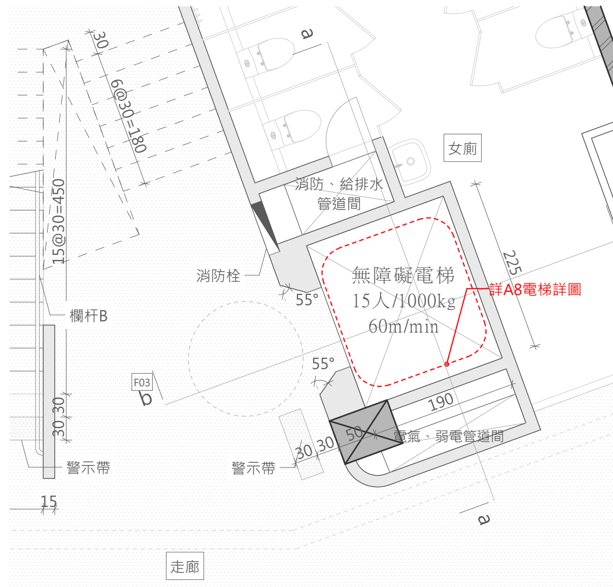
一樓電梯平面詳圖 A1SCALE=1/50 A3SCALE=1/100
