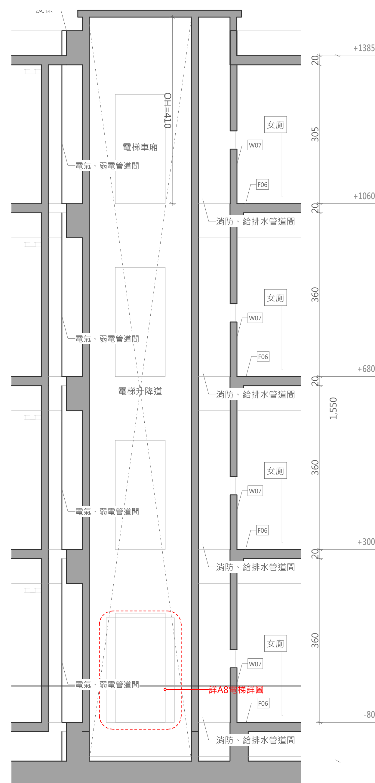
B棟電梯剖面詳圖b A1SCALE=1/50 A3SCALE=1/100
