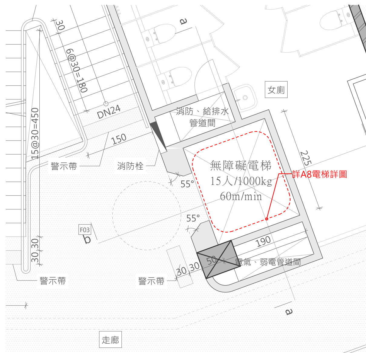
三樓電梯平面詳圖 A1SCALE=1/50 A3SCALE=1/100
