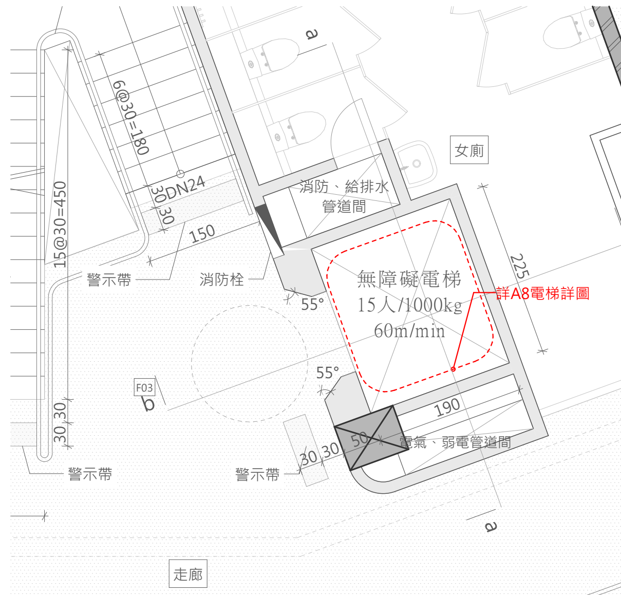
二樓電梯平面詳圖 A1SCALE=1/50 A3SCALE=1/100
