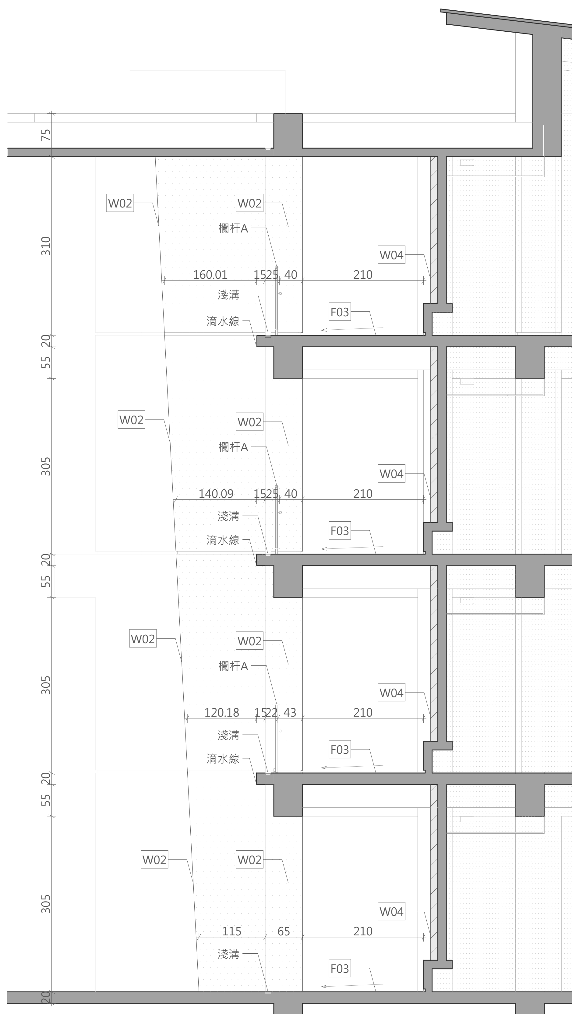
A棟 外牆剖面a A1SCALE=1/40 A3SCALE=1/80
