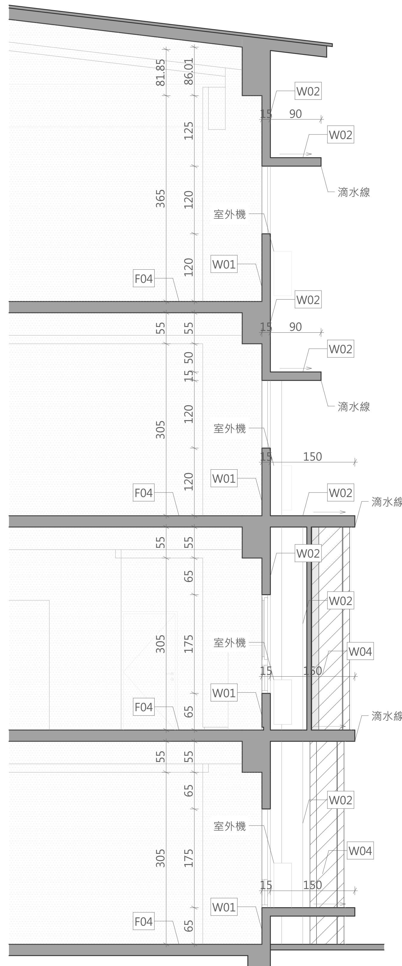
A棟 外牆剖面a A1SCALE=1/40 A3SCALE=1/80
