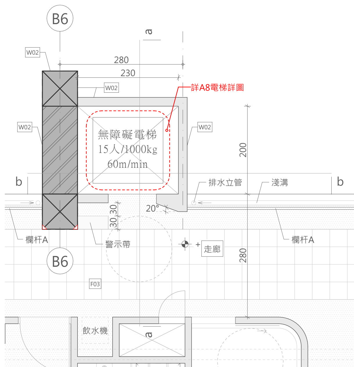
A棟四樓電梯平面詳圖 A1SCALE=1/50 A3SCALE=1/100
