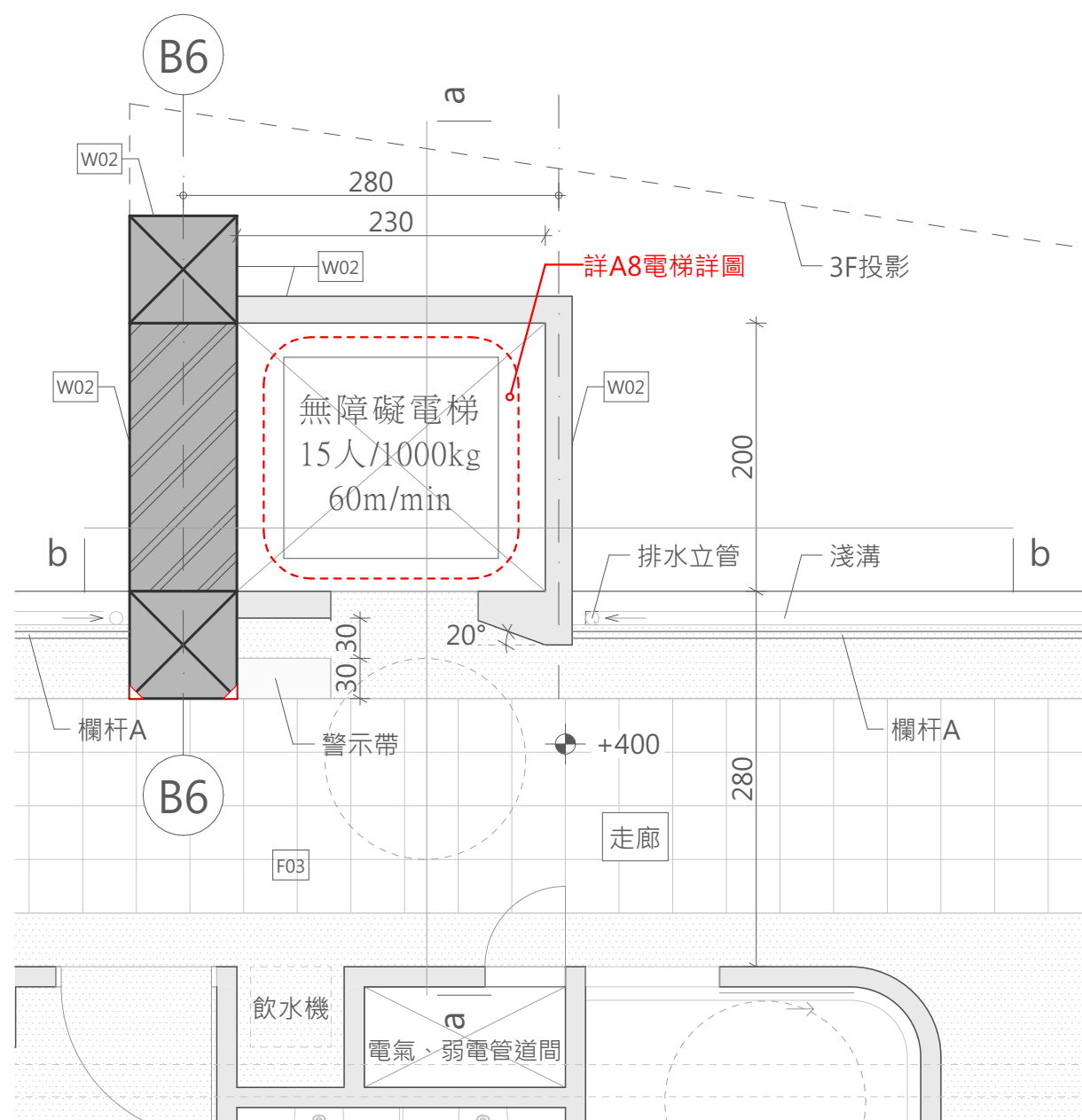
A棟二樓電梯平面詳圖 A1SCALE=1/50 A3SCALE=1/100
