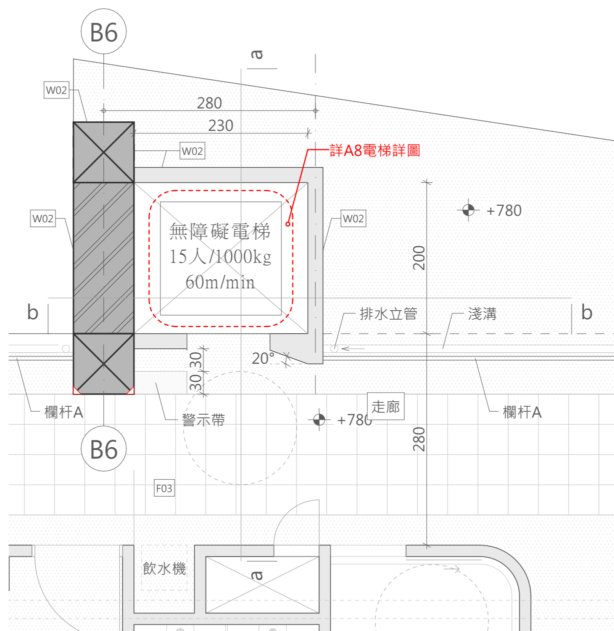
A棟三樓電梯平面詳圖 A1SCALE=1/50 A3SCALE=1/100
