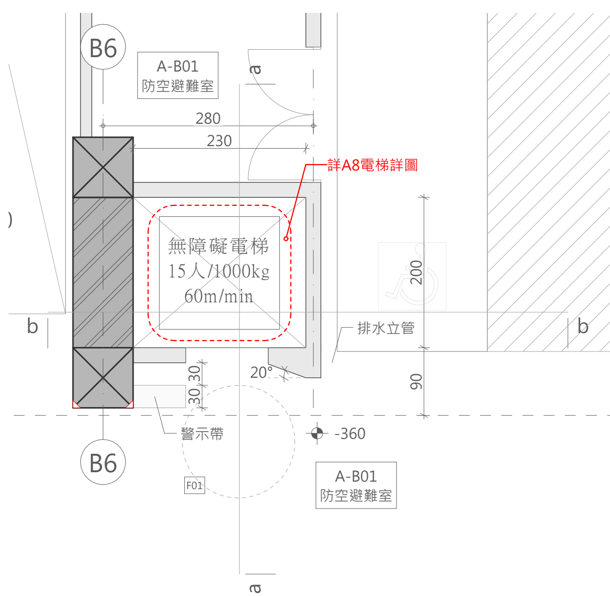
A棟一樓電梯平面詳圖 A1SCALE=1/50 A3SCALE=1/100
