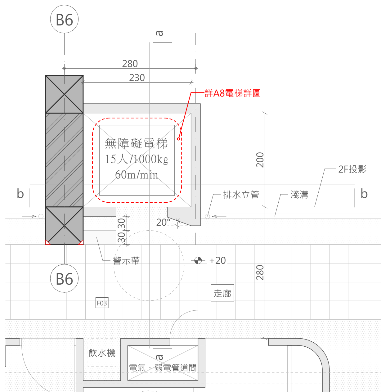
A棟一樓電梯平面詳圖 A1SCALE=1/50 A3SCALE=1/100
