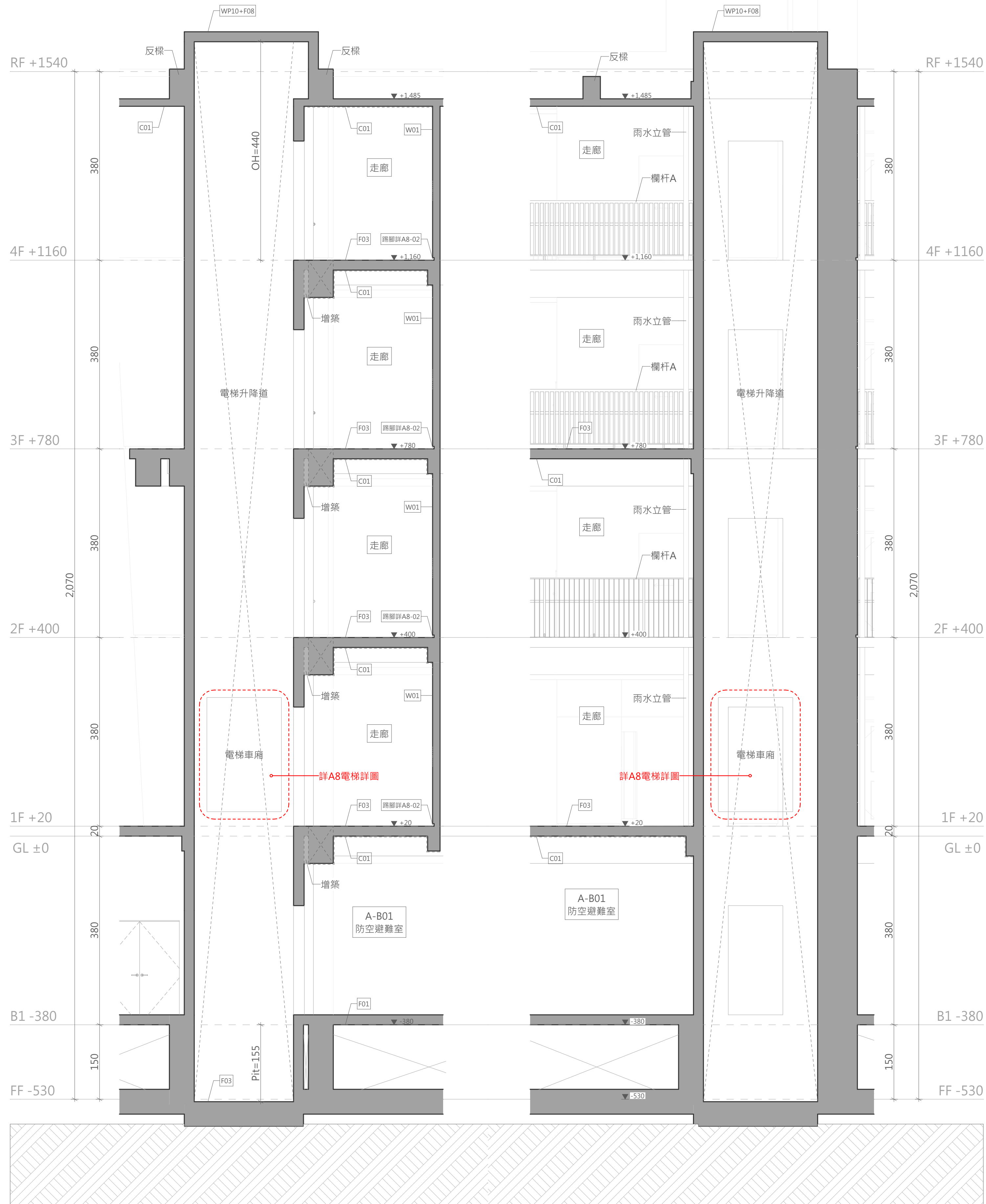
A棟電梯剖面詳圖a A1SCALE=1/50 A3SCALE=1/100
