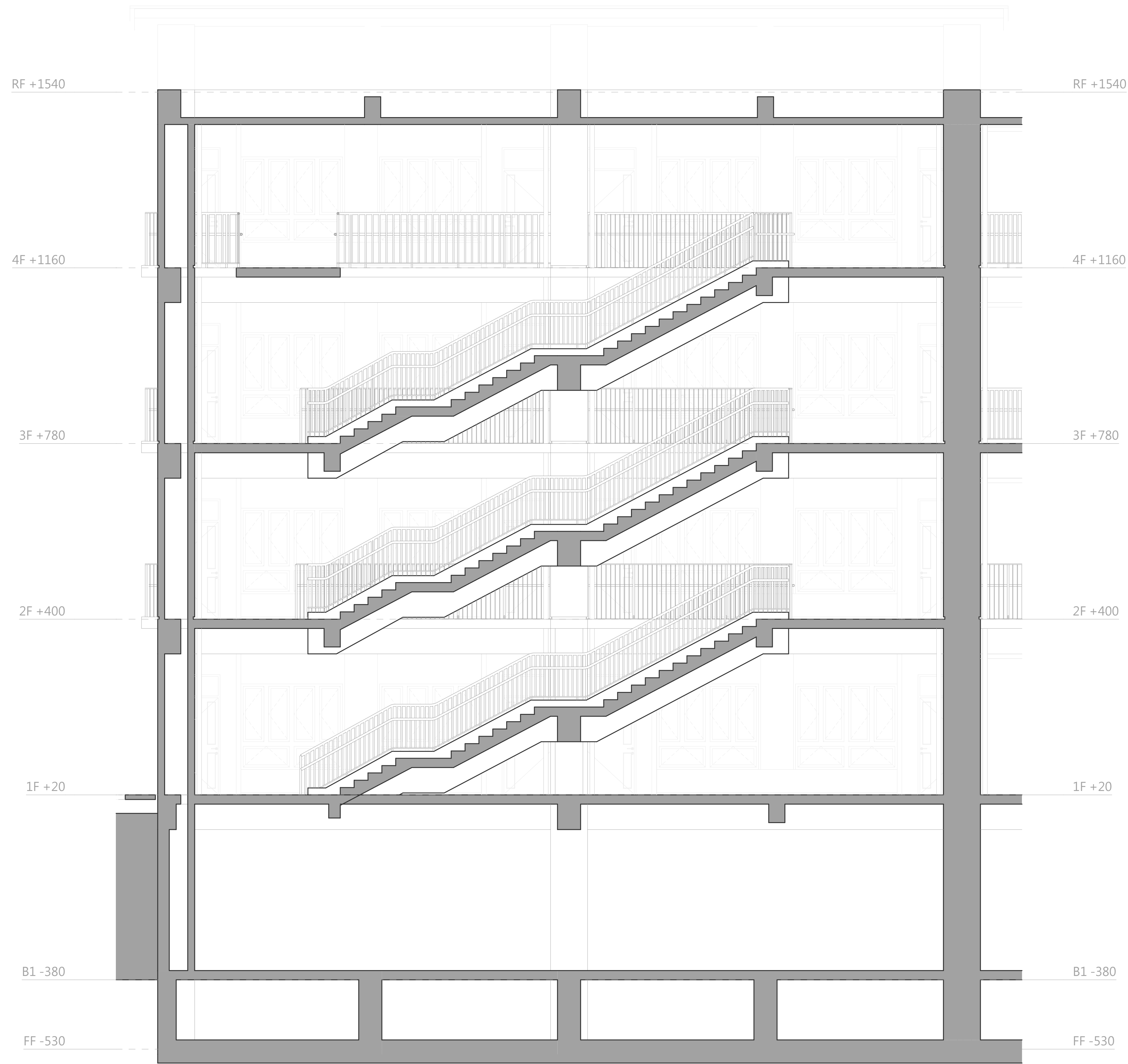
A棟B梯剖面詳圖a A1SCALE=1/50 A3SCALE=1/100
