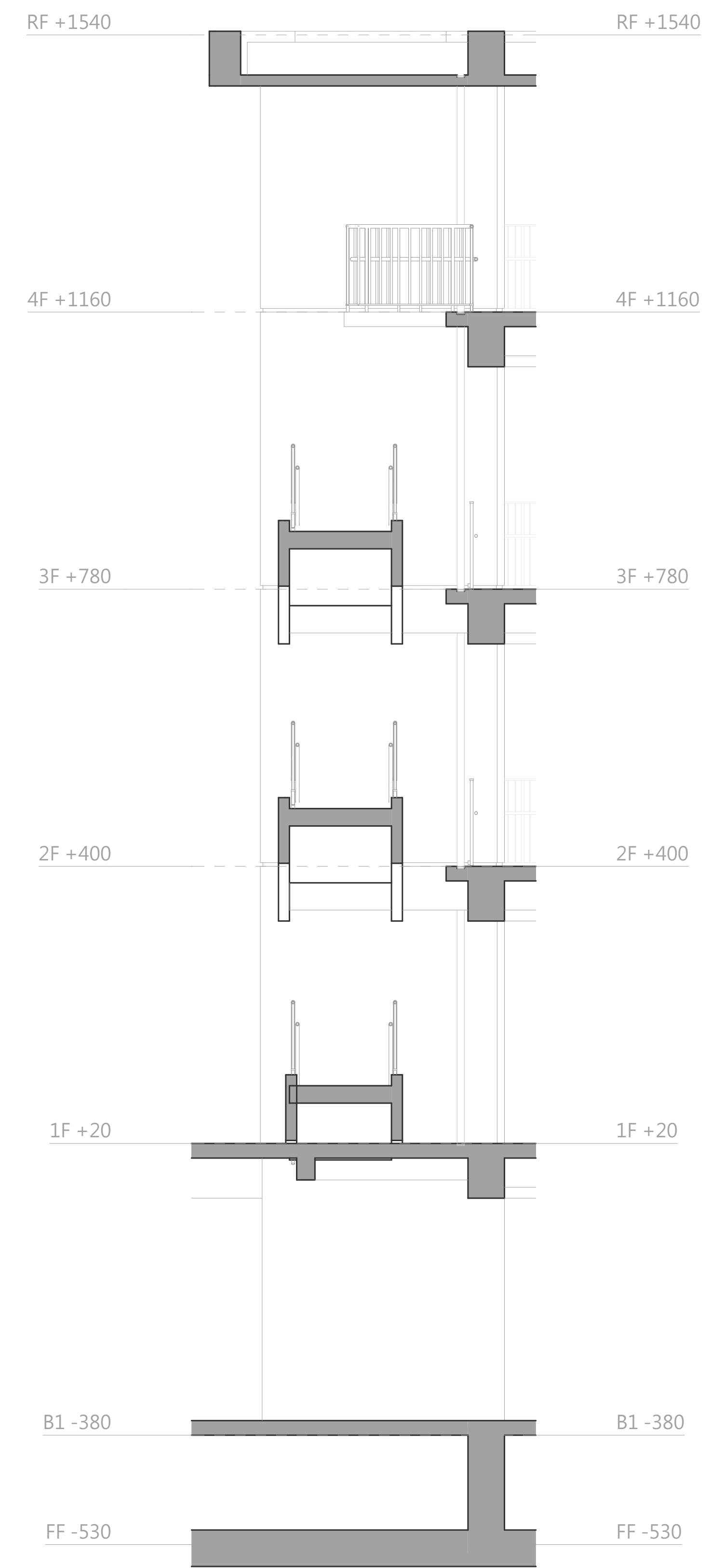
A棟B梯剖面詳圖b A1SCALE=1/50 A3SCALE=1/100
