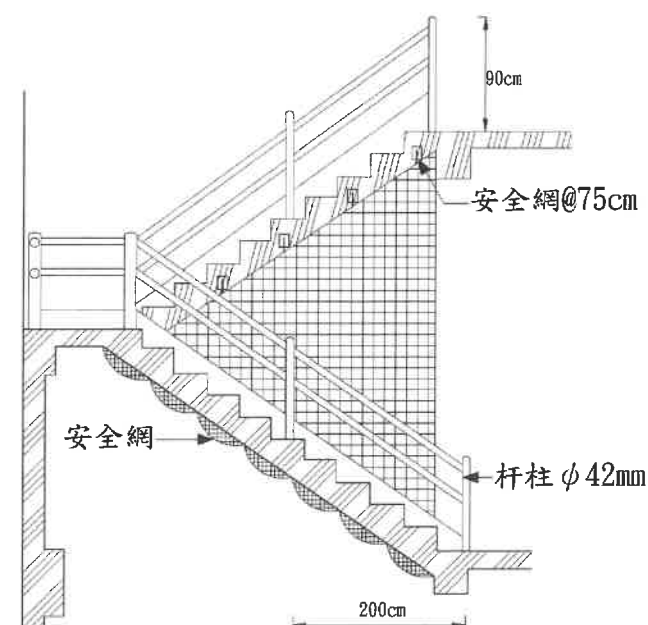
樓梯側立面圖
