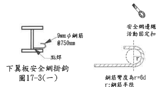
鋼樑吊掛前，下翼版預先焊接安全網掛勾示意圖
