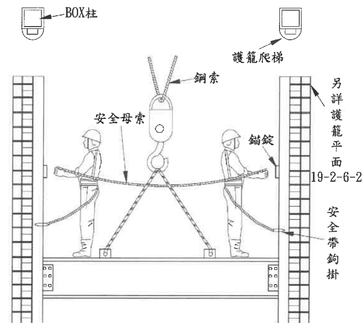
安全母索安裝作業
