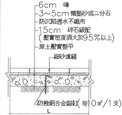
2 北側活動廣場施工剖面圖 SCALE: 1:15(A1); 1:30(A3)
