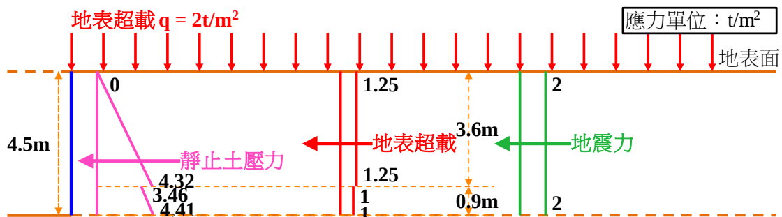
圖 6-2(b) 長期側向土壓力示意
