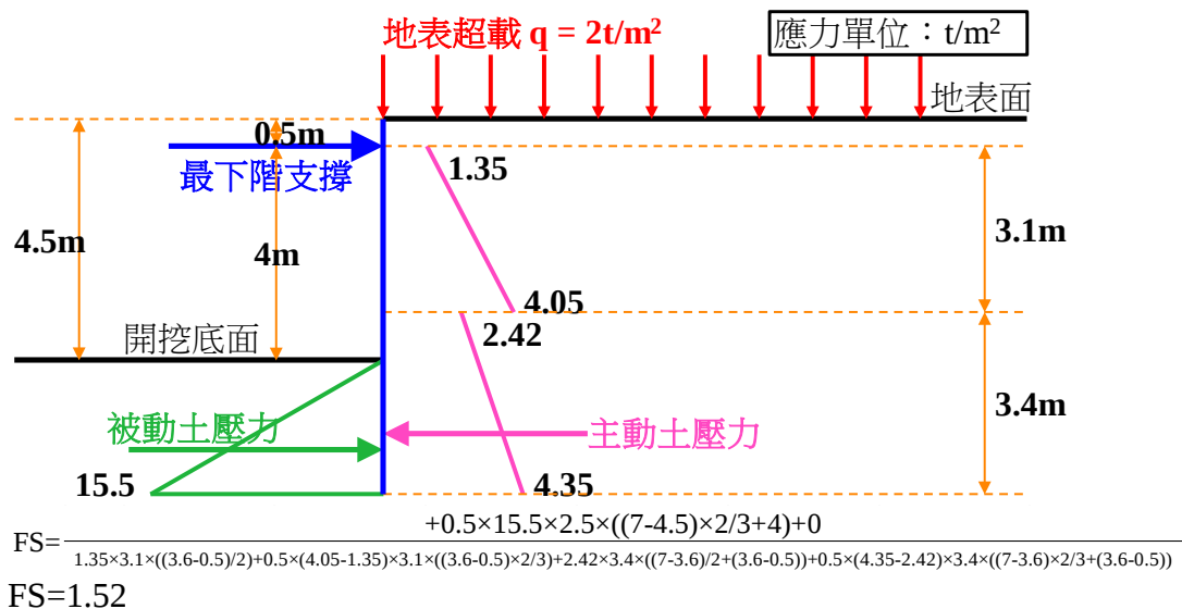
圖 6-1(a) 貫入深度分析示意
