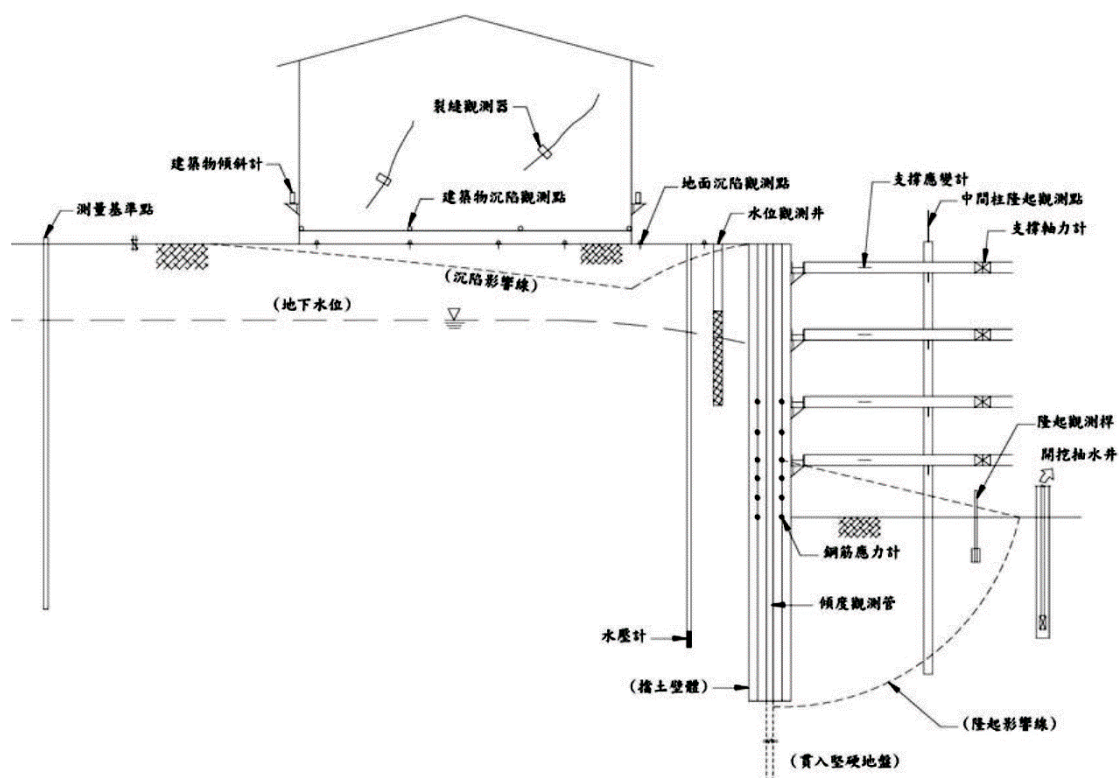
圖 6-3 開挖安全監測系統配置示意圖 (台北市土木技師公會，實用開挖擋土支撐工程設計手冊，2002)
