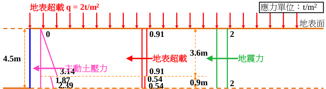
圖 6-2(a) 短期側向土壓力示意
