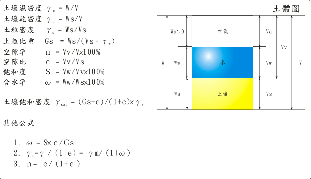
圖 3-5 土體圖及相關應用公式
