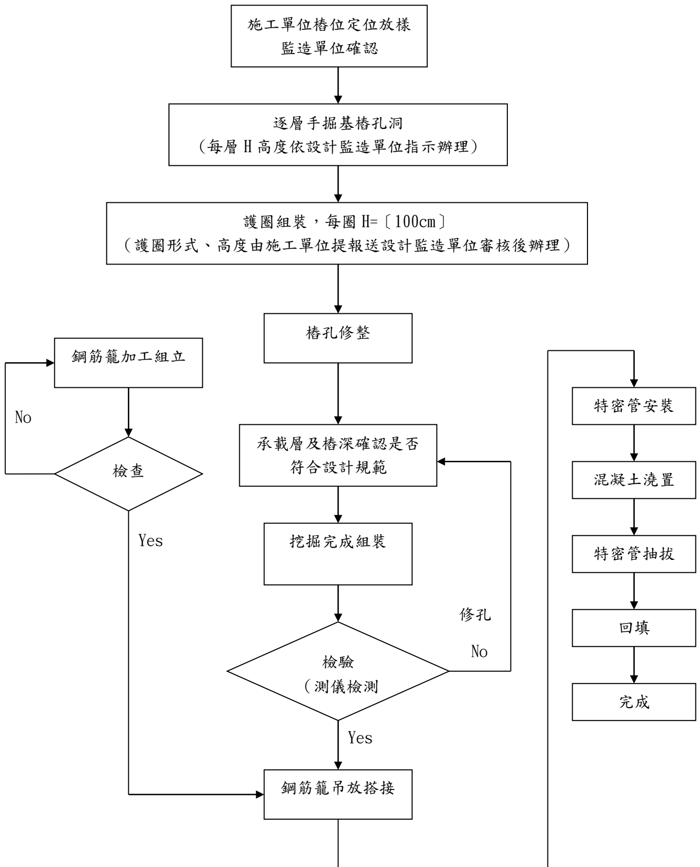
手掘式基樁施工流程圖
