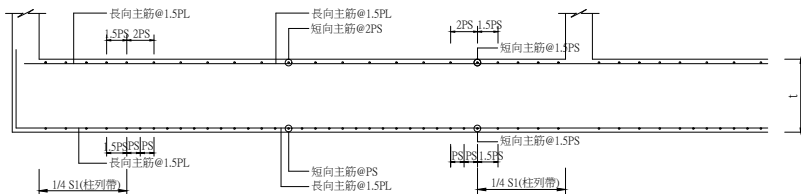
長向柱列帶剖面圖 ㉙ - ㉙
