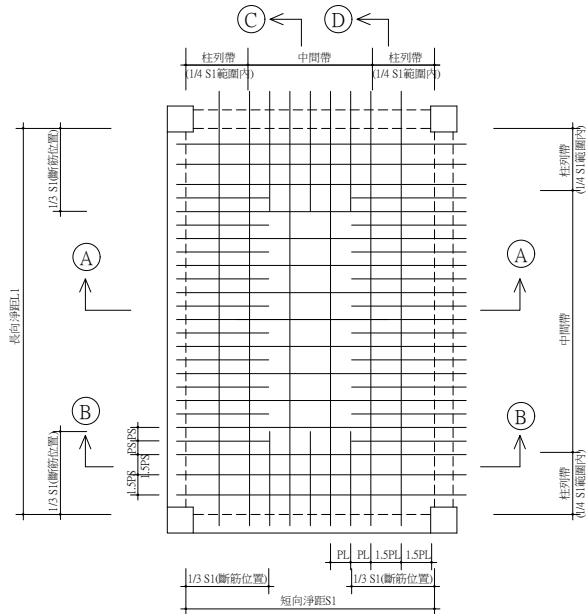
基礎版下層筋平面配置示意圖
