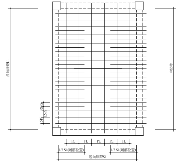
基礎版下層筋平面配置示意圖
