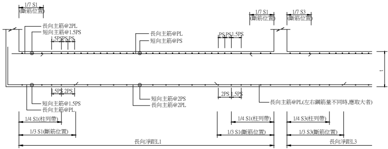
長向中間帶剖面圖 ㉘ - ㉘
