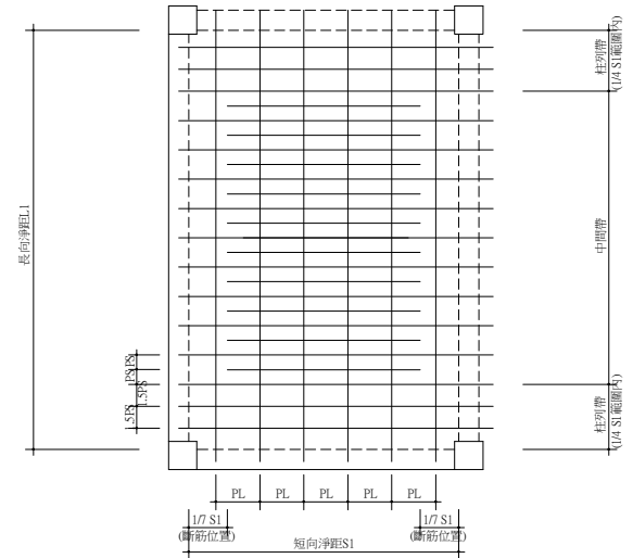
TYPE B:基礎版配筋平面圖及剖面圖—短向斷筋 長向直通式
