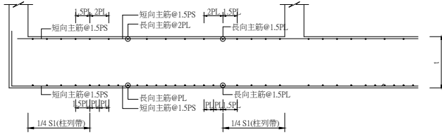
短向柱列帶剖面圖 ㉗ - ㉗
