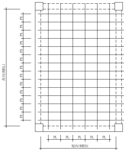
版平面配置示意圖
