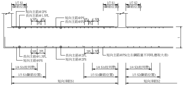
短向中間帶剖面圖 ㉖ - ㉖
