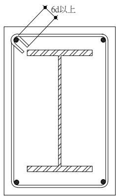
(a)135°彎鉤閉合形
