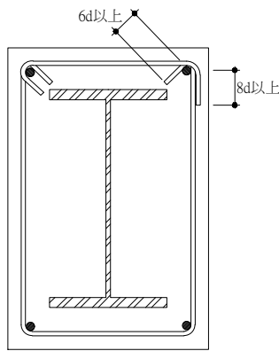
(b)兩端135°彎鉤U形加 90°與135°彎鉤門形
