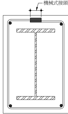
(d)機械式接頭閉合形
