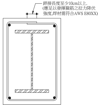
(c)搭接銲接方式(需採可焊 型鋼筋)
