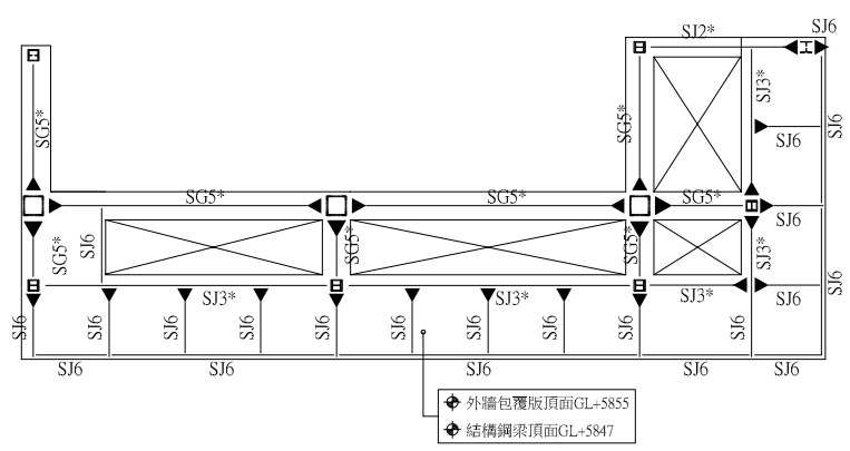
註：1.本圖梁位不可直接用於放樣及相關施工圖說，承商須依據建築圖說幾何關係並參考結構配置原則檢討及繪製相關圖面，經審查核可後方可施工。 2.本層設計活載重為500kgf/m 2 。 3."——"為大樑側撐，詳見圖S0-14
